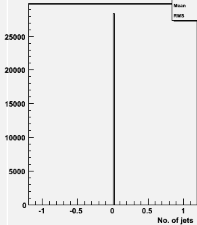
No. jets (ycut=0.001) : w102825 e1a_e1n2n2_o
