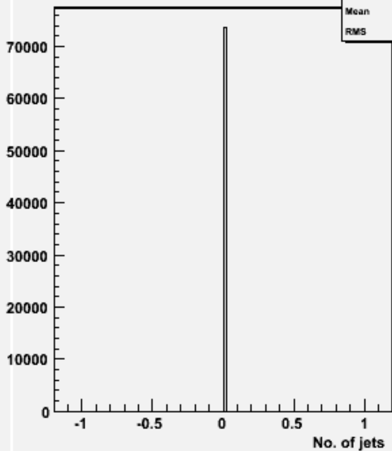
No. jets (ycut=0.001) : w102824 e1a_e1n2n2_o
