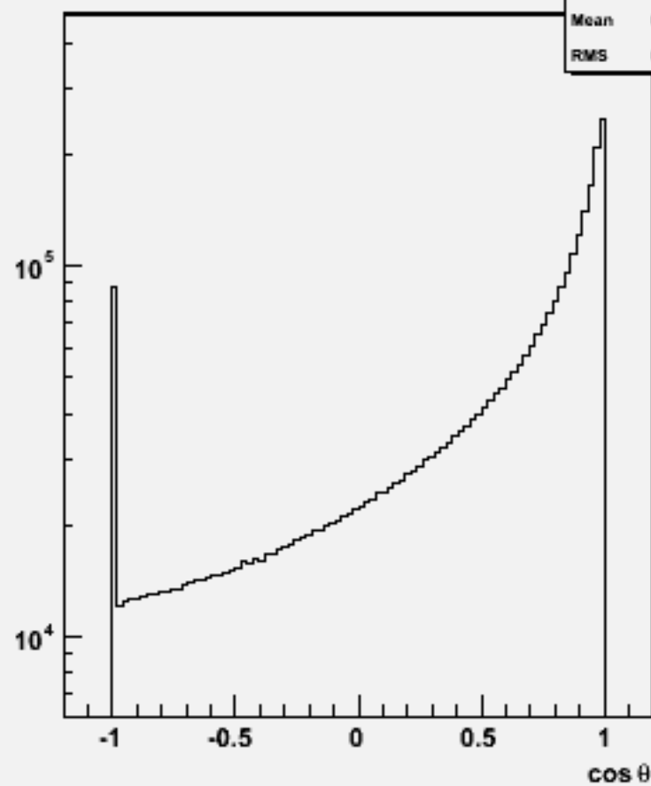
Particle cos \theta : w102821 e1a_n1sc_o
