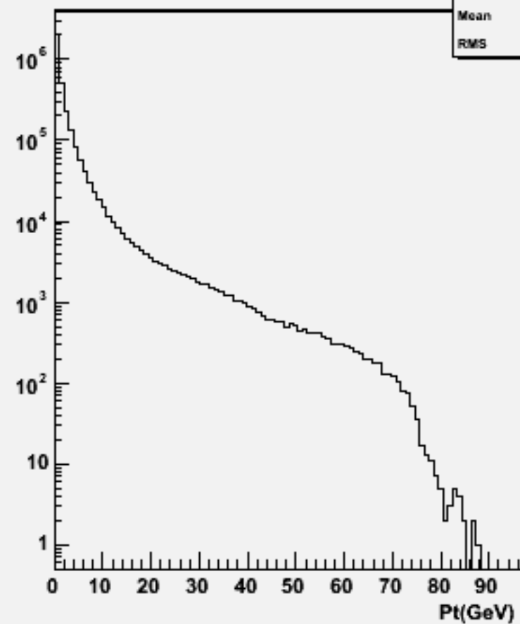
Particle Pt : w102821 e1a_n1sc_o
