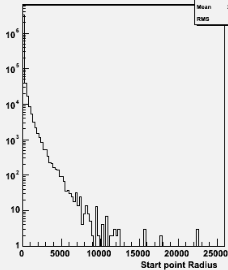
Start point R : w102821 e1a_n1sc_o
