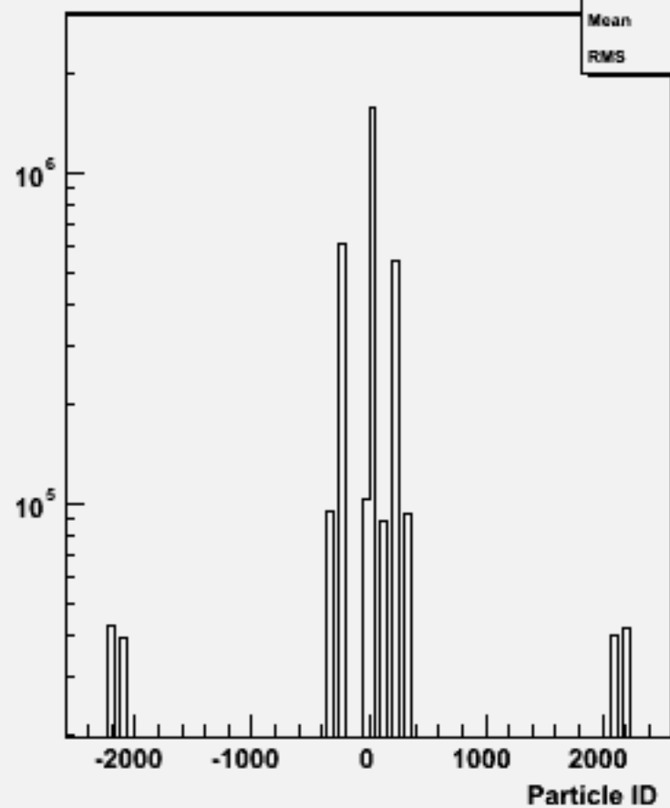
Particle ID : w102821 e1a_n1sc_o
