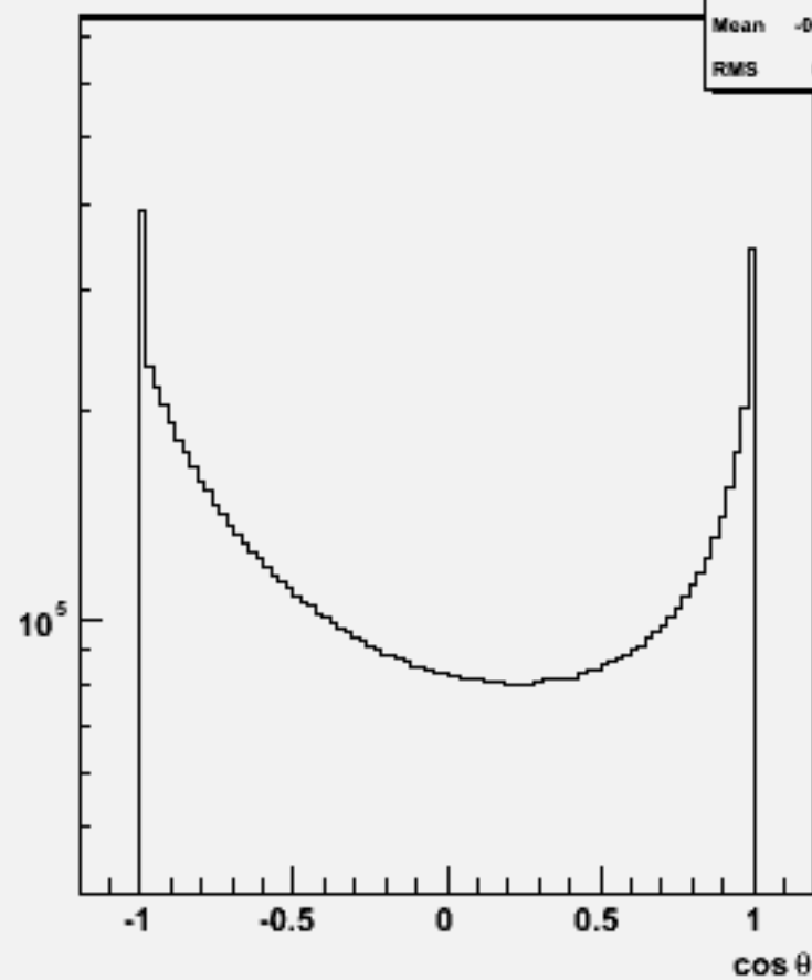
Particle cos \theta : w102820 e1a_n1sc_o
