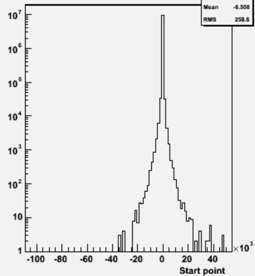
Start point Z : w102820 e1a_n1sc_o
