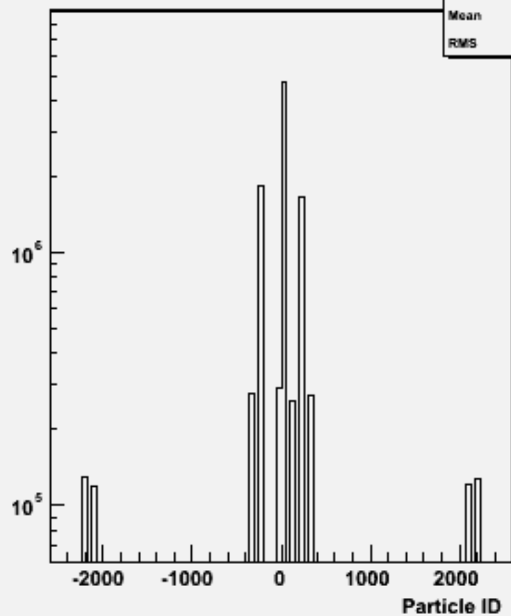
Particle ID : w102820 e1a_n1sc_o
