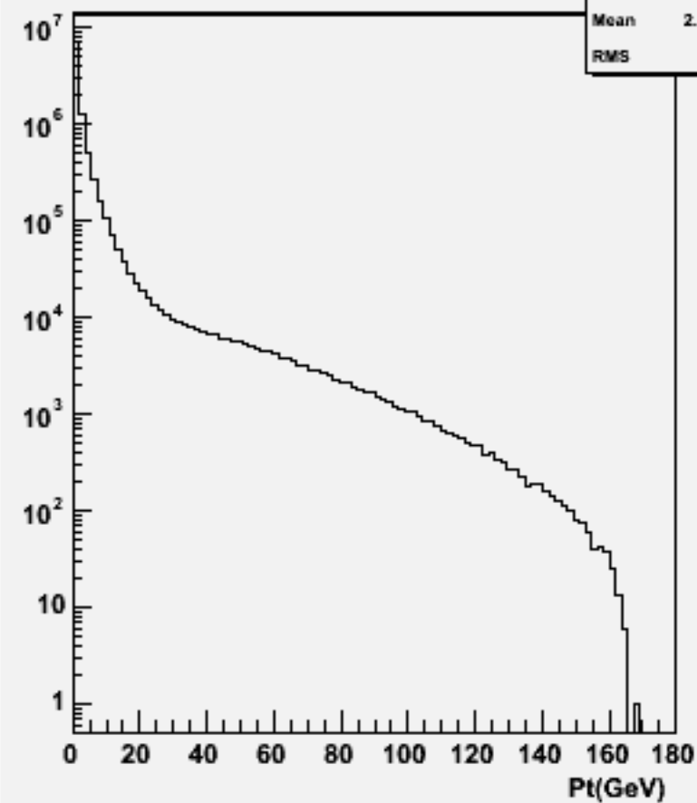
Particle Pt : w102820 e1a_n1sc_o
