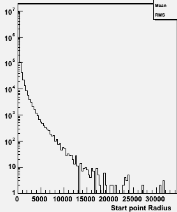
Start point R : w102820 e1a_n1sc_o
