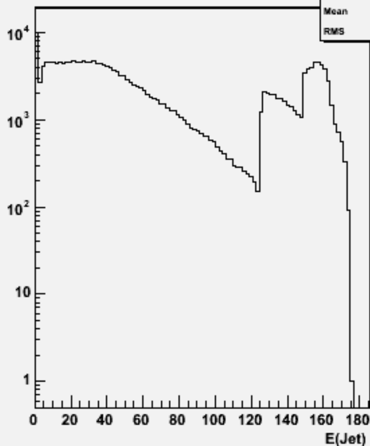
Jet energies(All jets)w102817 e1a_n1du_o
