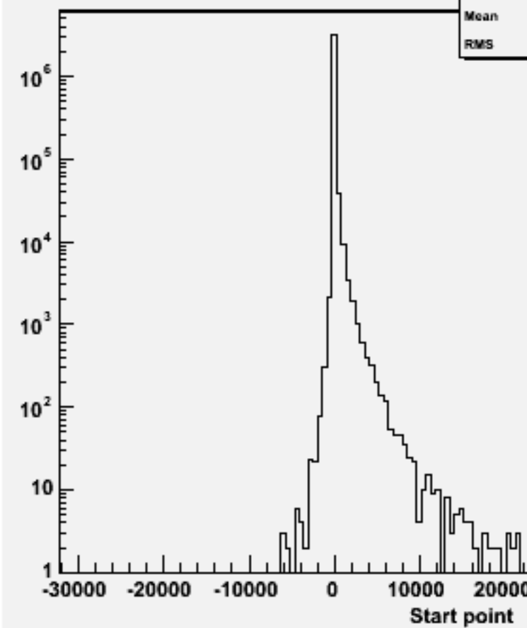
Start point Z : w102817 e1a_n1du_o
