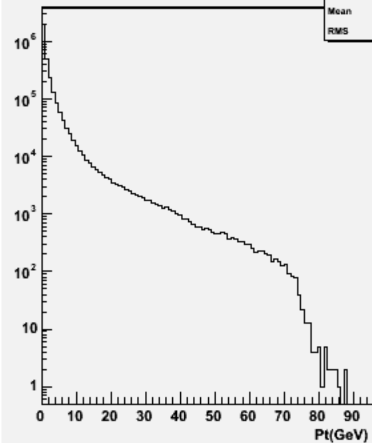
Particle Pt : w102817 e1a_n1du_o
