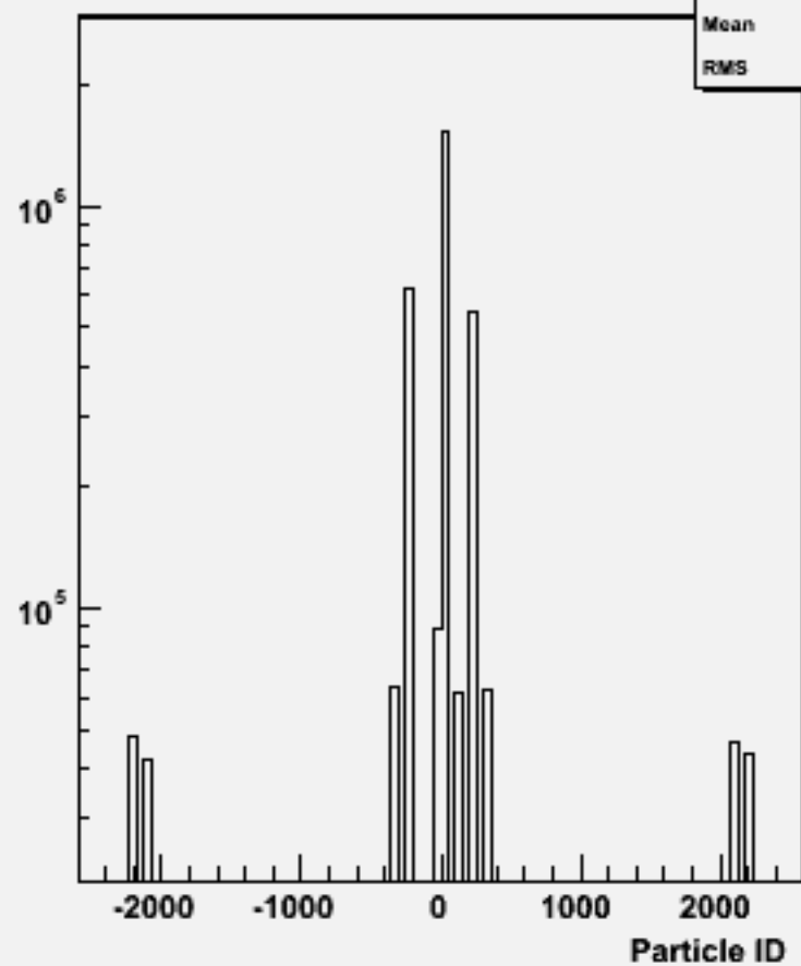
Particle ID : w102817 e1a_n1du_o
