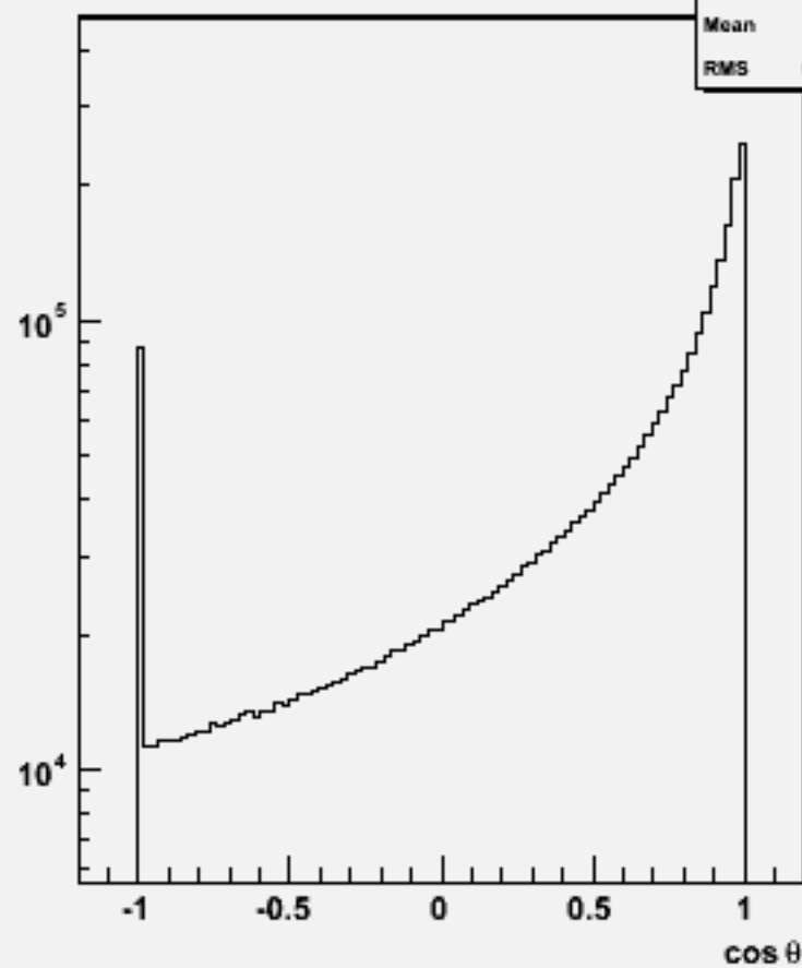
Particle cos \theta : w102817 e1a_n1du_o
