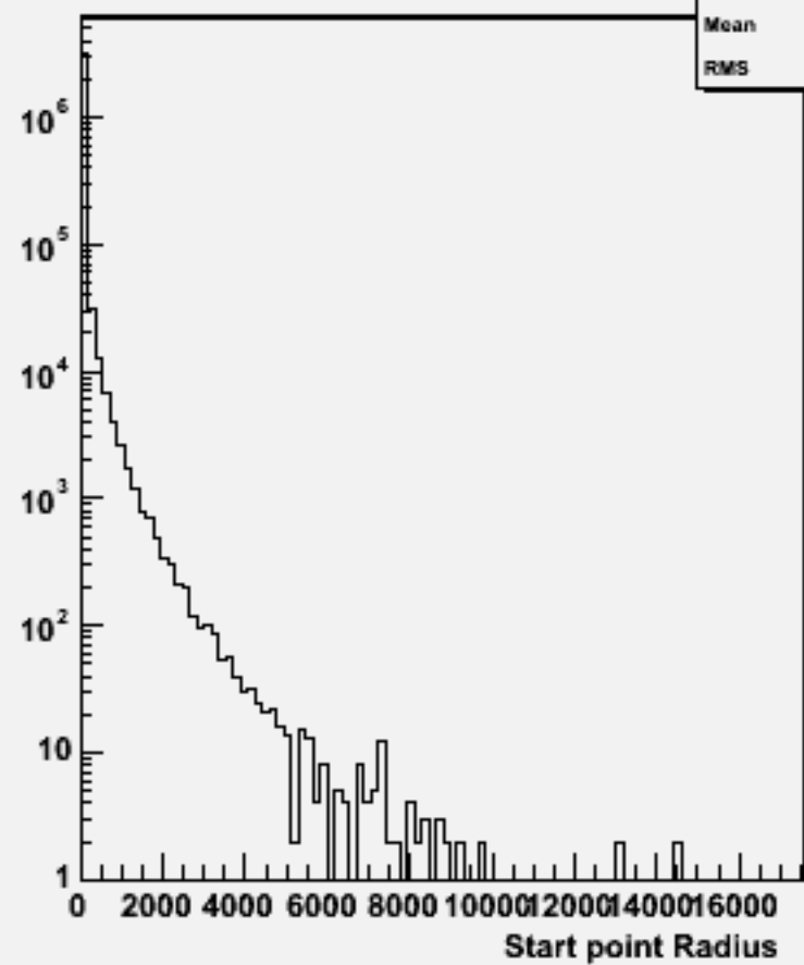
Start point R : w102817 e1a_n1du_o
