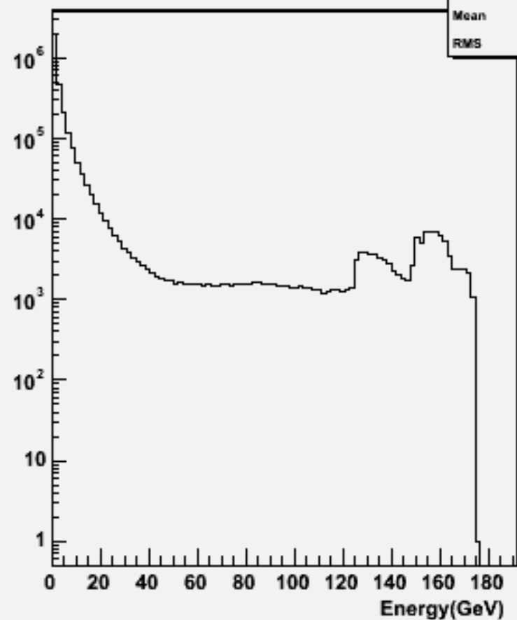
Particle Energy : w102817 e1a_n1du_o
