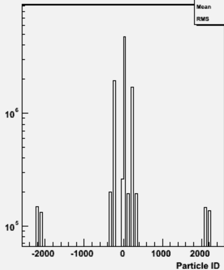
Particle ID : w102816 e1a_n1du_o
