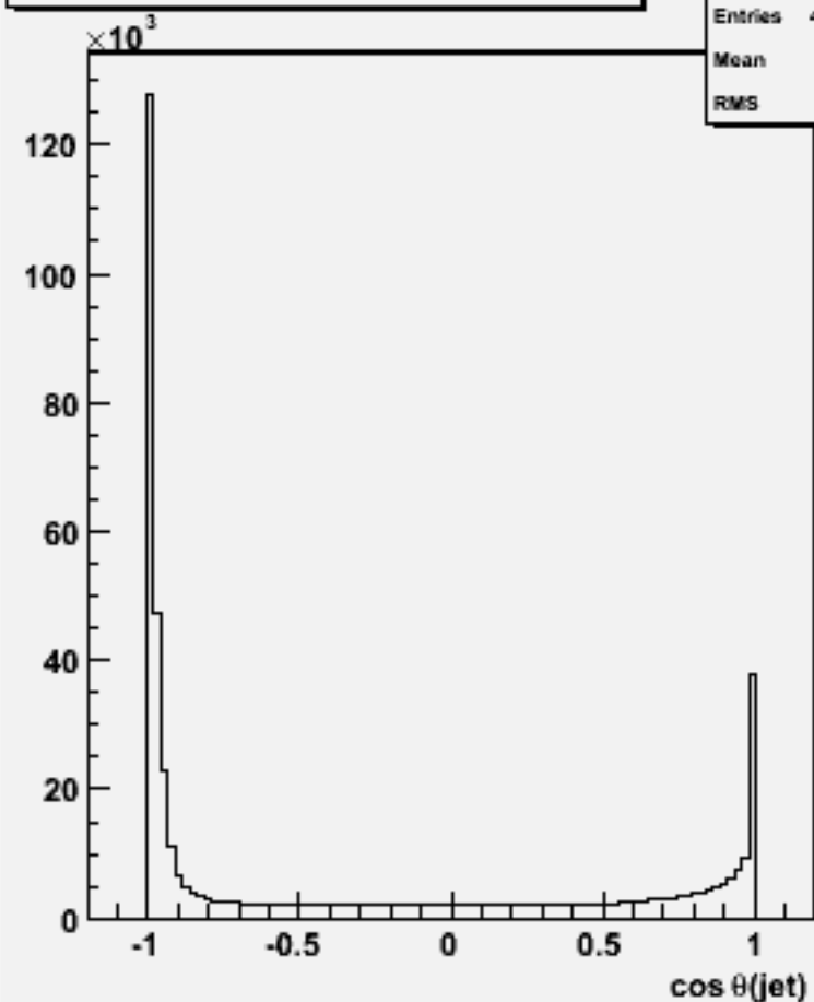
cos \theta for 2-jets :w102816 e1a_n1du_o
