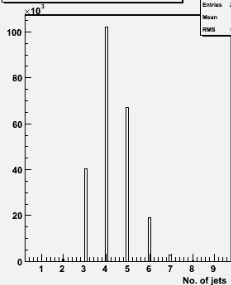
No. jets (ycut=0.001) : w102816 e1a_n1du_o
