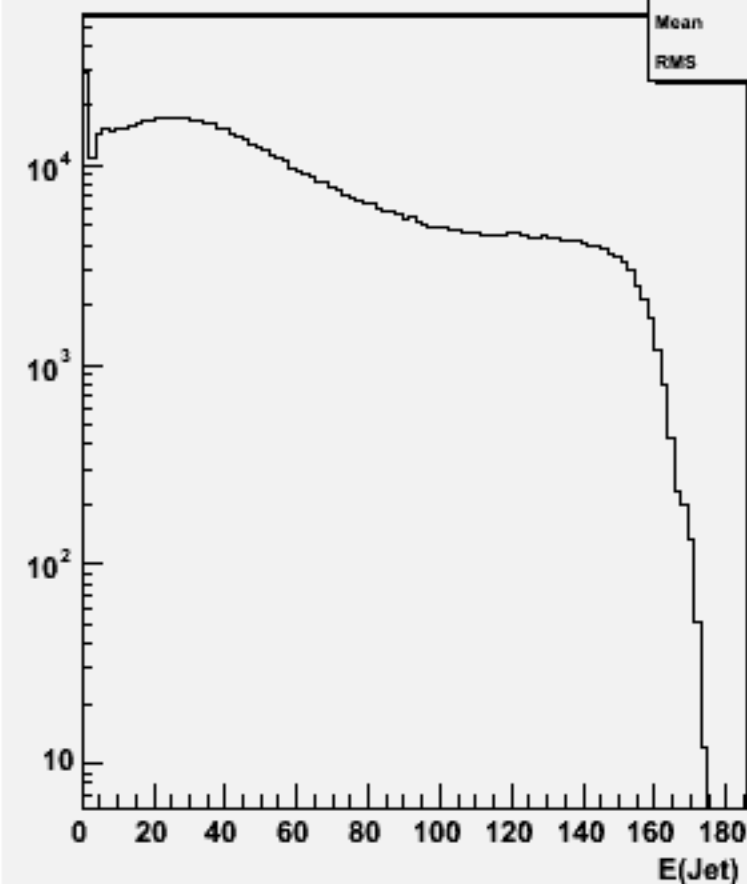
Jet energies(All jets)w102816 e1a_n1du_o
