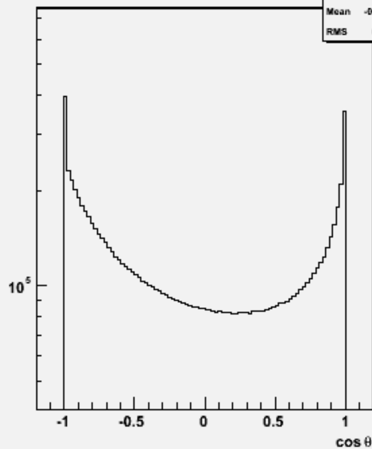
Particle cos \theta : w102816 e1a_n1du_o
