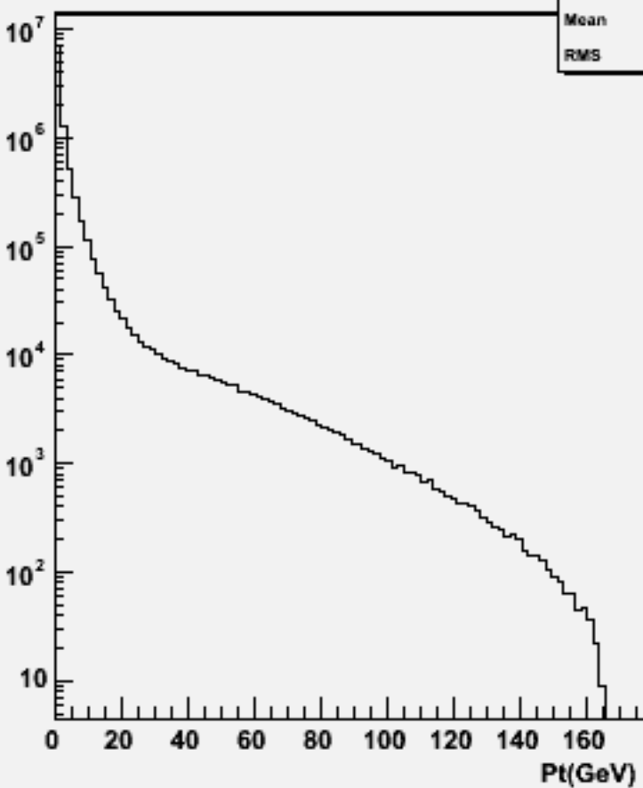
Particle Pt : w102816 e1a_n1du_o
