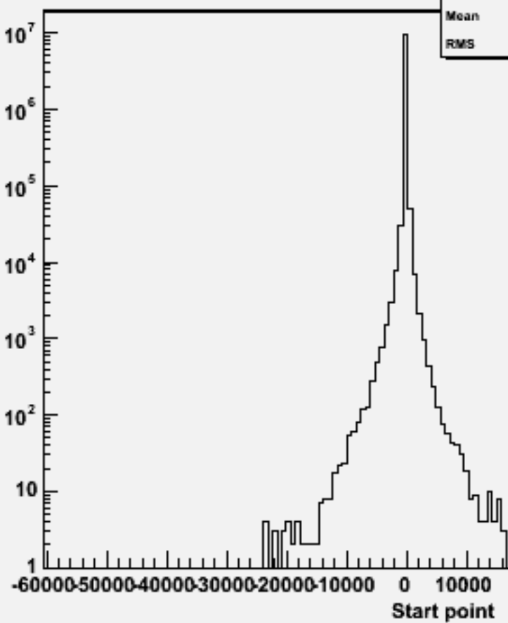
Start point Z : w102816 e1a_n1du_o
