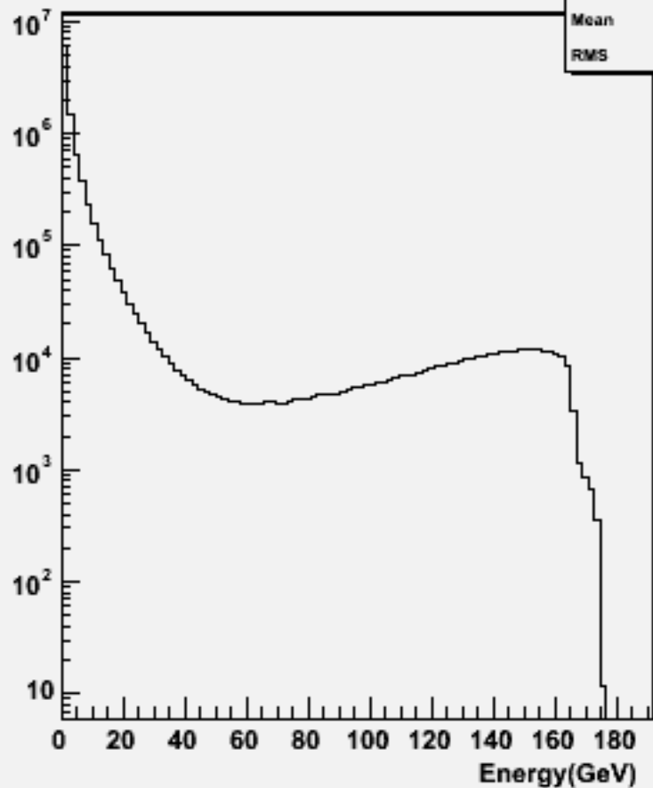
Particle Energy : w102816 e1a_n1du_o
