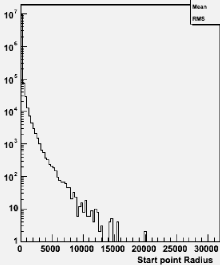
Start point R : w102816 e1a_n1du_o
