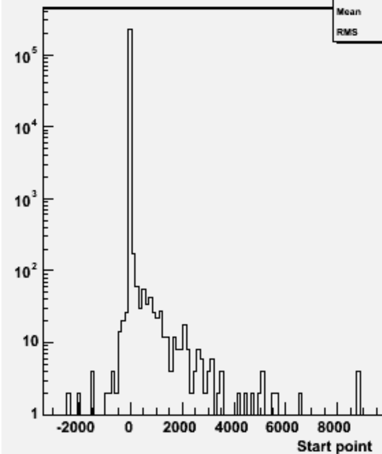
Start point Z : w102813 e1a_n1e3n3_o
