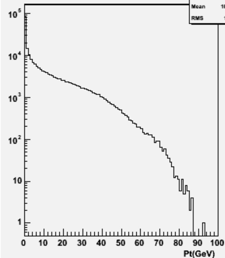
Particle Pt : w102813 e1a_n1e3n3_o
