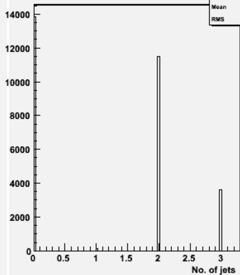
No. jets (ycut=0.001) : w102813 e1a_n1e3n3_o
