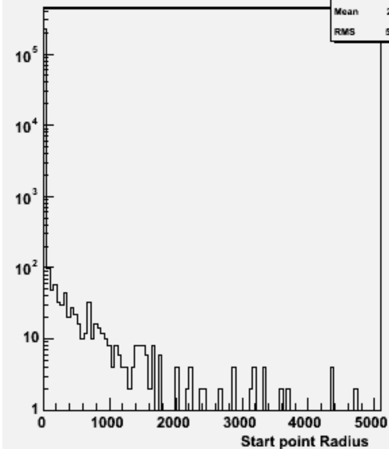
Start point R : w102813 e1a_n1e3n3_o
