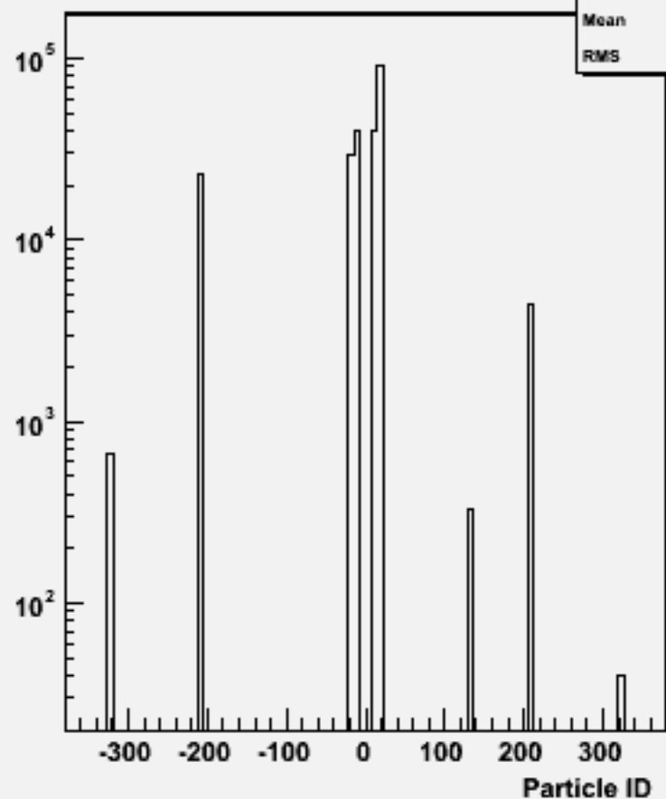
Particle ID : w102813 e1a_n1e3n3_o
