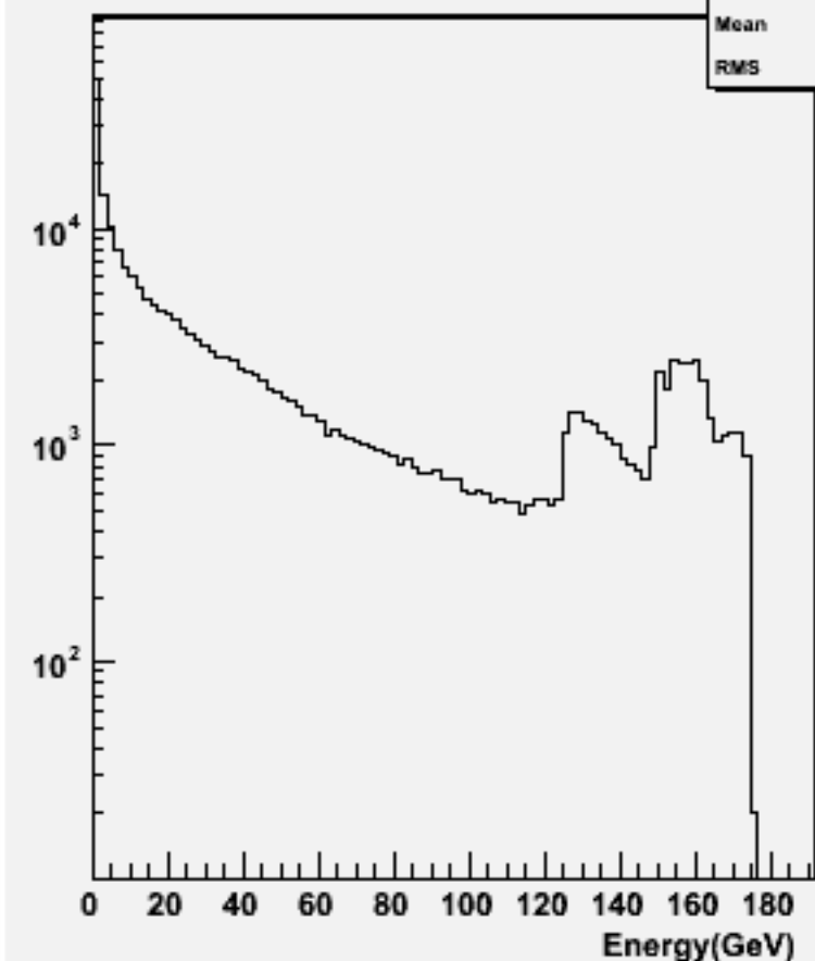
Particle Energy : w102813 e1a_n1e3n3_o
