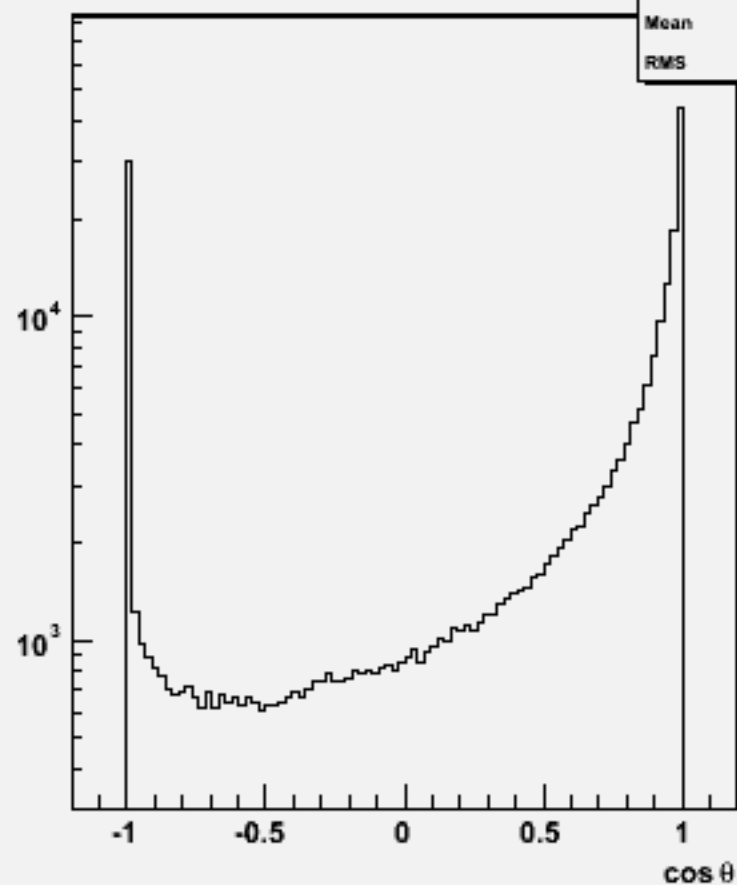
Particle \cos\theta : w102813 e1a_n1e3n3_o
