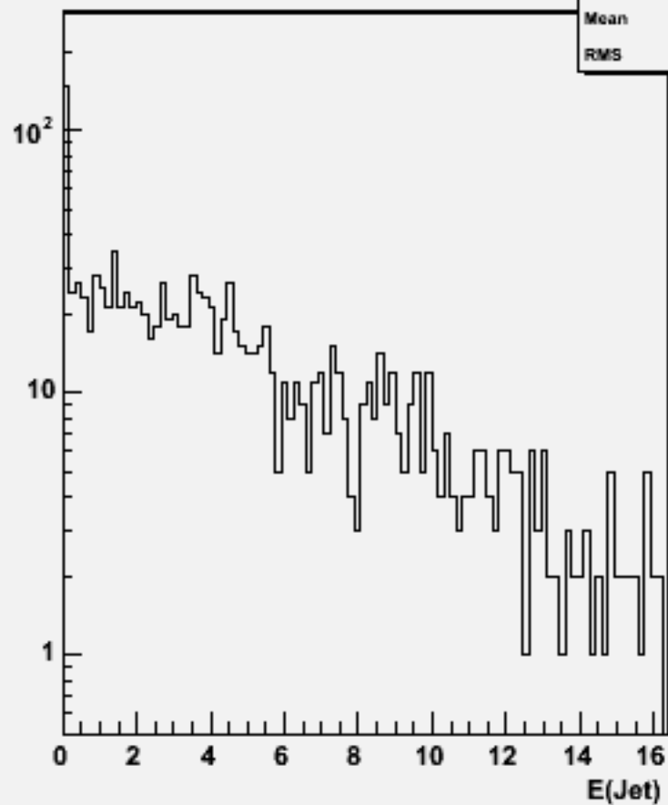
Jet energies(All jets)w102812 e1a_n1e3n3_o
