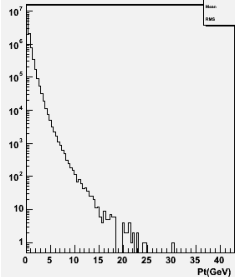
Particle Pt : w102802 aa_bb_o
