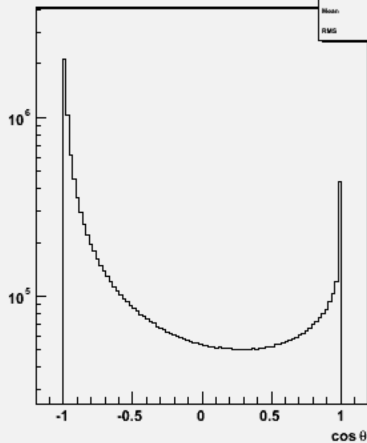
Particle cos \theta : w102802 aa_bb_o
