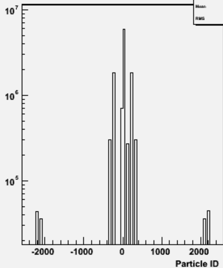
Particle ID : w102802 aa_bb_o
