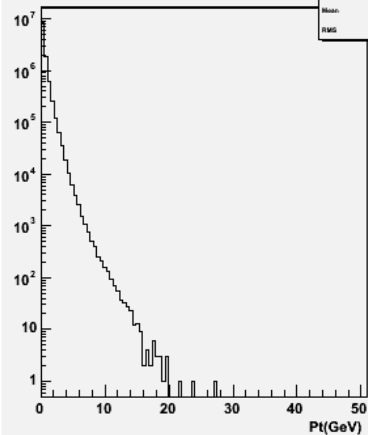
Particle Pt : w102801 aa_bb_o
