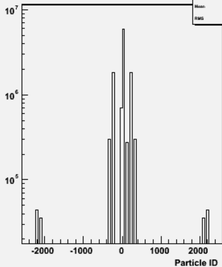
Particle ID : w102801 aa_bb_o
