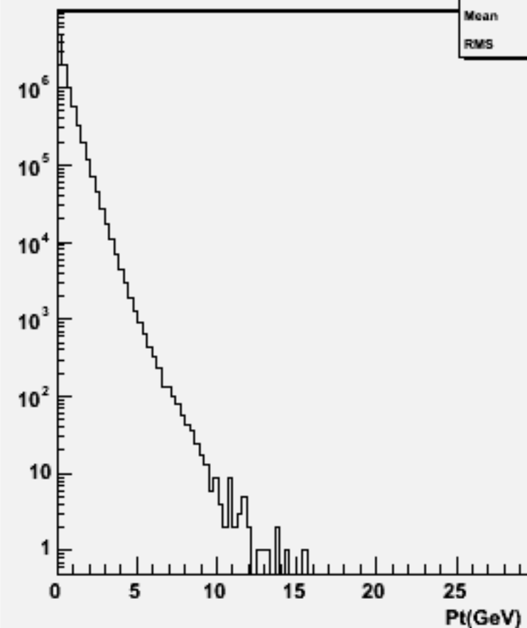
Particle Pt : w102799 aa_cc_o
