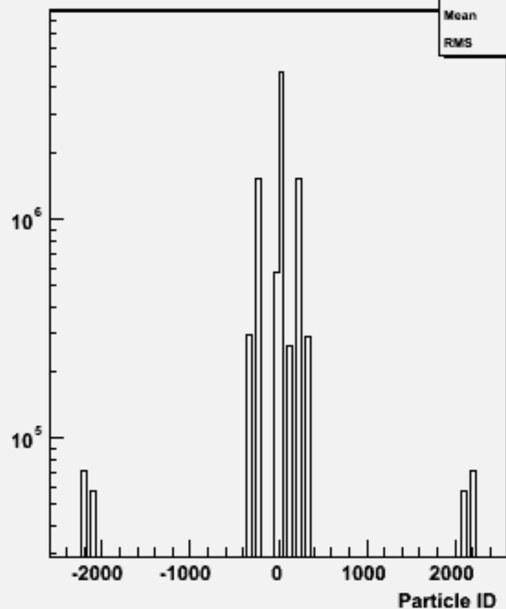
Particle ID : w102799 aa_cc_o
