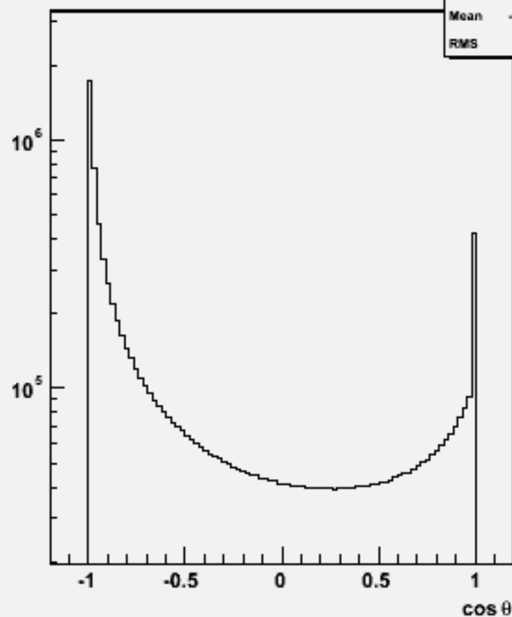
Particle \cos\theta : w102798 aa_cc_o
