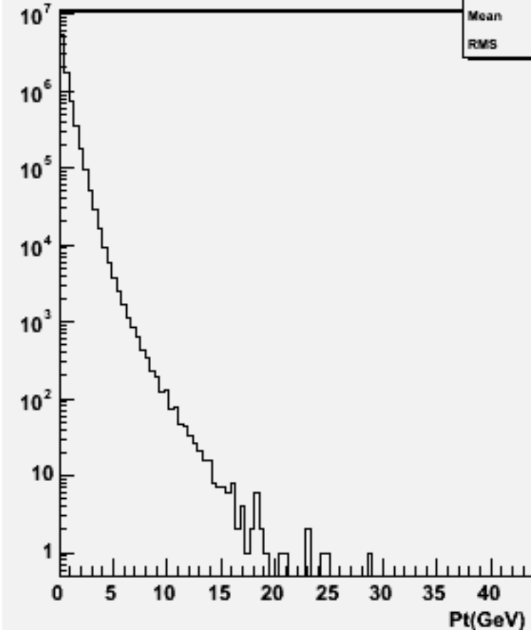
Particle Pt : w102798 aa_cc_o
