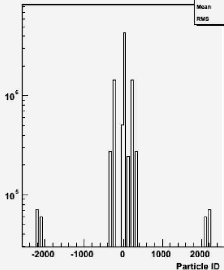
Particle ID : w102798 aa_cc_o
