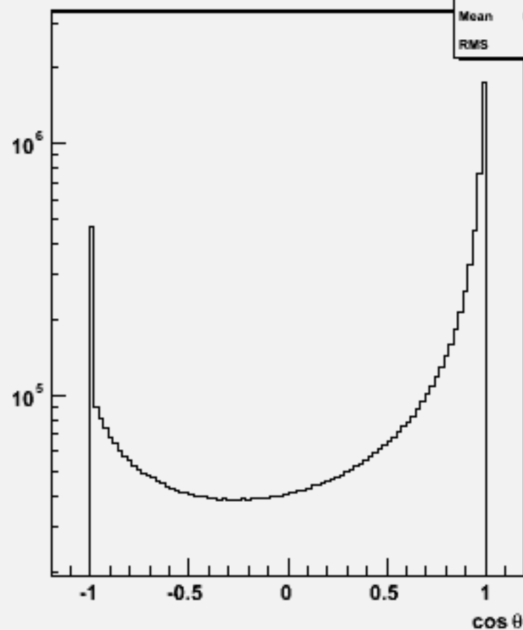
Particle cosθ : w102789 aa_dd_o
