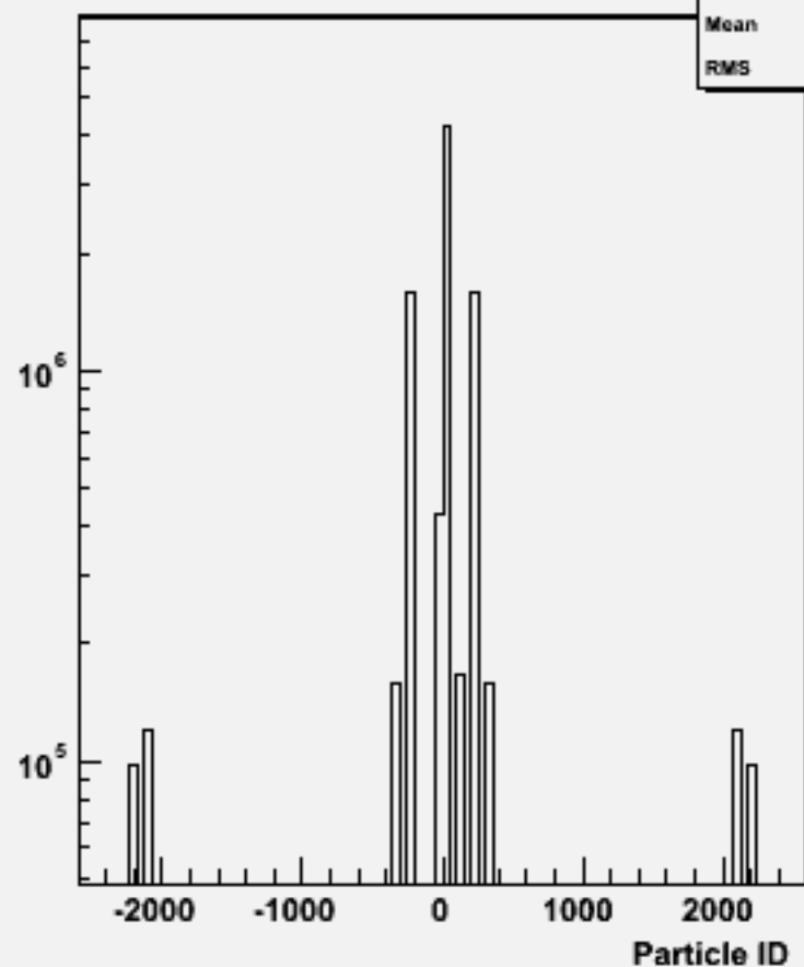
Particle ID : w102789 aa_dd_o
