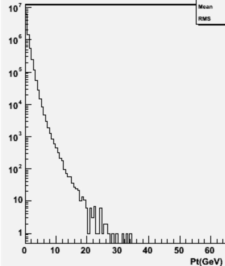
Particle Pt : w102789 aa_dd_o
