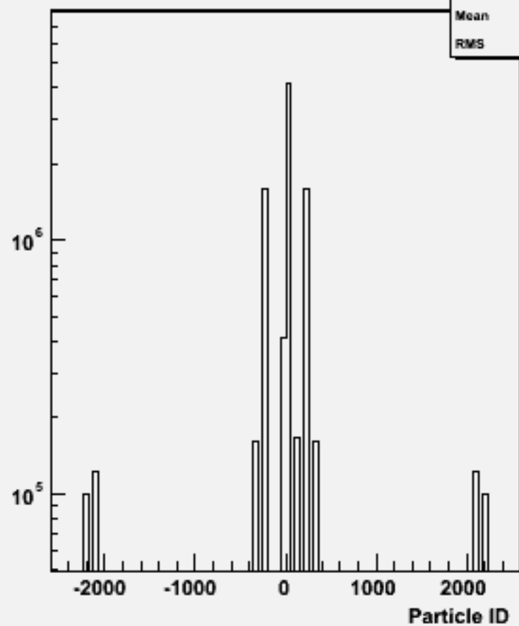
Particle ID : w102788 aa_dd_o
