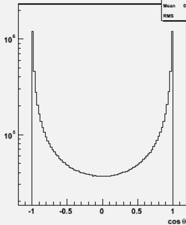
Particle cos \theta : w102788 aa_dd_o
