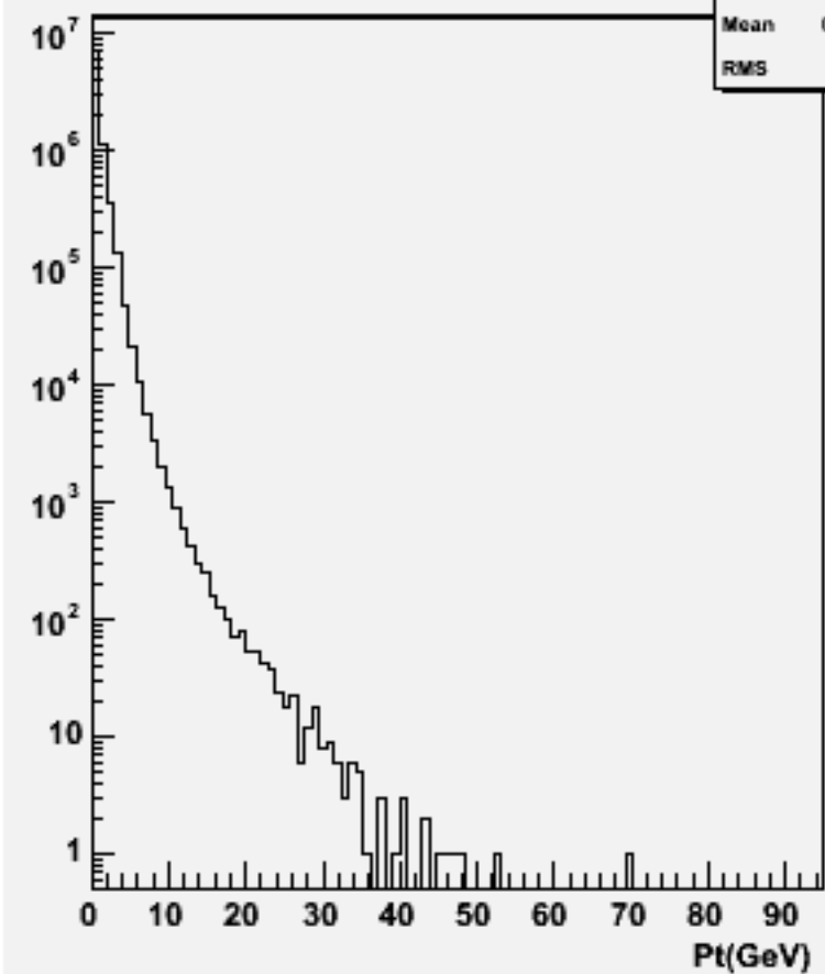
Particle Pt : w102788 aa_dd_o
