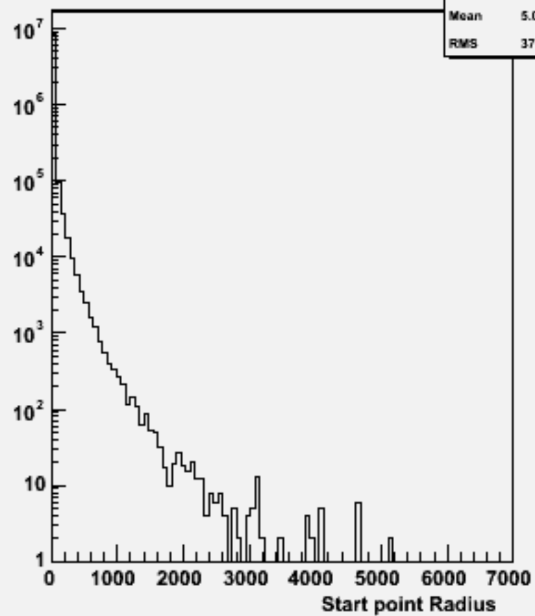
Start point R : w102788 aa_dd_o
