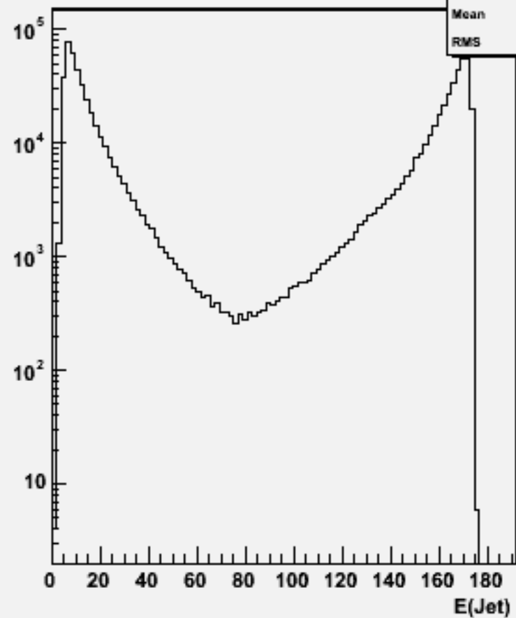
Jet energies(All jets)w102785 aa_uu_o
