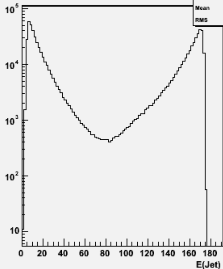
Jet energies(All jets)w102784 aa_uu_o
