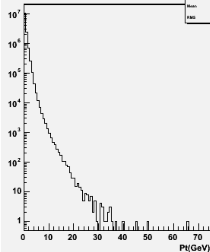
Particle Pt : w102781 aa_e3e3_o
