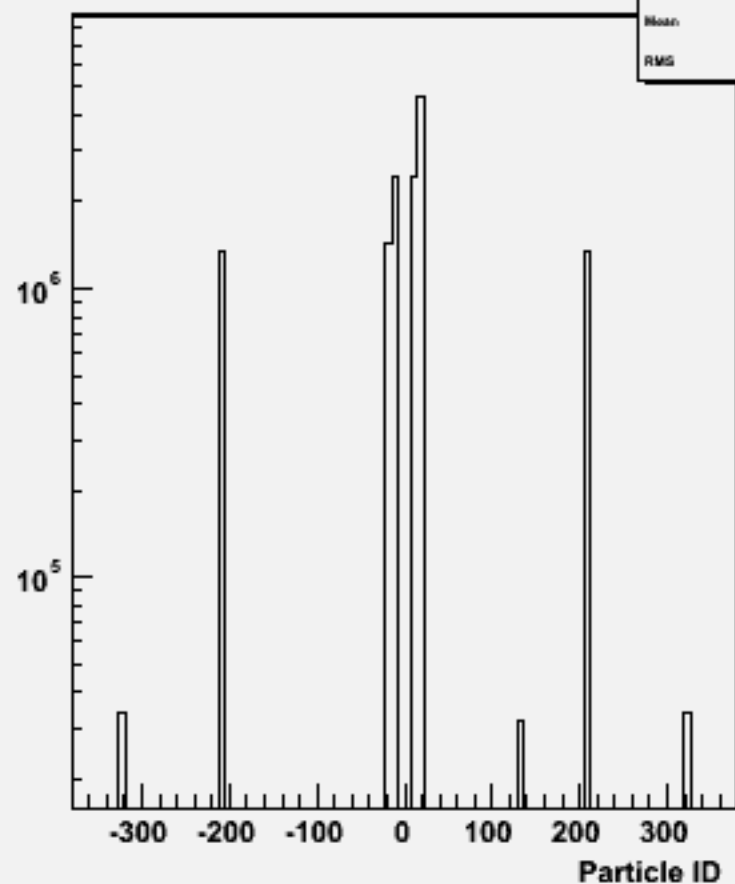
Particle ID : w102781 aa_e3e3_o
