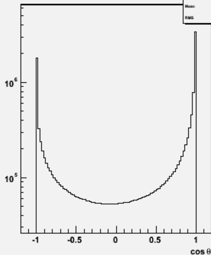
Particle cos \theta : w102781 aa_e3e3_o
