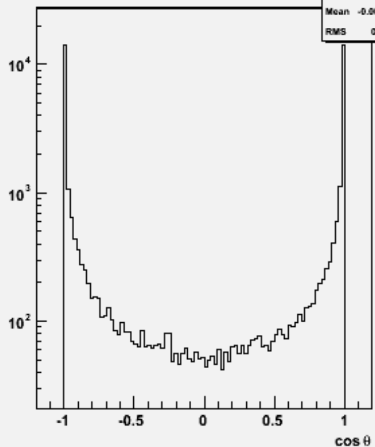
Particle cos \theta : w102779 aa_e2e2_o
