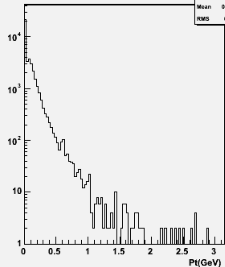
Particle Pt : w102779 aa_e2e2_o
