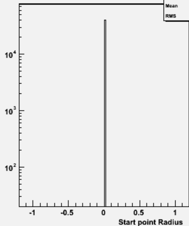
Start point R : w102779 aa_e2e2_o
