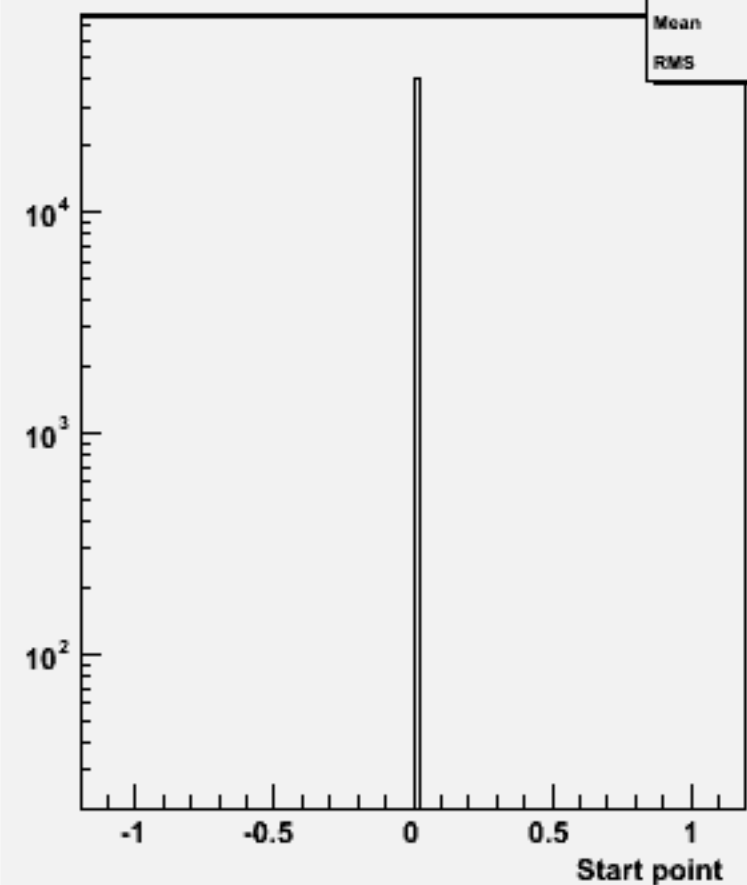
Start point Z : w102779 aa_e2e2_o
