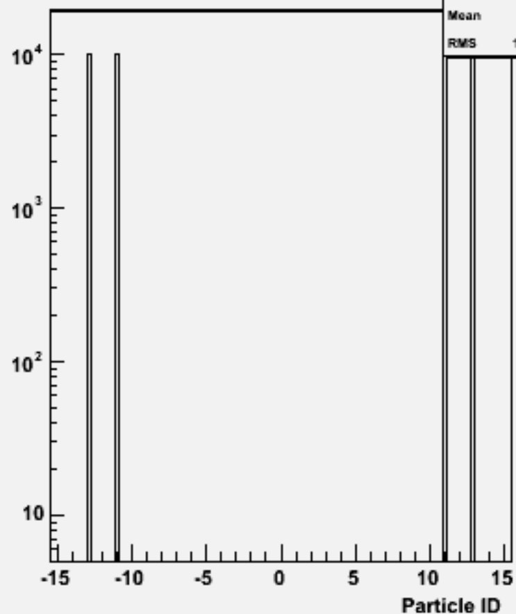
Particle ID : w102779 aa_e2e2_o
