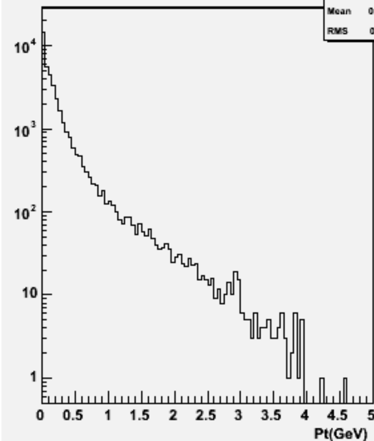
Particle Pt : w102776 aa_e2e2_o
