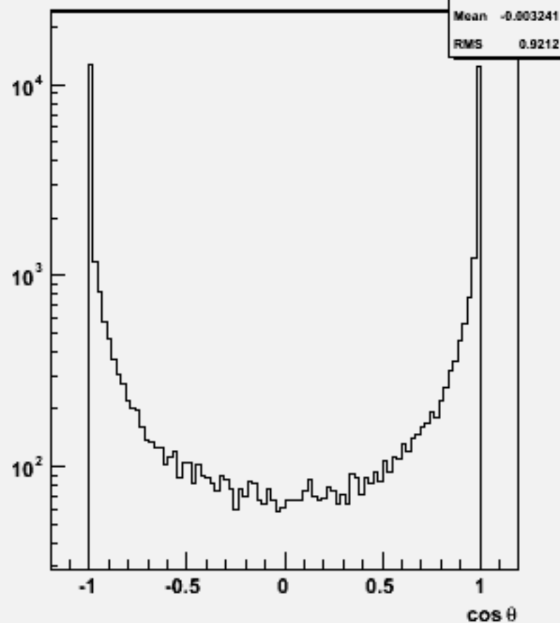
Particle cos \theta : w102776 aa_e2e2_o
