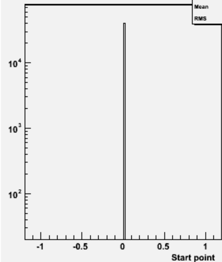
Start point Z : w102776 aa_e2e2_o
