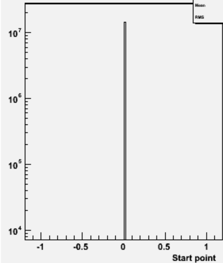
Start point Z : w102775 aa_e1e1_o
