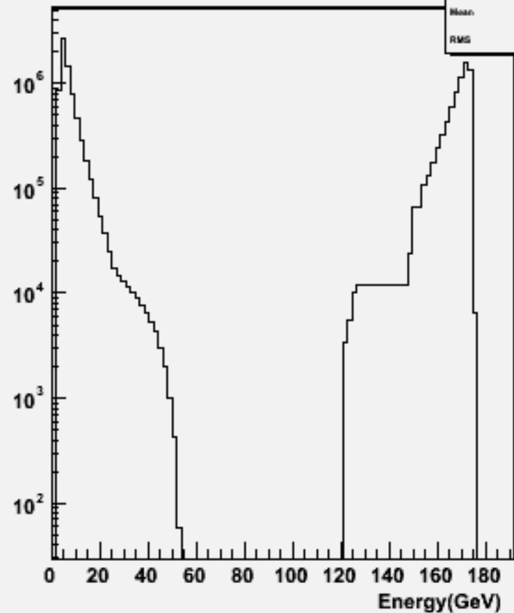
Start point R : w102775 aa_e1e1_o
