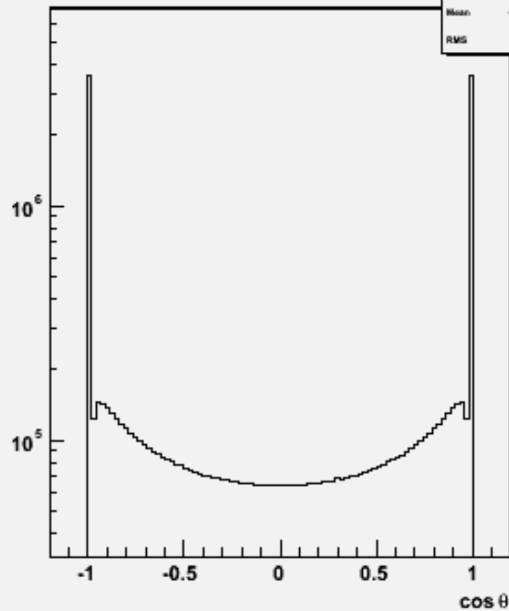
Particle \cos\theta : w102775 aa_e1e1_o
