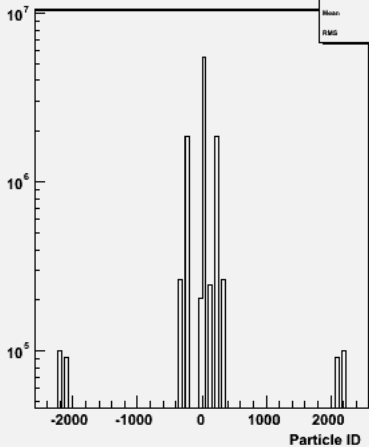
Particle ID : w102770 bb_o
