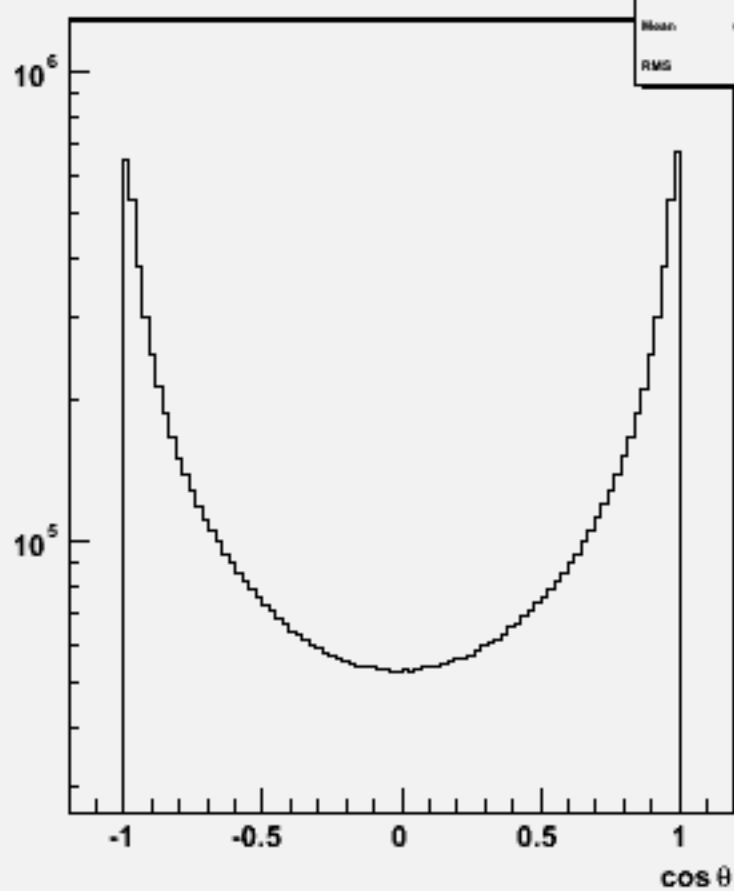
Particle cosθ : w102770 bb_o
