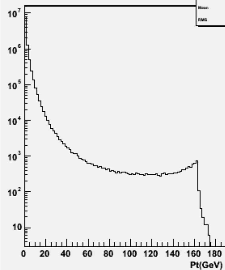
Particle Pt : w102770 bb_o
