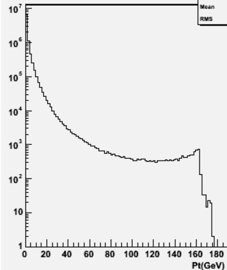
Particle Pt : w102766 ss_o
