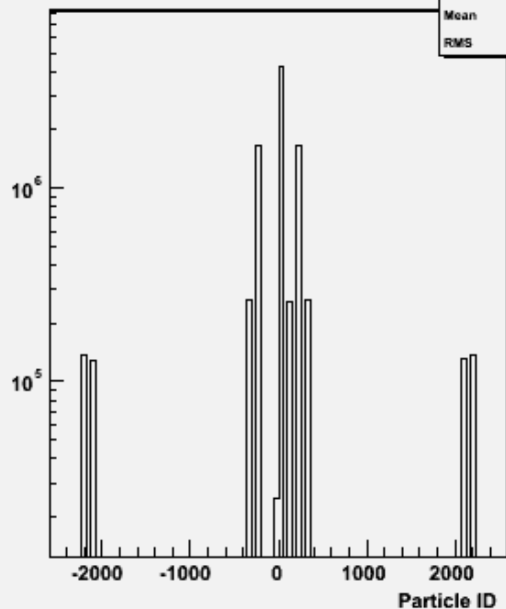
Particle ID : w102766 ss_o
