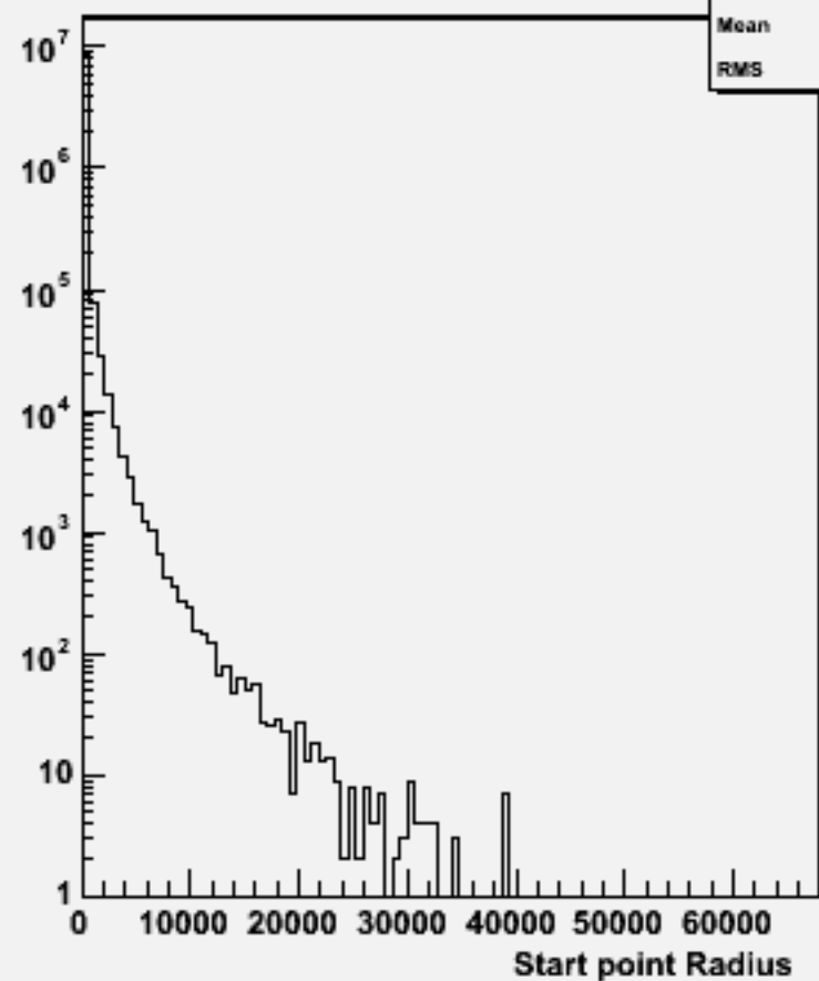
Start point R : w102766 ss_o
