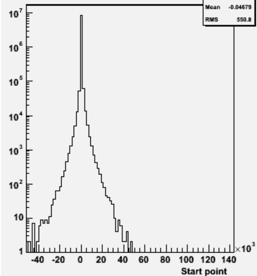
Start point Z : w102766 ss_o
