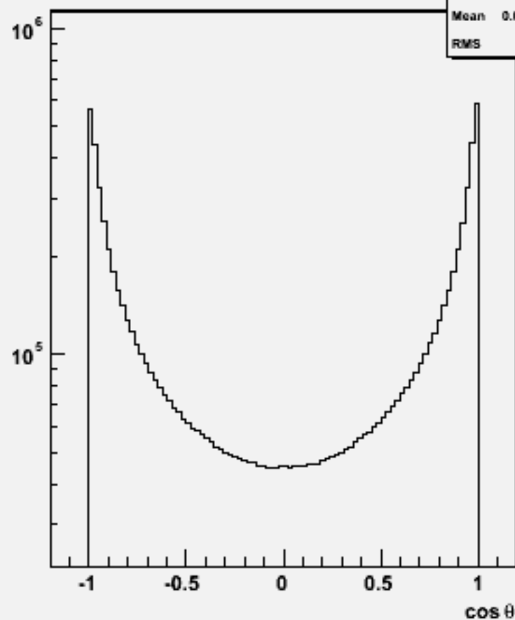
Particle cosθ : w102766 ss_o
