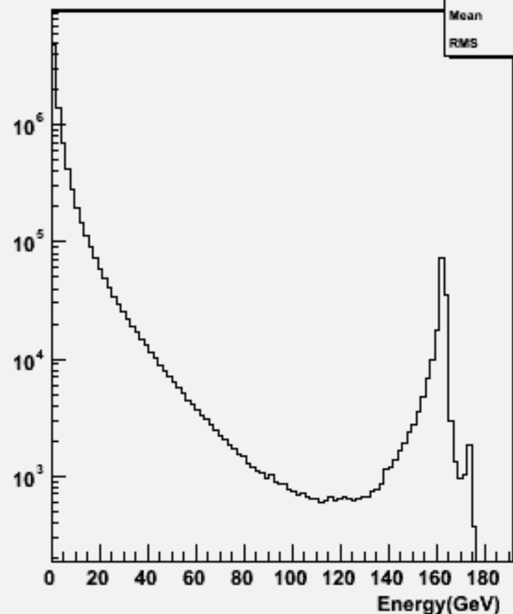
Particle Energy : w102766 ss_o
