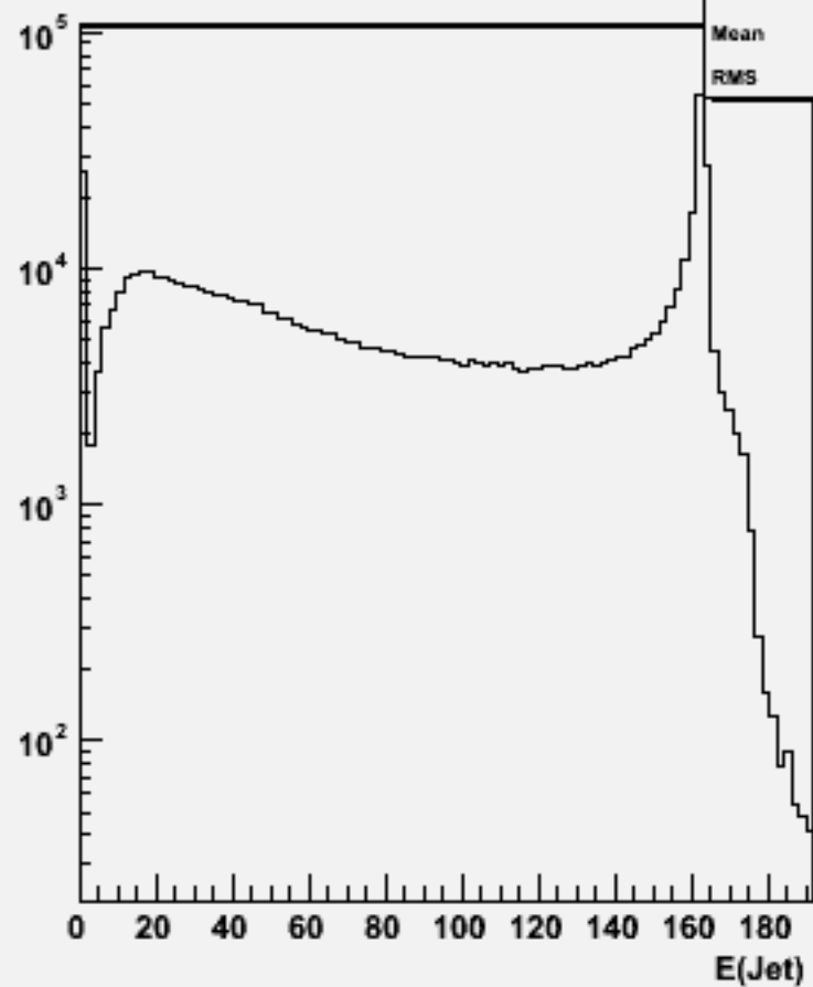
Jet energies(All jets)w102762 dd_o
