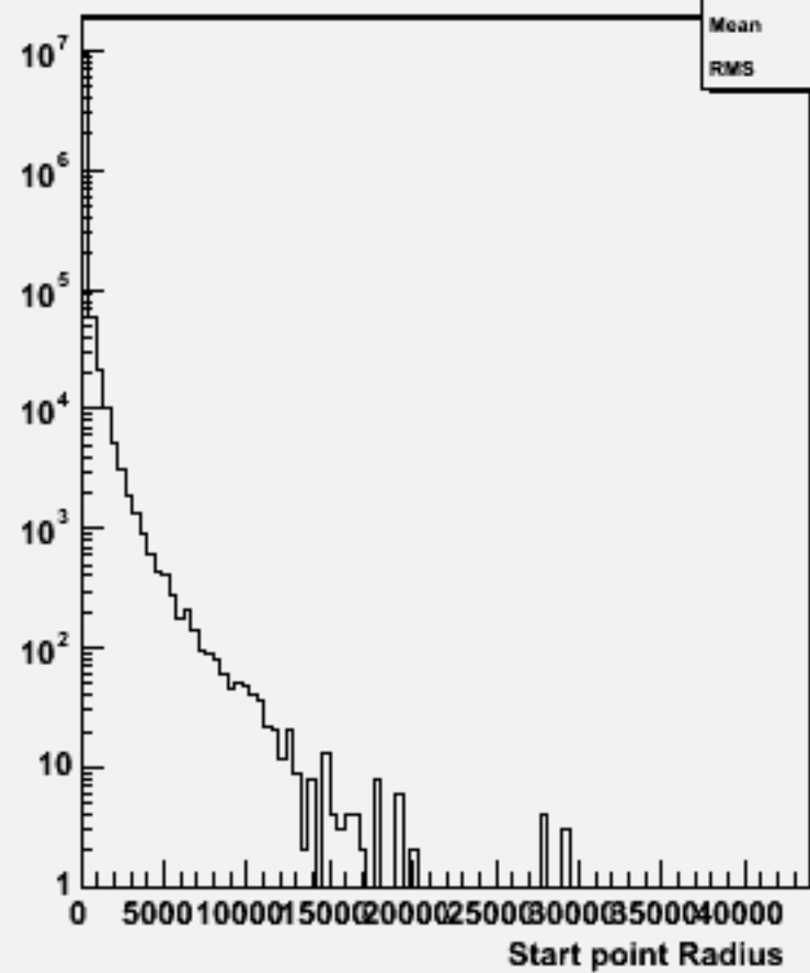
Start point R : w102762 dd_o
