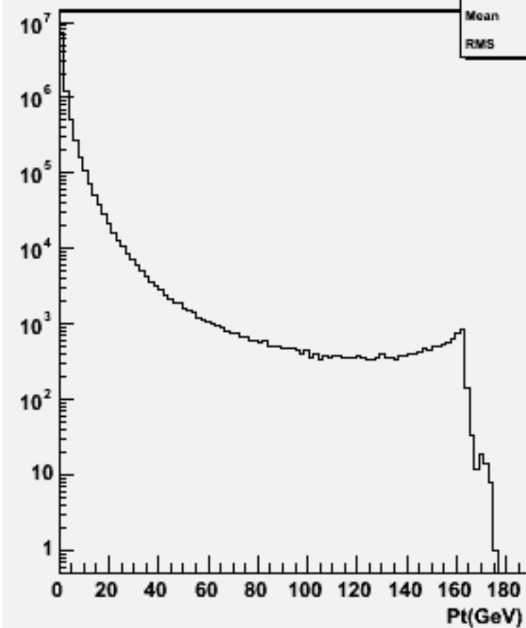
Start point Z : w102762 dd_o
