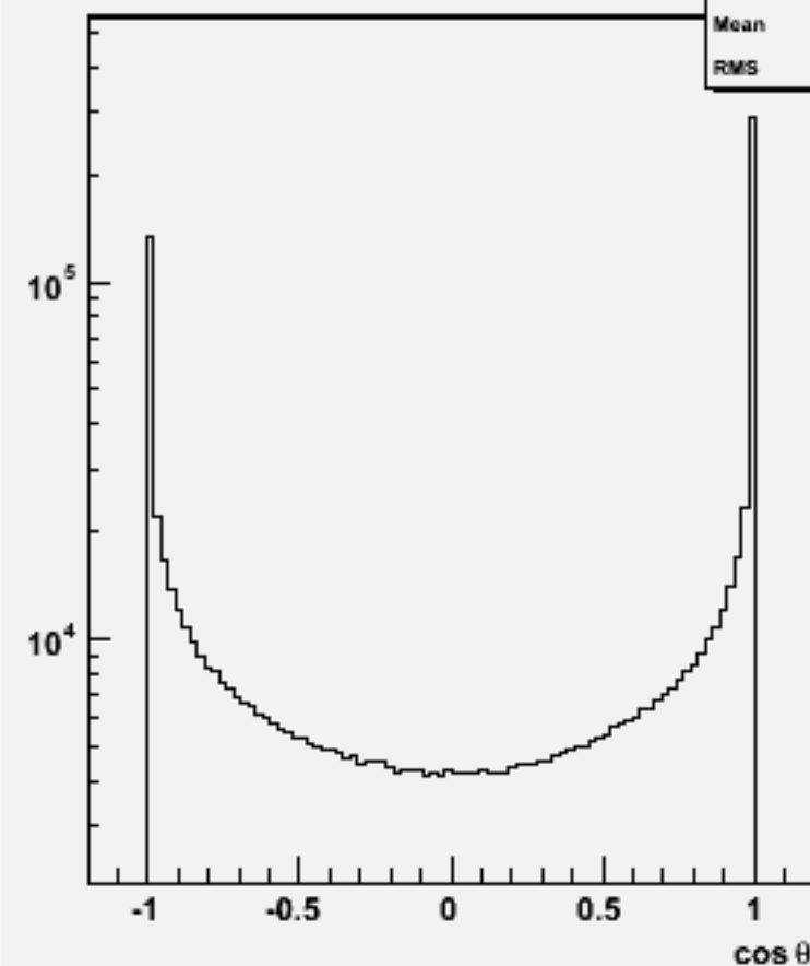
Jet cos \theta (All jets)w102757 e3e3_o
