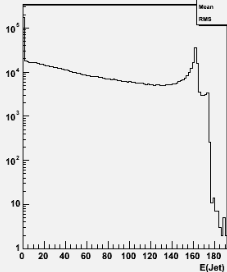
Jet energies(All jets)w102757 e3e3_o
