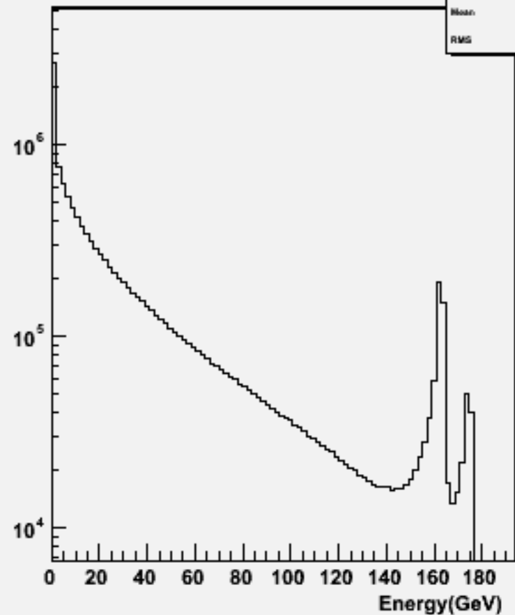
Start point R : w102757 e3e3_o
