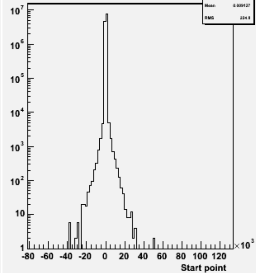
Start point Z : w102757 e3e3_o
