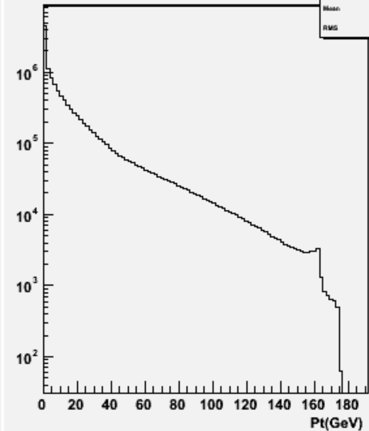
Start point Z : w102757 e3e3_o
