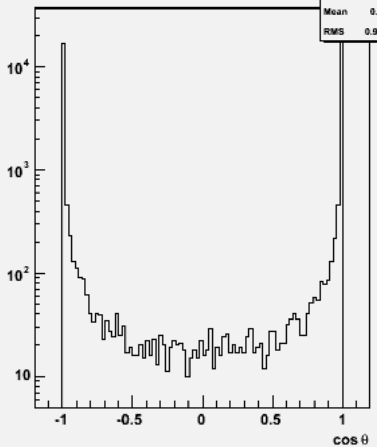
Particle cos \theta : w102750 e1e1_o
