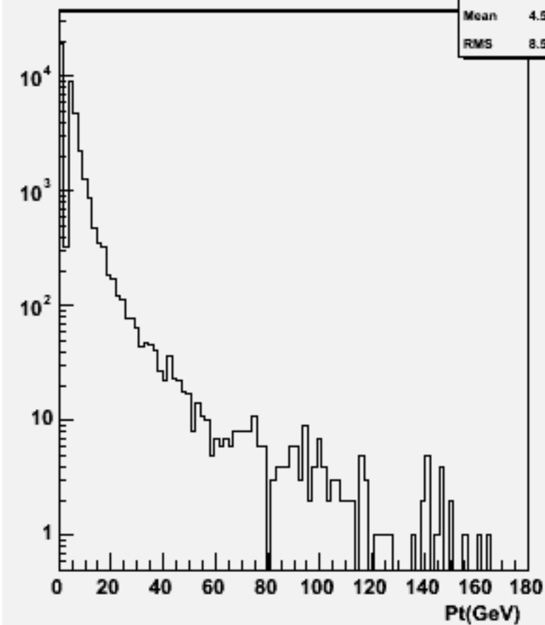
Particle Pt : w102750 e1e1_o
