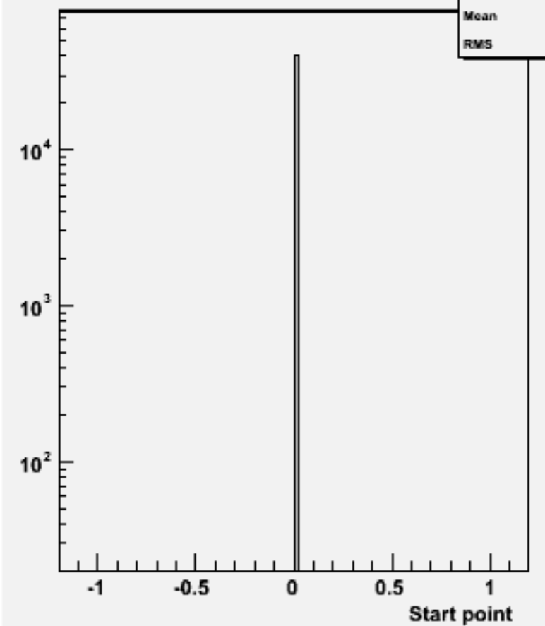
Start point Z : w102750 e1e1_o
