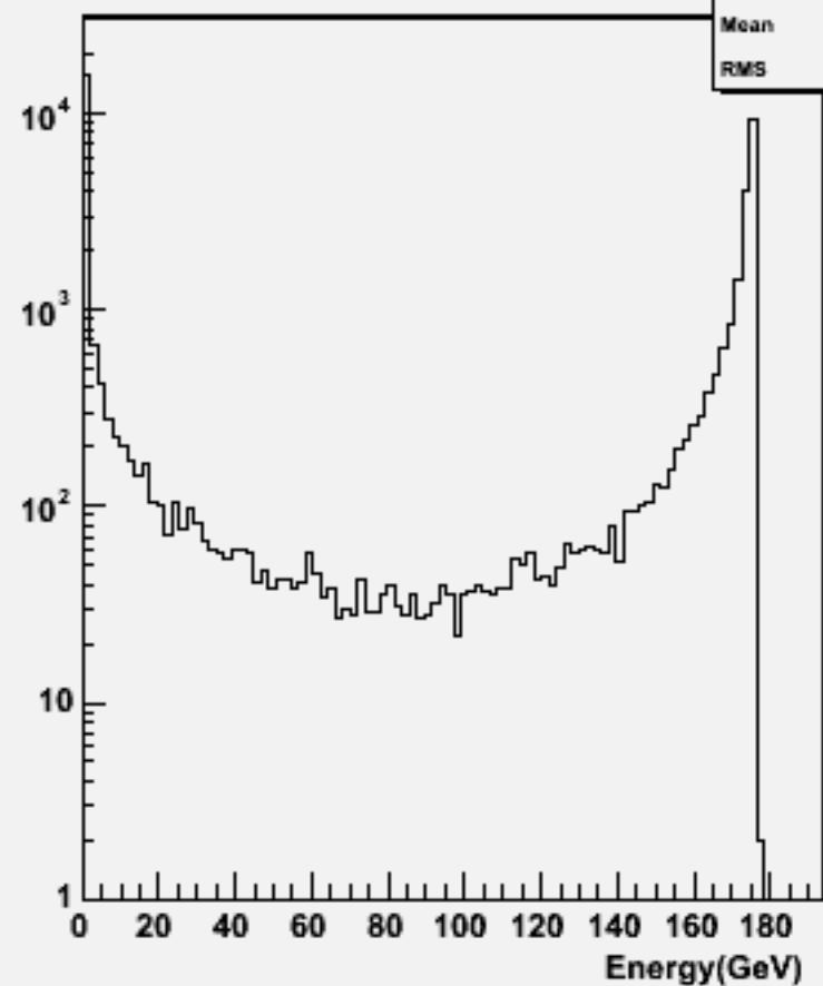
Particle Energy : w102750 e1e1_o
