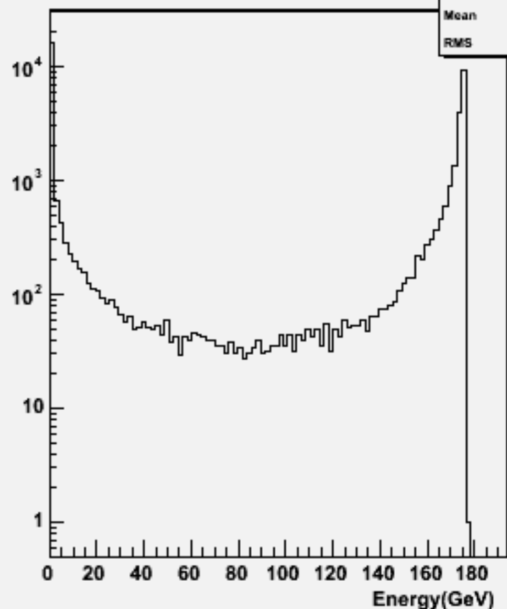
Particle Energy : w102749 e1e1_o
