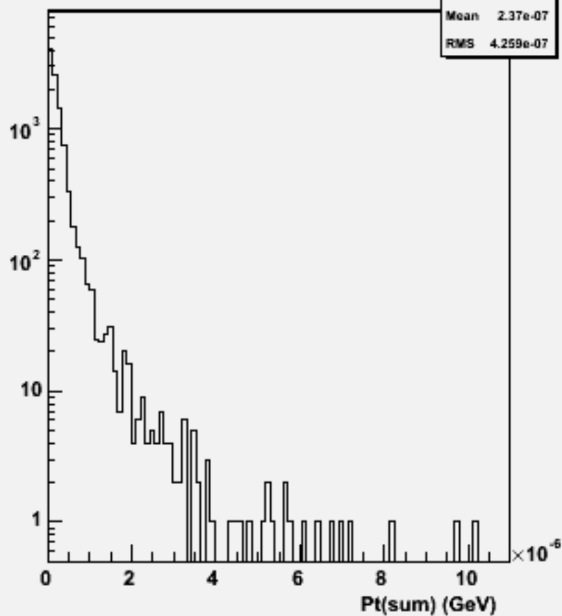
Pt Sum: w102749 e1e1_o
