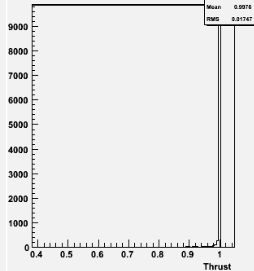
Thrust w102749 e1e1_o
