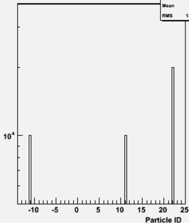
Particle ID : w102749 e1e1_o
