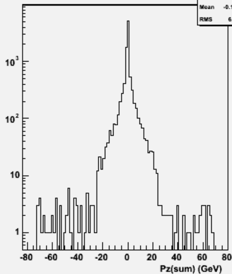
Pz Sum: w102749 e1e1_o
