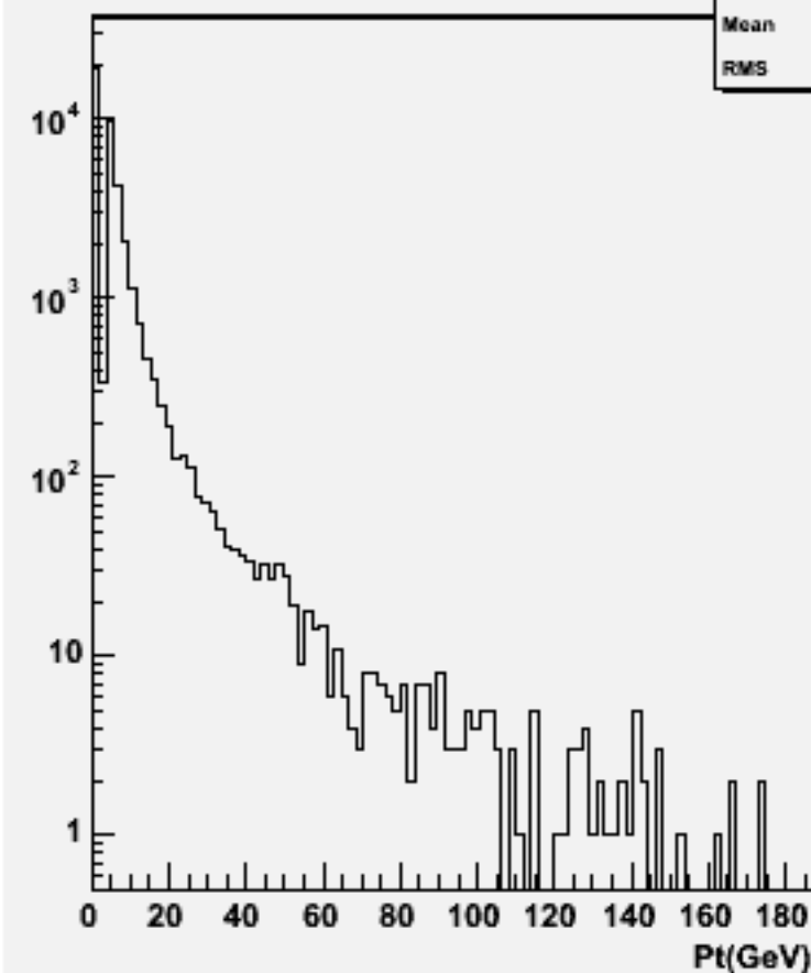
Particle Pt : w102749 e1e1_o
