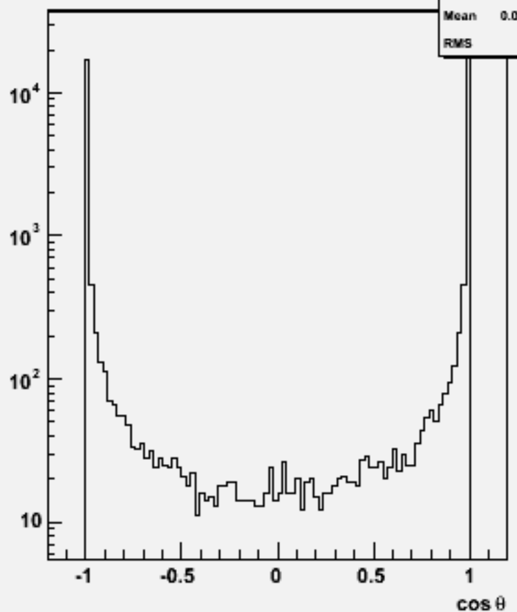
Particle cos \theta : w102749 e1e1_o
