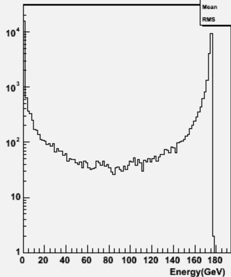
Particle Energy : w102748 e1e1_o
