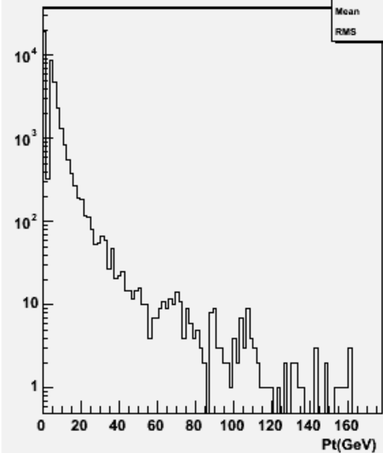
Particle Pt : w102748 e1e1_o
