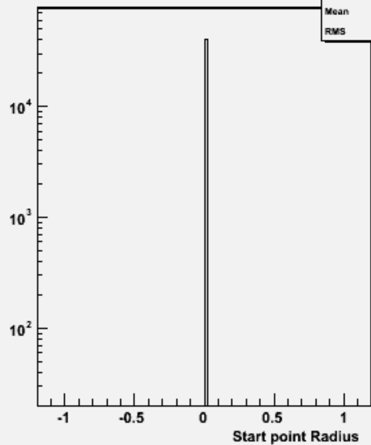
Start point R : w102748 e1e1_o
