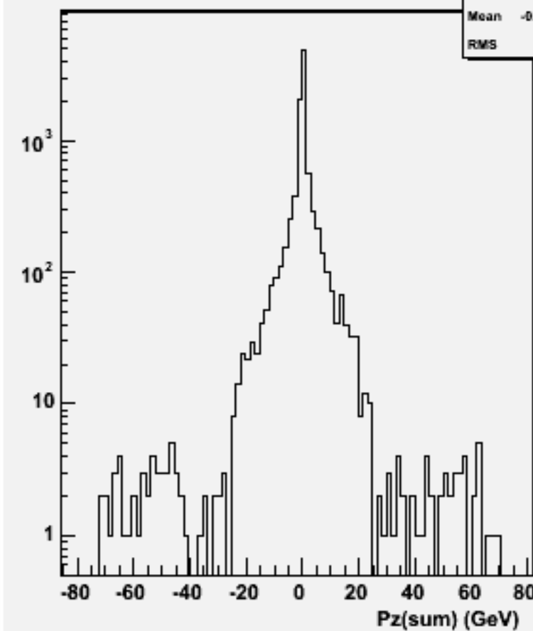
Pz Sum: w102748 e1e1_o
