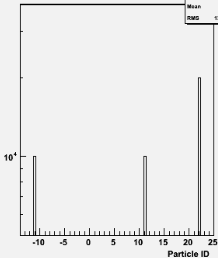
Particle ID : w102748 e1e1_o
