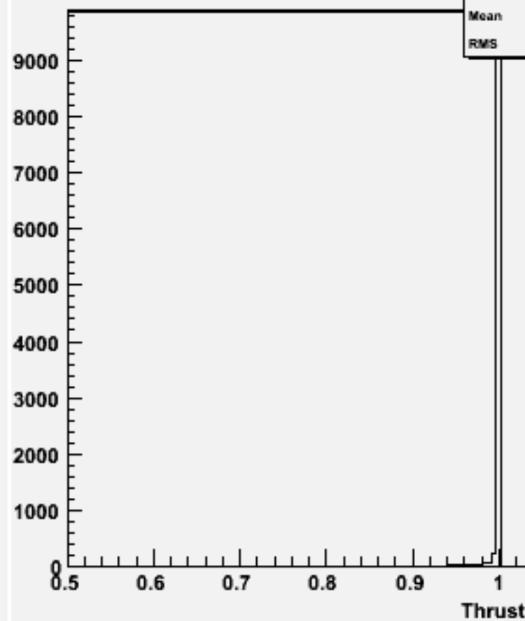
Thrust w102748 e1e1_o
