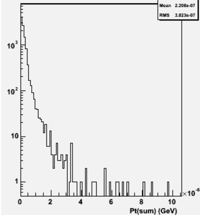
Pt Sum: w102748 e1e1_o
