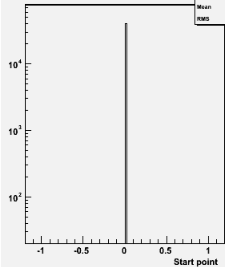
Start point Z : w102748 e1e1_o
