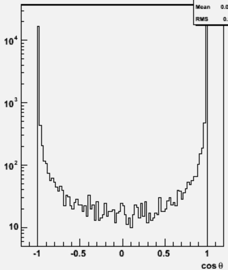
Particle cos \theta : w102748 e1e1_o
