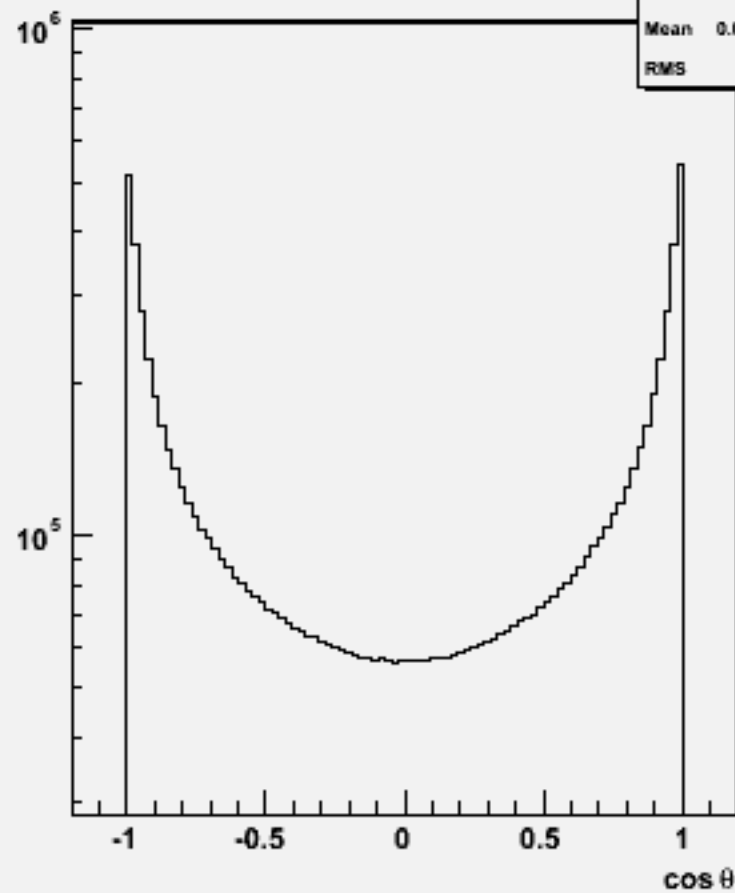
Particle cosθ : w102746 cc_o
