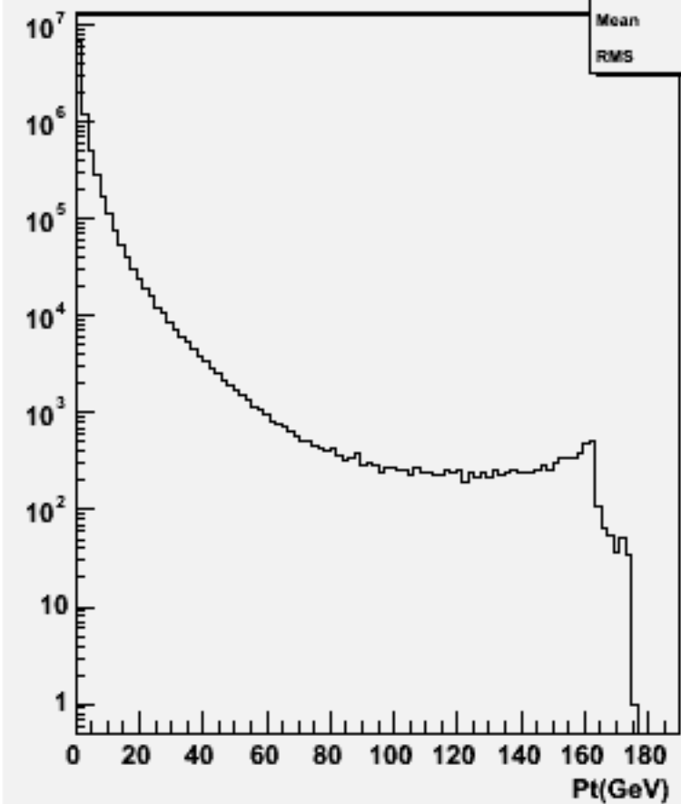
Particle Pt : w102746 cc_o
