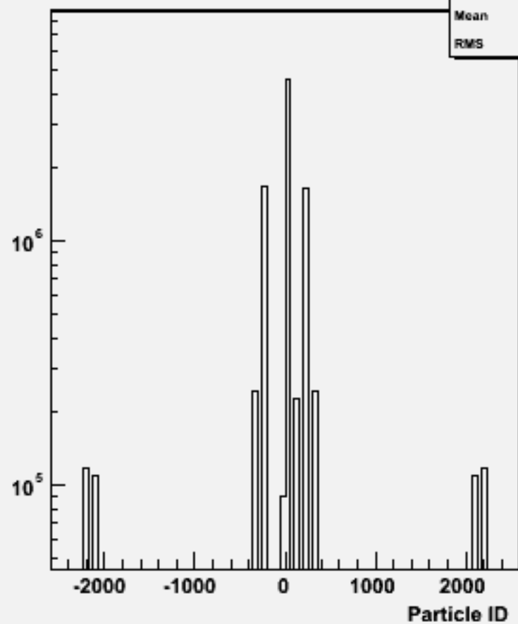
Particle ID : w102746 cc_o
