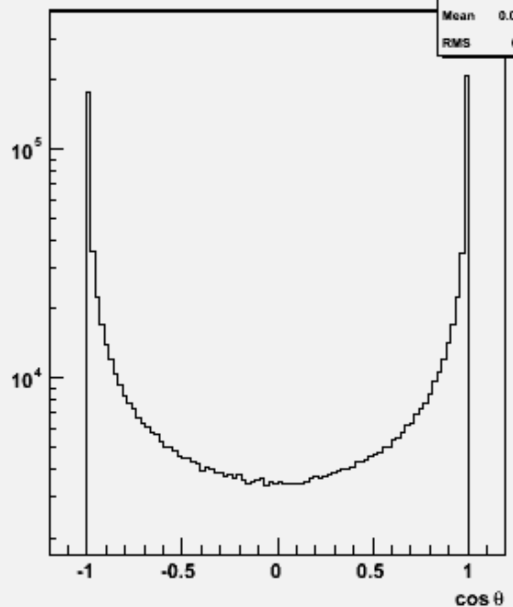
Particle cos \theta : w102726 n3n3aa_o
