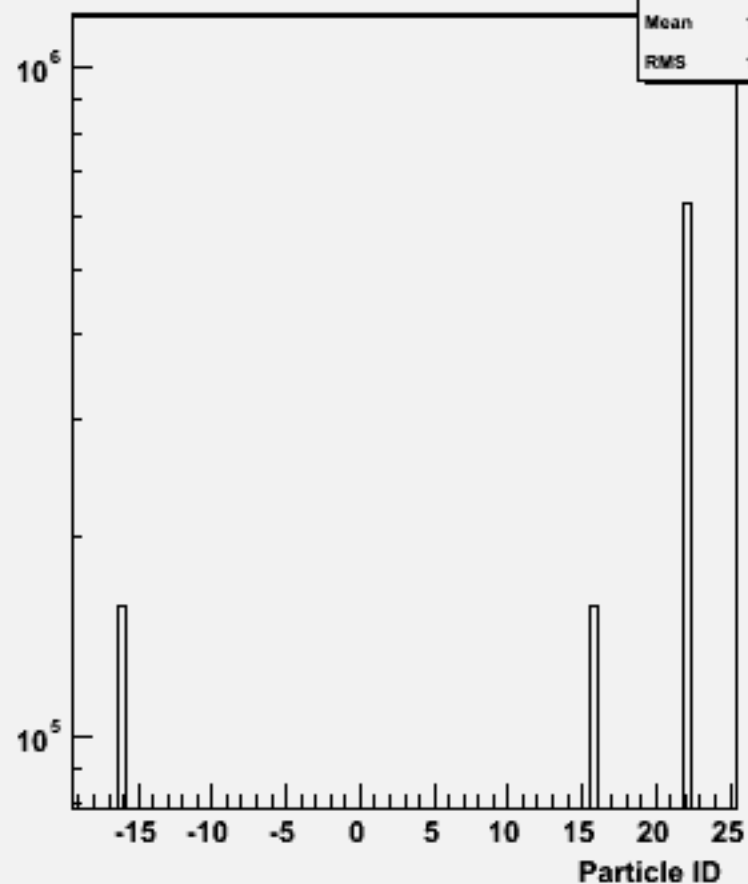
Particle ID : w102726 n3n3aa_o
