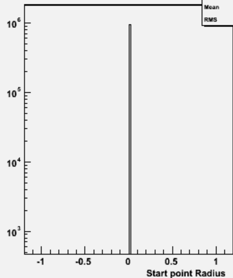
Start point R : w102726 n3n3aa_o
