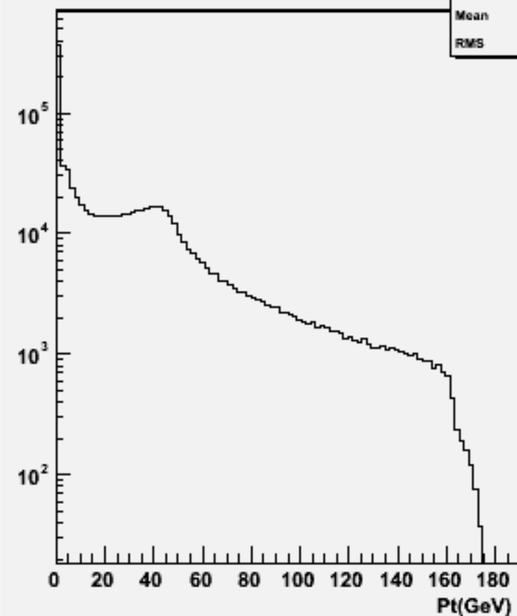
Particle Pt : w102726 n3n3aa_o
