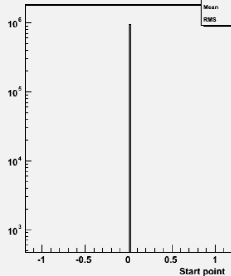
Start point Z : w102726 n3n3aa_o
