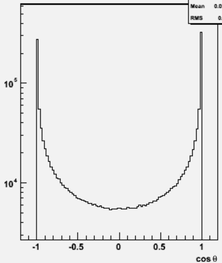
Particle cosθ : w102725 n3n3aa_o
