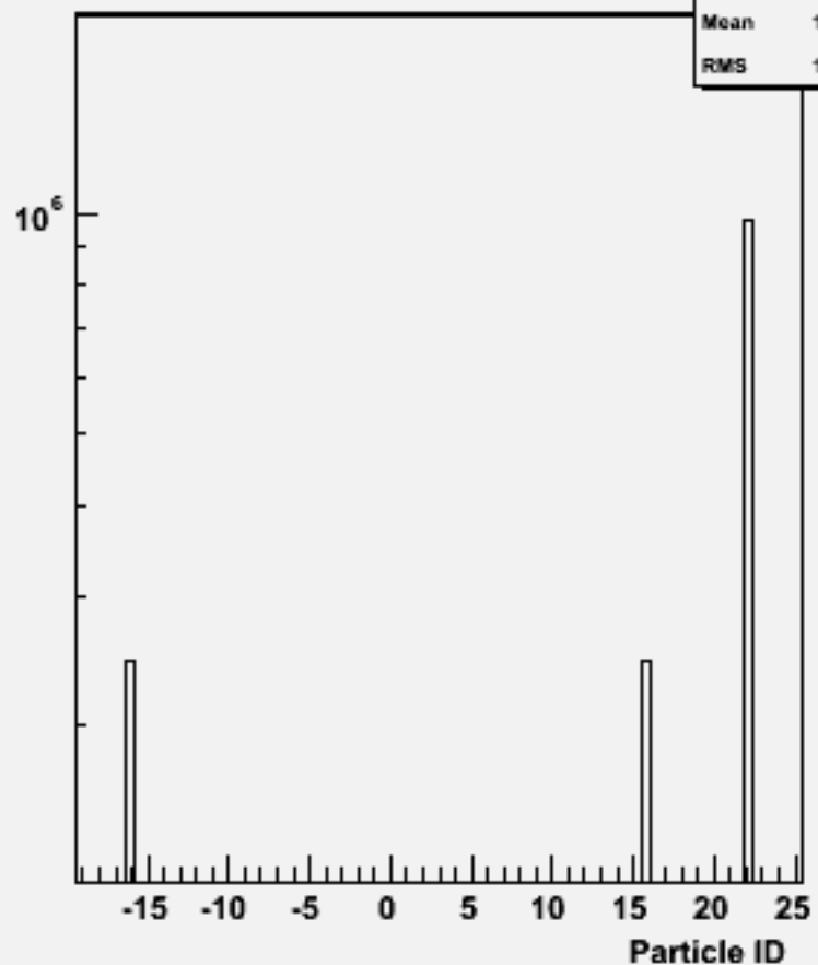
Particle ID : w102725 n3n3aa_o
