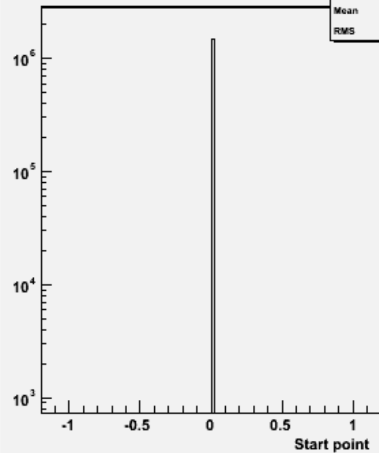
Start point Z : w102725 n3n3aa_o
