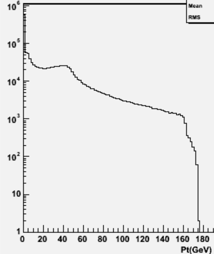
Particle Pt : w102725 n3n3aa_o
