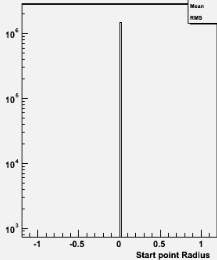
Start point R : w102725 n3n3aa_o
