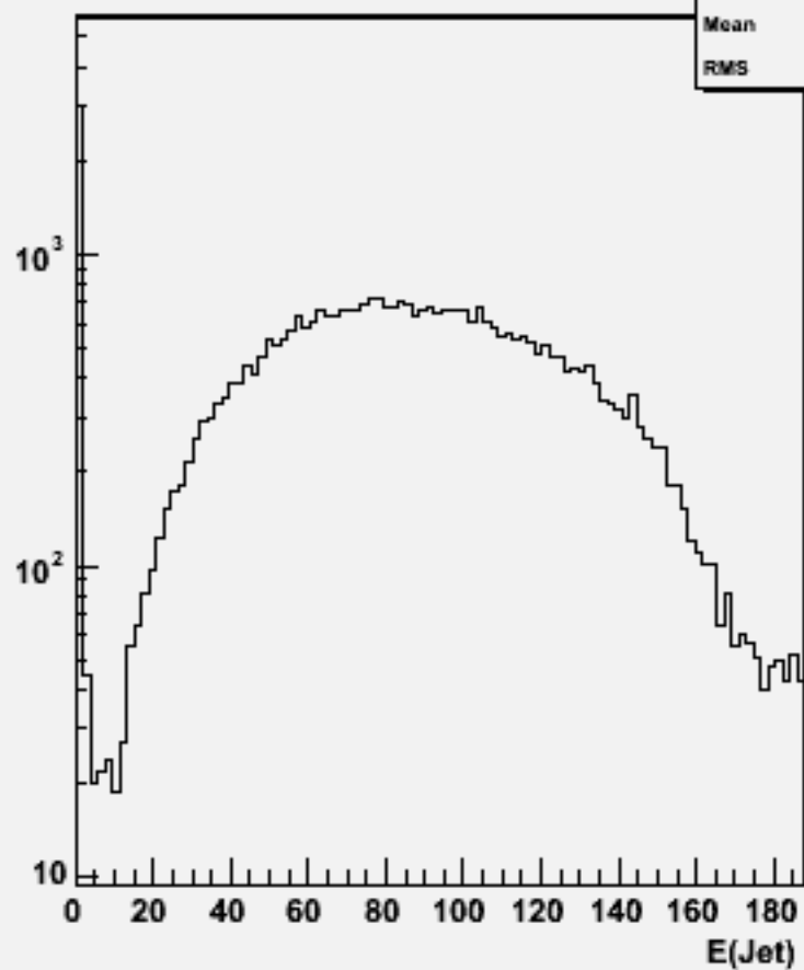
Jet energies(All jets)w102593 e2e2ssbb_o
