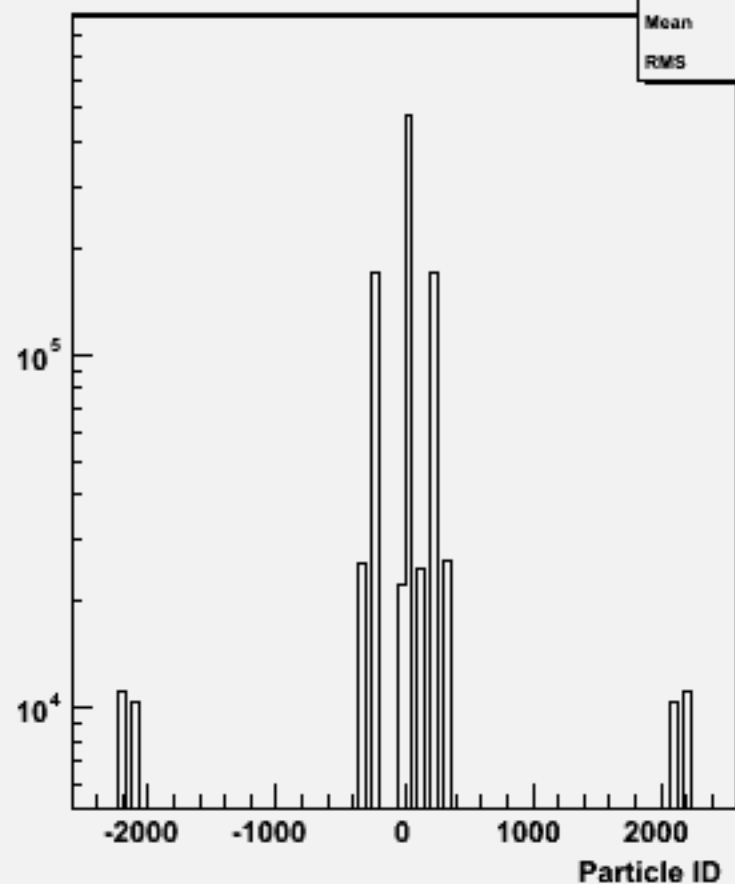
Particle ID : w102593 e2e2ssbb_o
