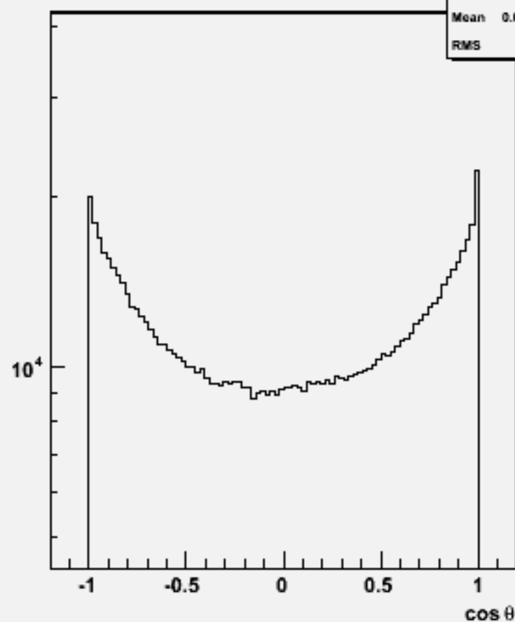
Particle cos \theta : w102593 e2e2ssbb_o
