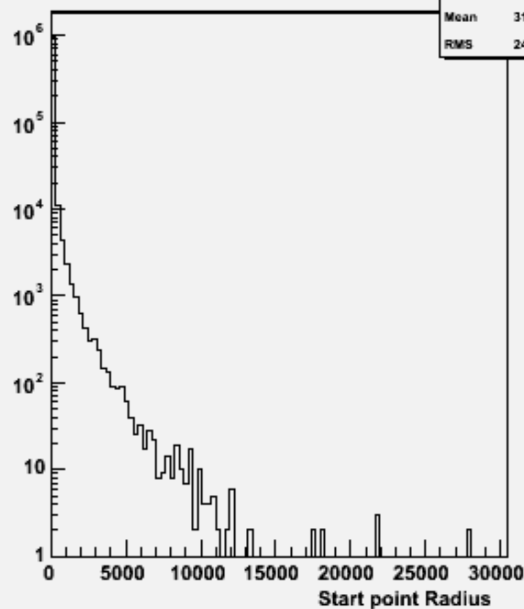
Start point R : w102593 e2e2ssbb_o
