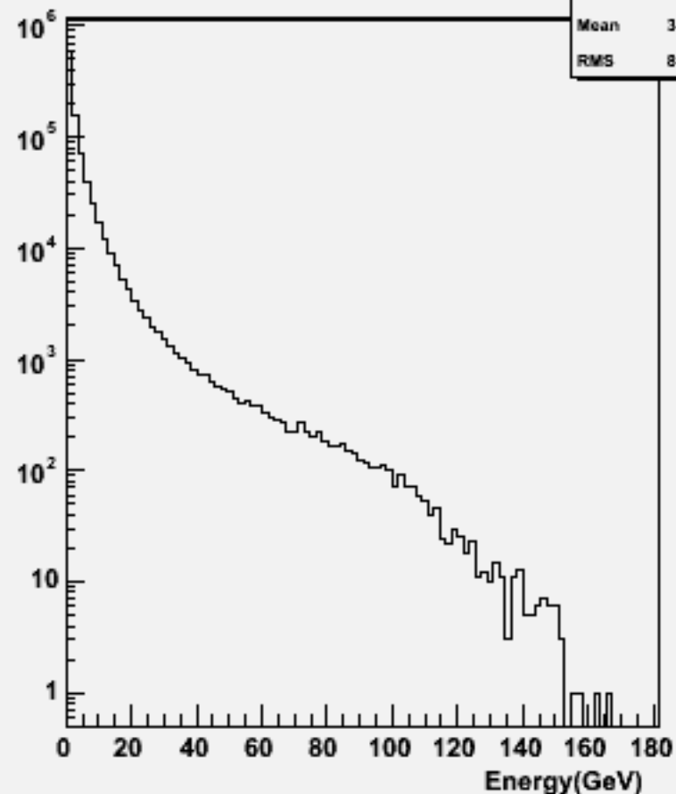
Particle Energy : w102593 e2e2ssbb_o
