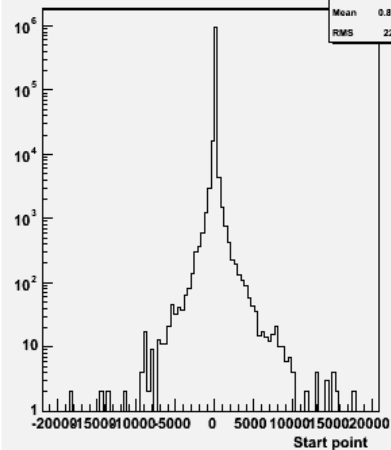
Start point Z : w102593 e2e2ssbb_o
