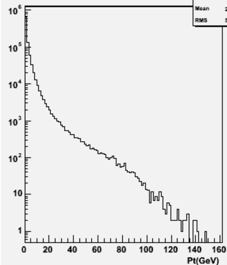
Particle Pt : w102593 e2e2ssbb_o
