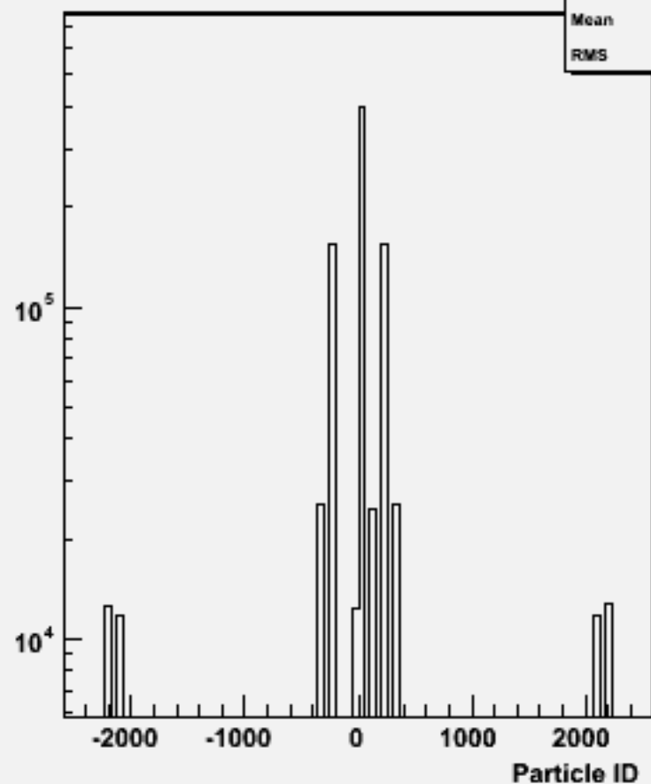
Particle ID : w102589 e2e2ssss_o
