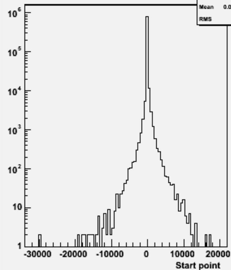
Start point Z : w102589 e2e2ssss_o
