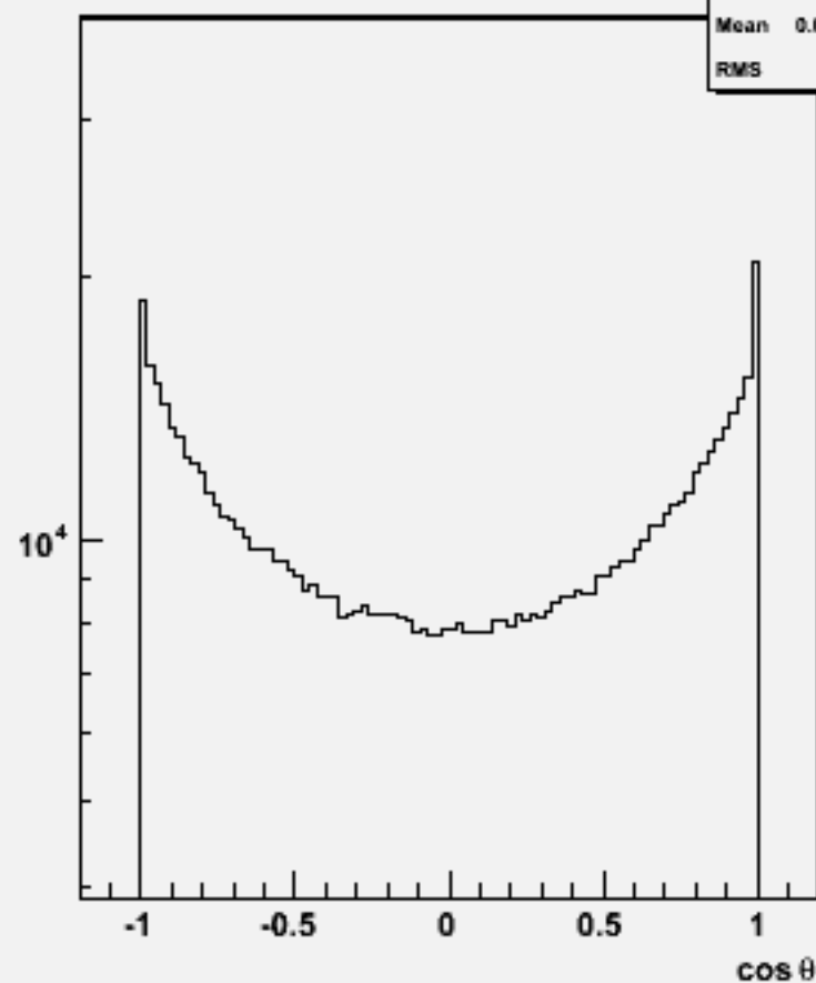
Particle cos \theta : w102589 e2e2ssss_o
