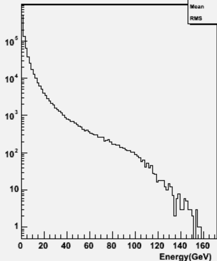
Particle Energy : w102589 e2e2ssss_o
