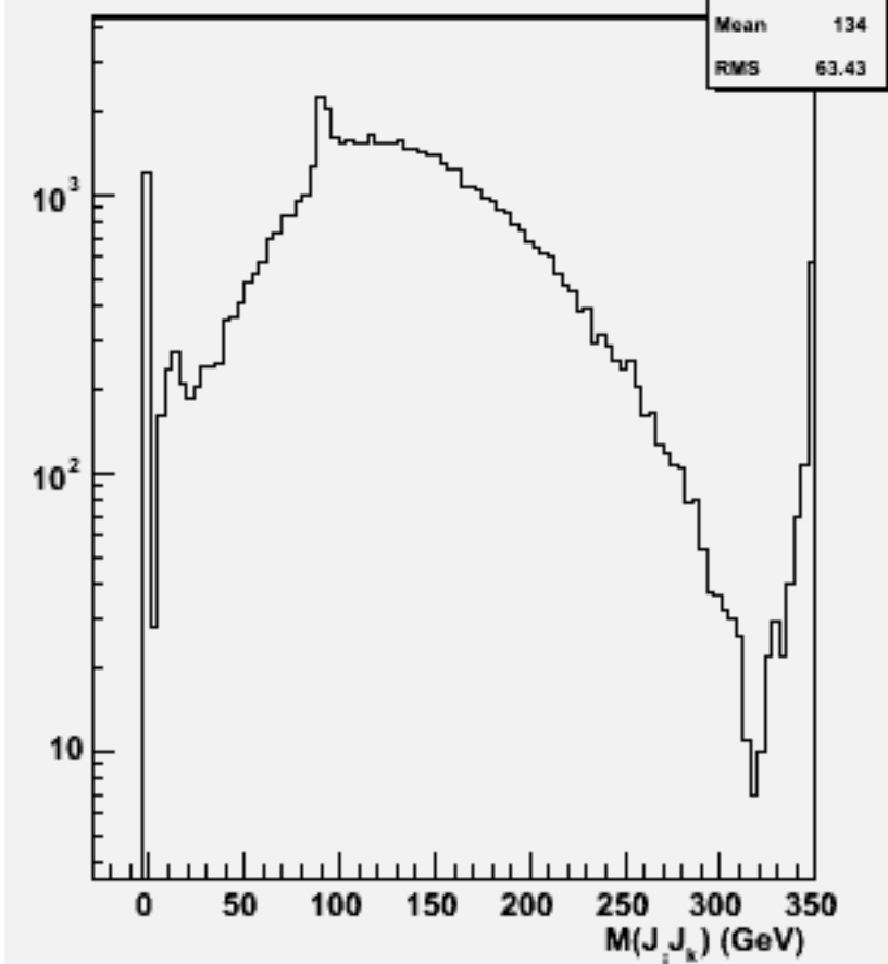
2jets mass(All comb)w102589 e2e2ssss_o
