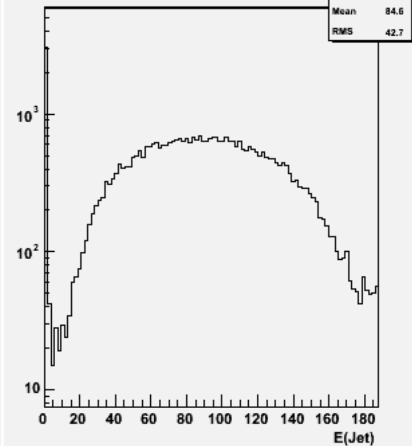
Jet energies(All jets)w102589 e2e2ssss_o
