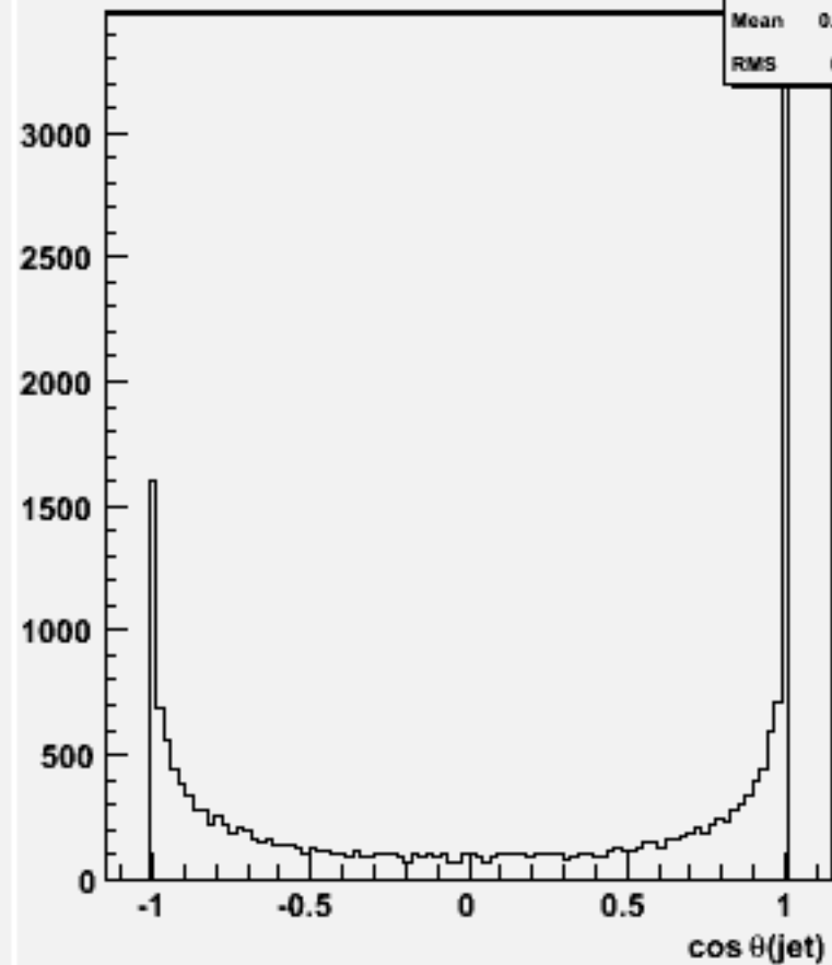
cos \theta for 2-jets :w102589 e2e2ssss_o
