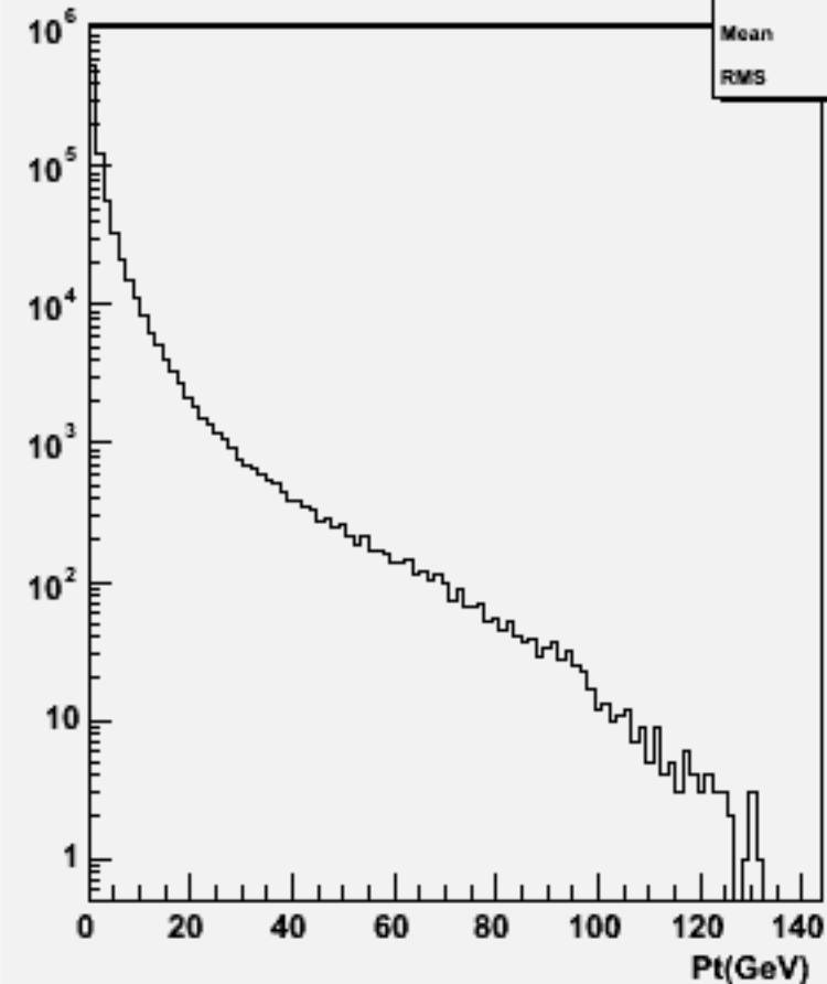
Particle Pt : w102589 e2e2ssss_o
