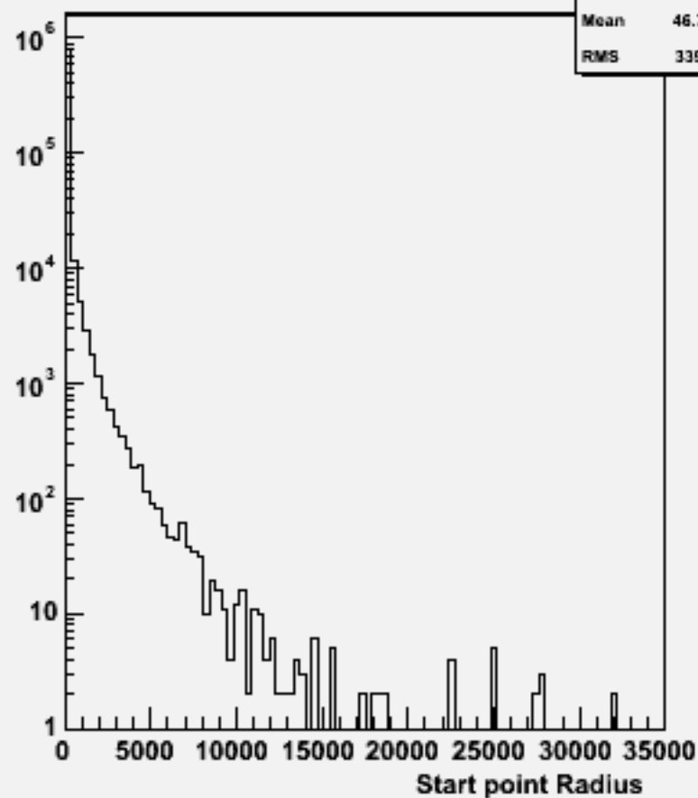
Start point R : w102589 e2e2ssss_o
