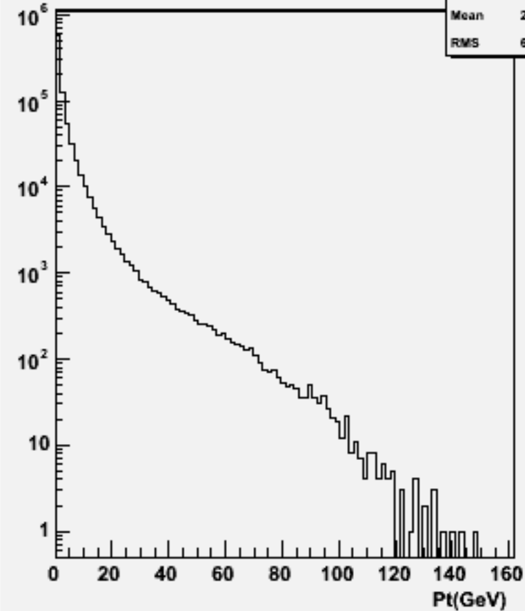
Particle Pt : w102588 e2e2ssss_o
