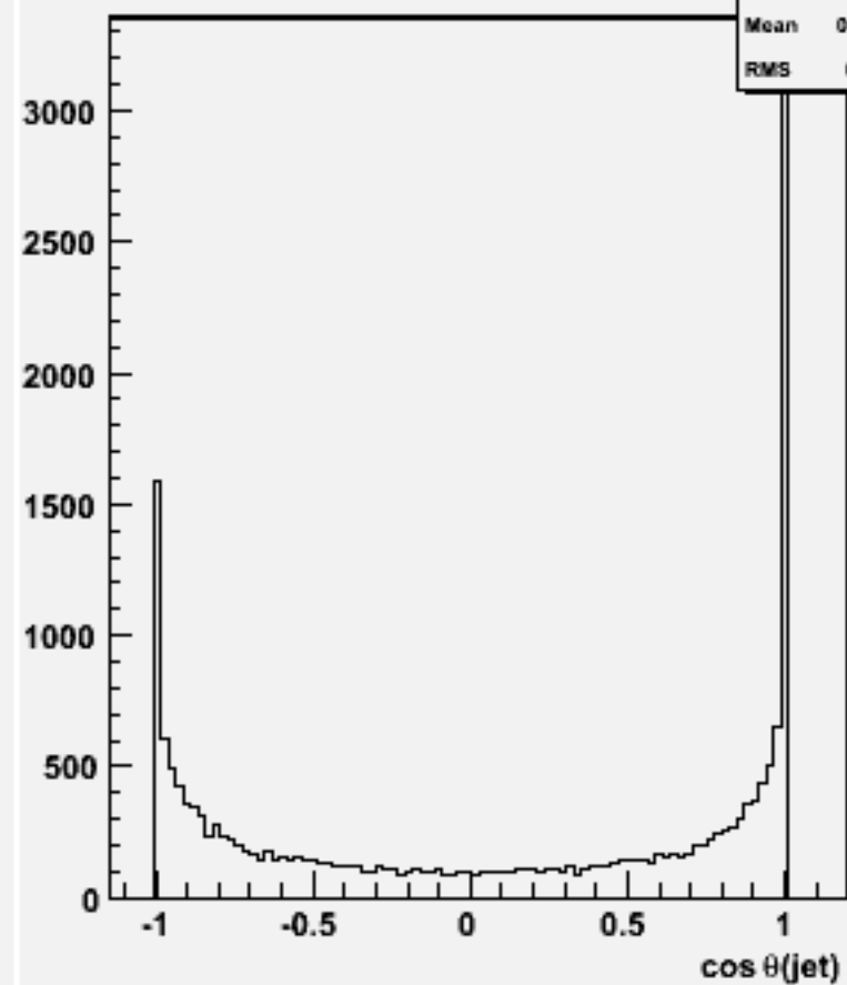
cos \theta for 2-jets :w102588 e2e2ssss_o
