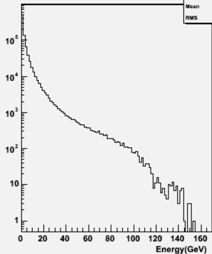
Particle Energy : w102588 e2e2ssss_o
