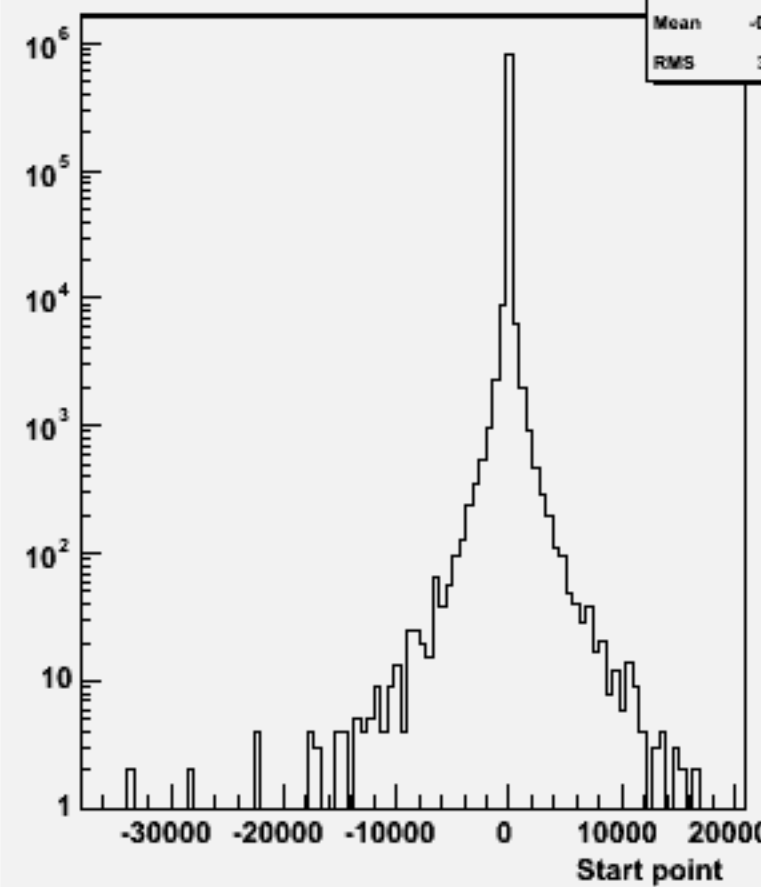
Start point Z : w102588 e2e2ssss_o
