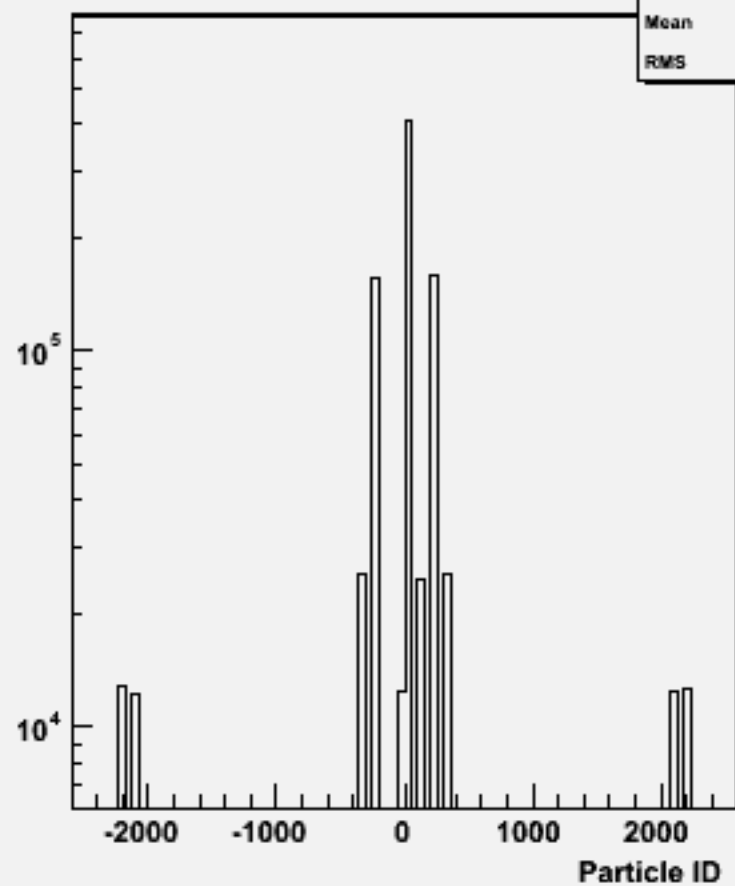
Particle ID : w102588 e2e2ssss_o
