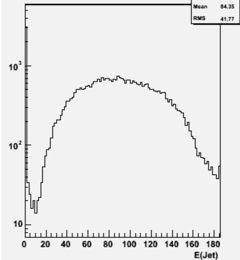
Jet energies(All jets)w102588 e2e2ssss_o
