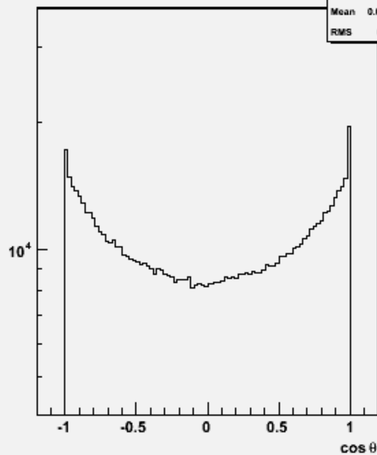
Particle cos \theta : w102588 e2e2ssss_o
