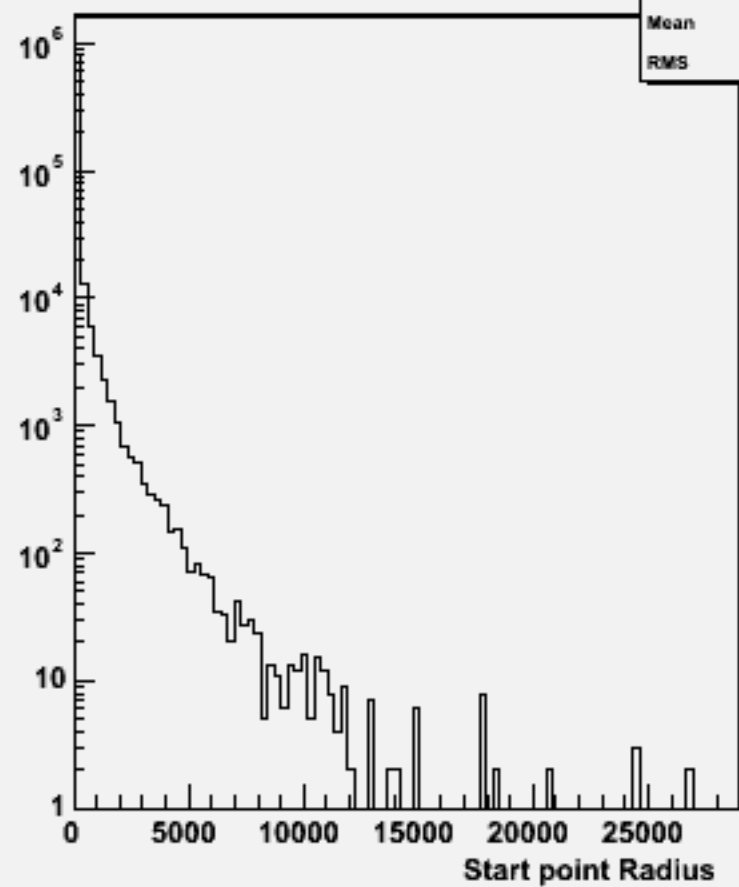
Start point R : w102588 e2e2ssss_o
