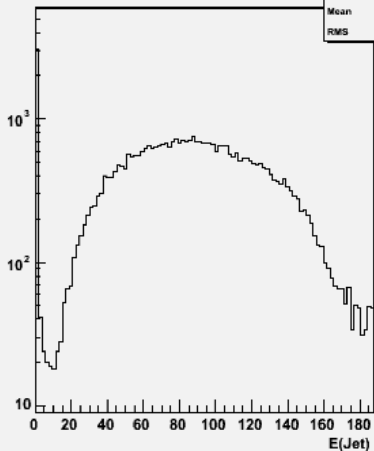
Jet energies(All jets)w102584 e2e2ddb_o
