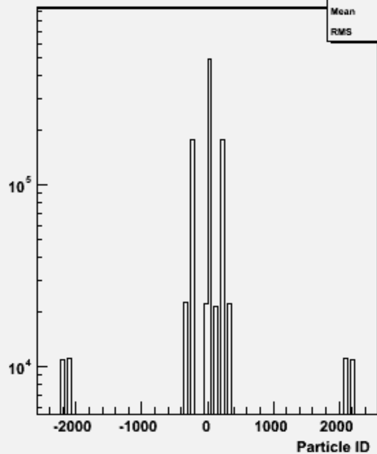
Particle ID : w102584 e2e2ddb_o
