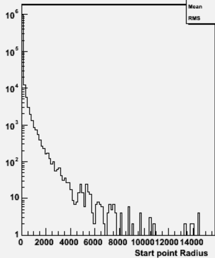
Start point R : w102584 e2e2ddb_o
