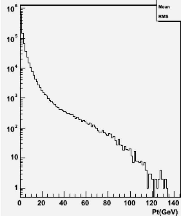
Particle Pt : w102584 e2e2ddb_o
