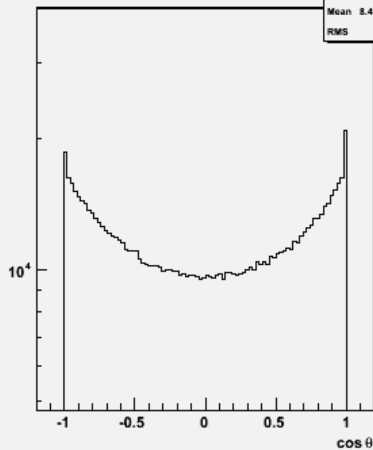
Particle cos \theta : w102584 e2e2ddb_o
