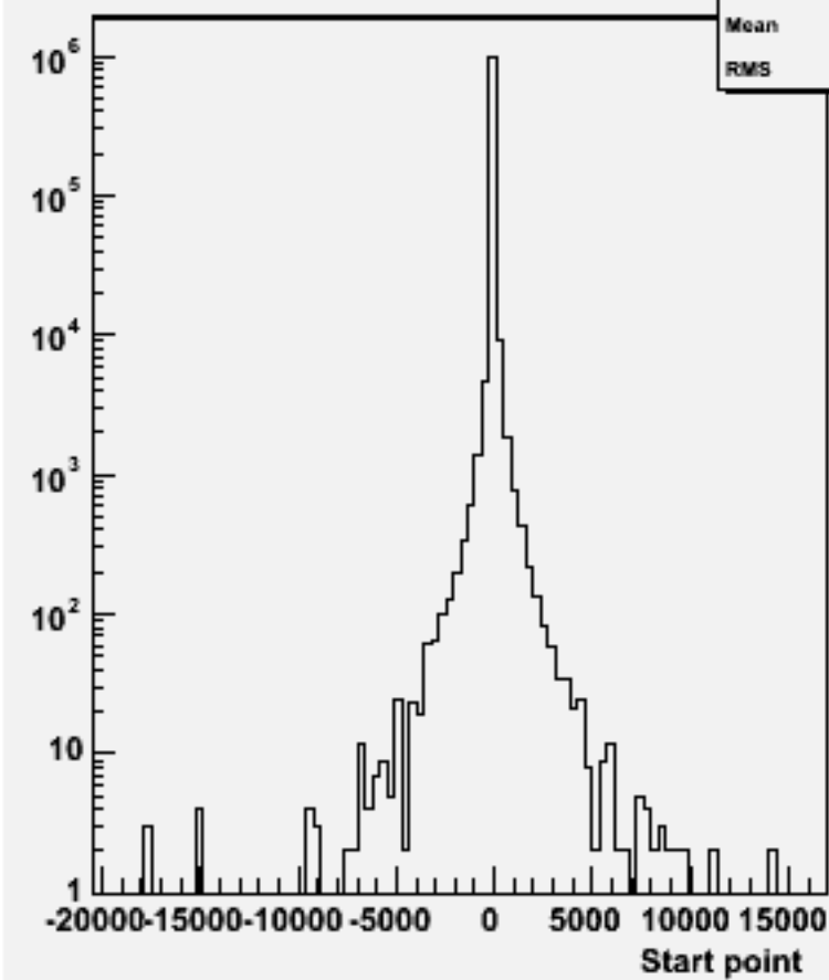
Start point Z : w102584 e2e2ddb_o
