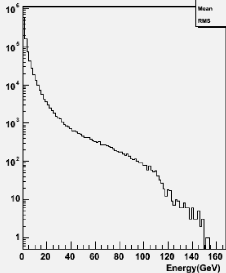
Particle Energy : w102584 e2e2ddb_o
