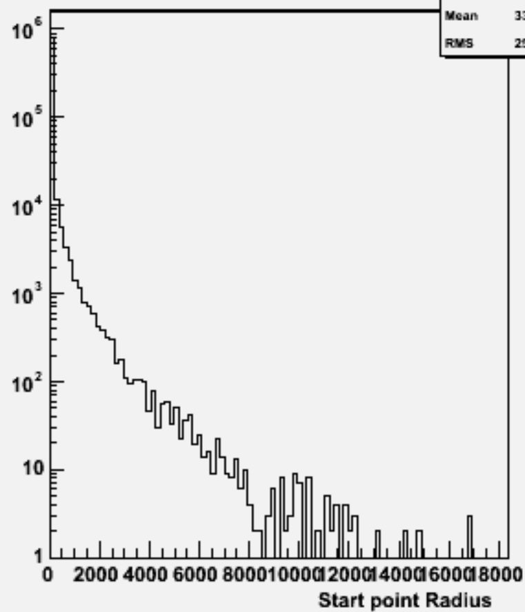
Start point R : w102581 e2e2ddss_o
