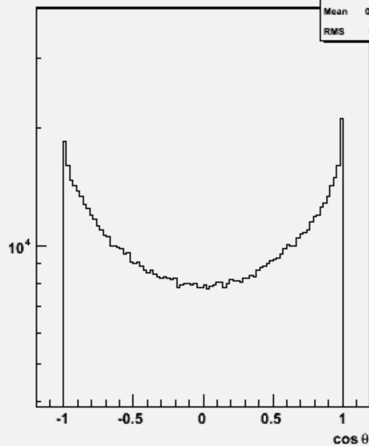
Particle cos \theta : w102581 e2e2ddss_o
