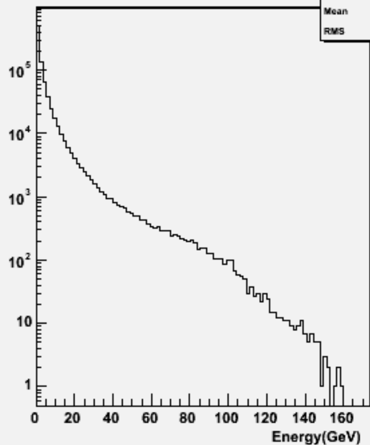
Particle Energy : w102581 e2e2ddss_o
