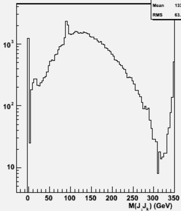
2jets mass(All comb)w102581 e2e2ddss_o
