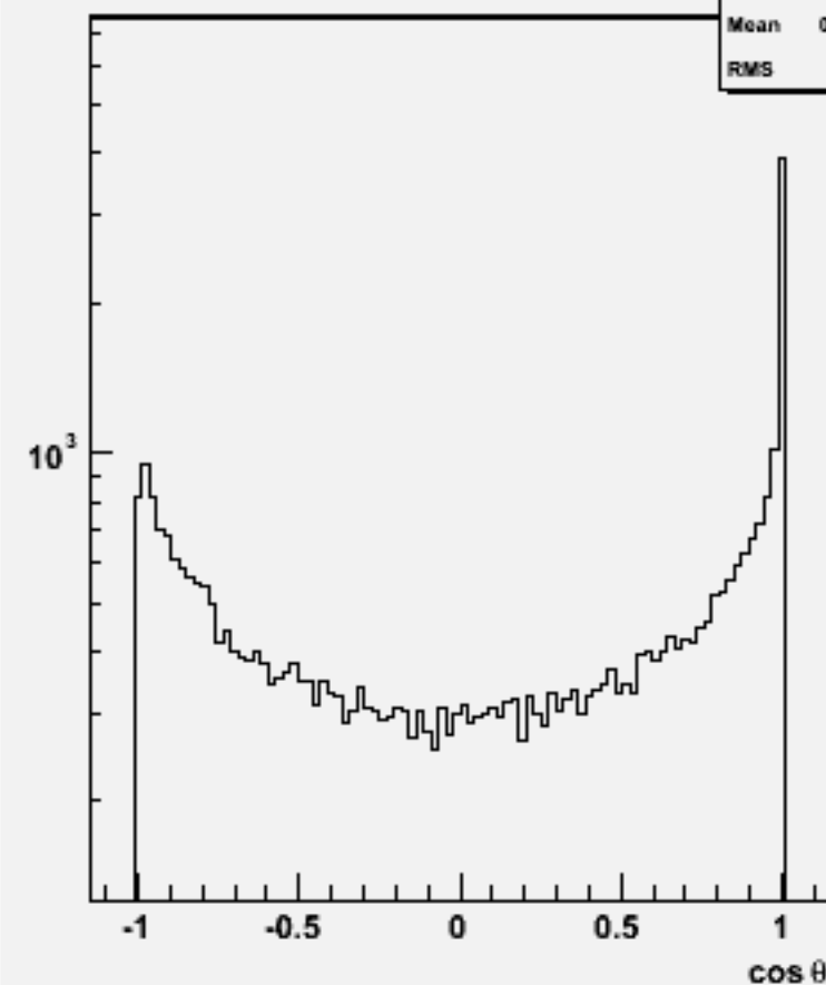
Jet cos \theta (All jets)w102581 e2e2ddss_o
