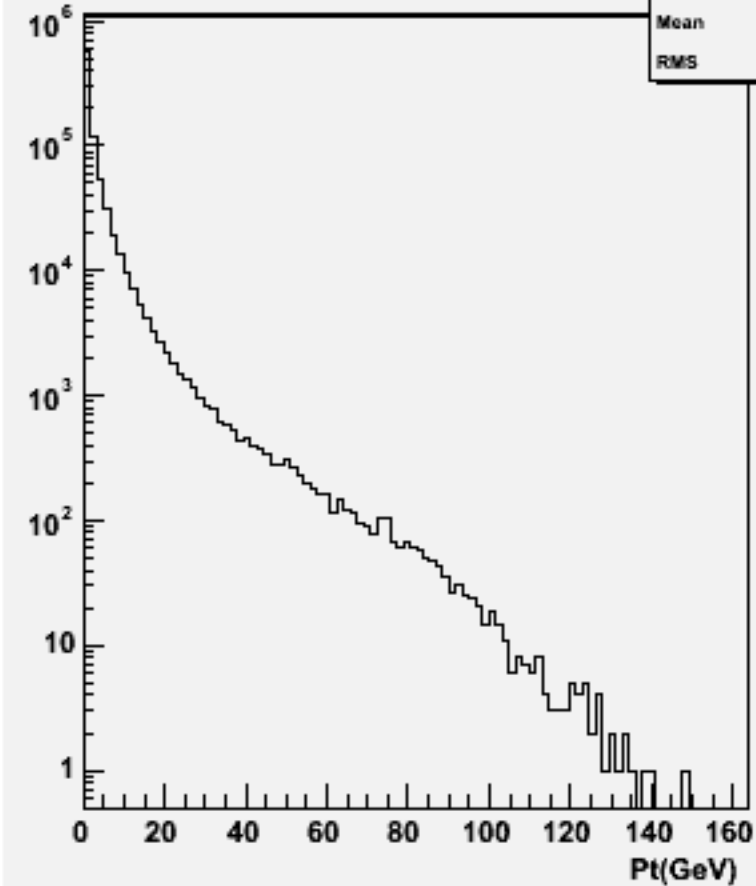
Particle Pt : w102581 e2e2ddss_o
