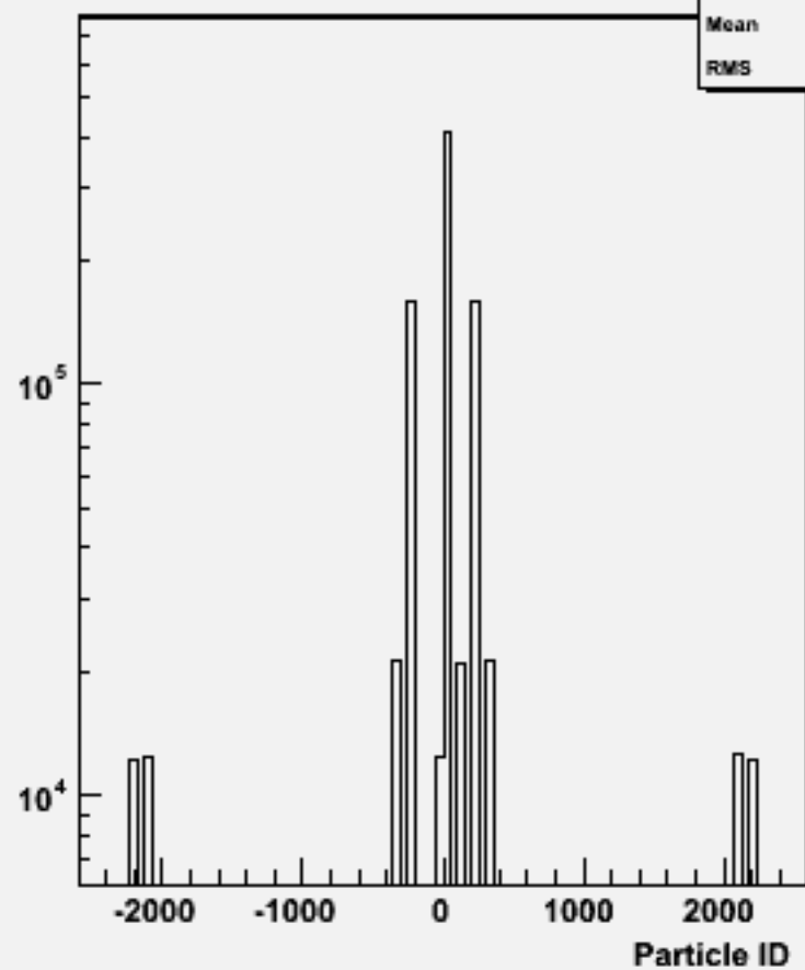
Particle ID : w102581 e2e2ddss_o
