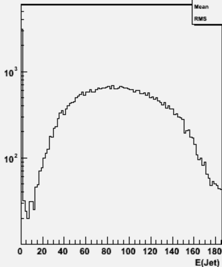
Jet energies(All jets)w102581 e2e2ddss_o
