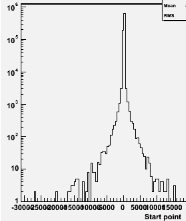
Start point Z : w102581 e2e2ddss_o
