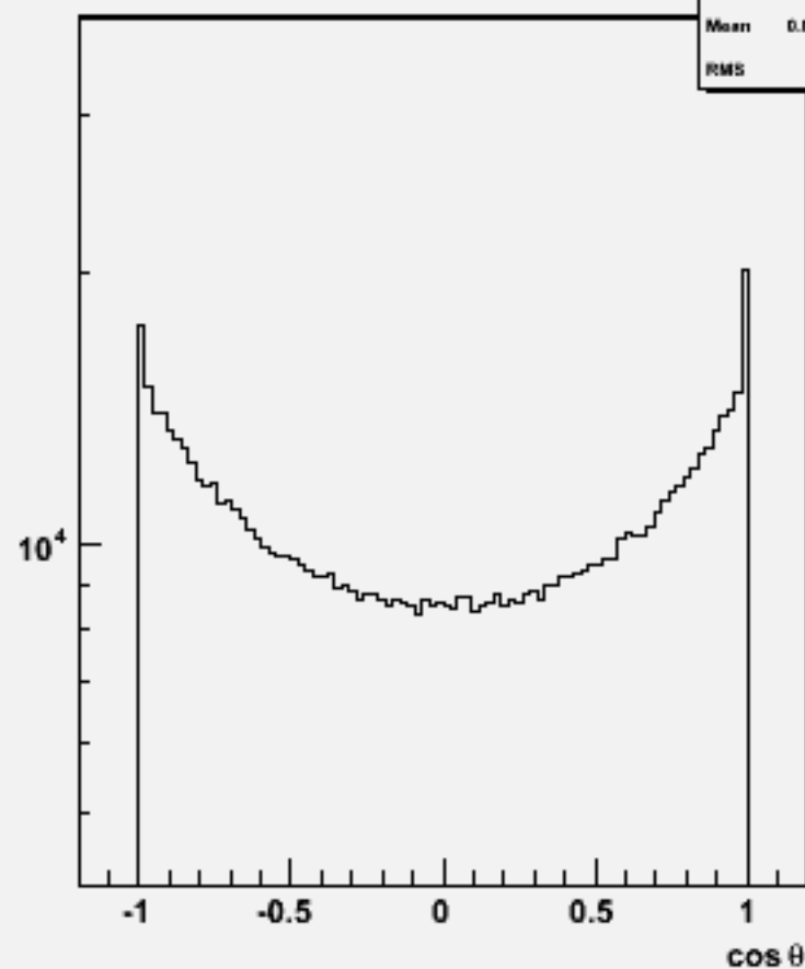
Particle cos \theta : w102576 e2e2dddd_o
