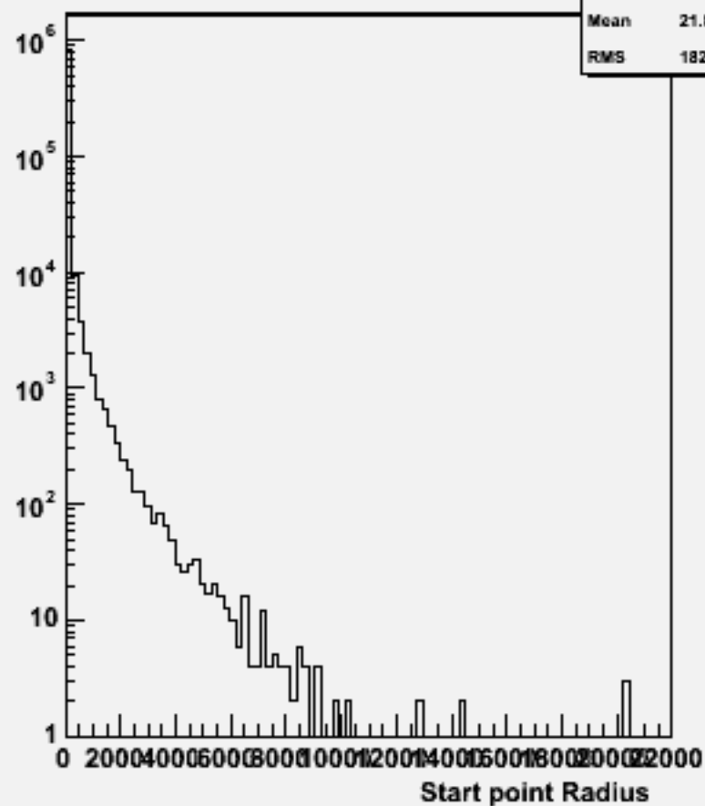
Start point R : w102576 e2e2dddd_o
