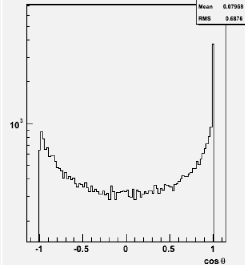
Jet cos \theta (All jets)w102576 e2e2dddd_o
