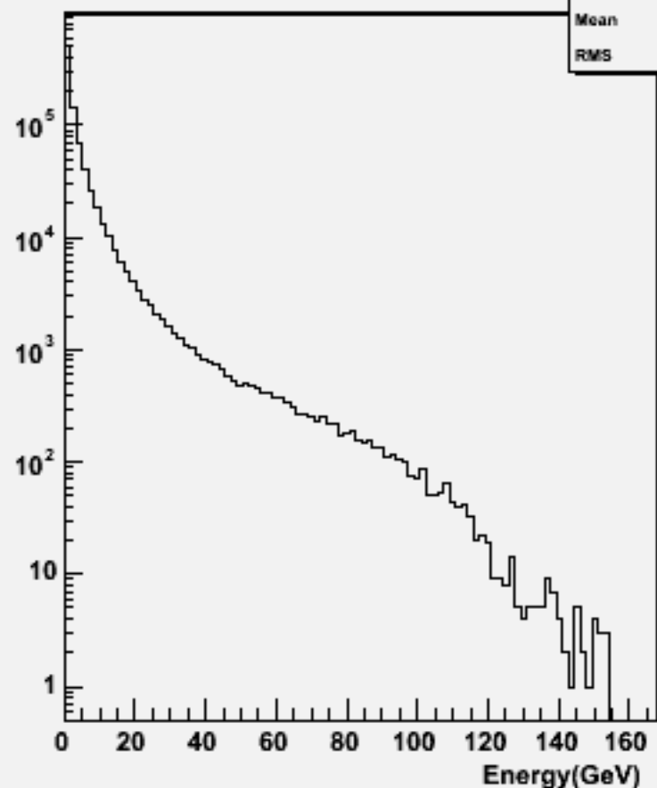
Particle Energy : w102576 e2e2dddd_o
