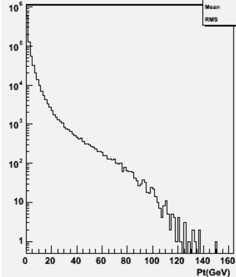
Particle Pt : w102576 e2e2dddd_o
