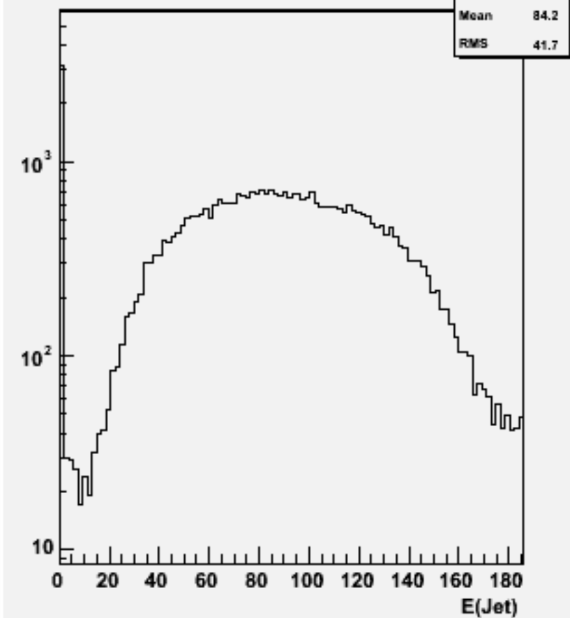
Jet energies(All jets)w102576 e2e2dddd_o
