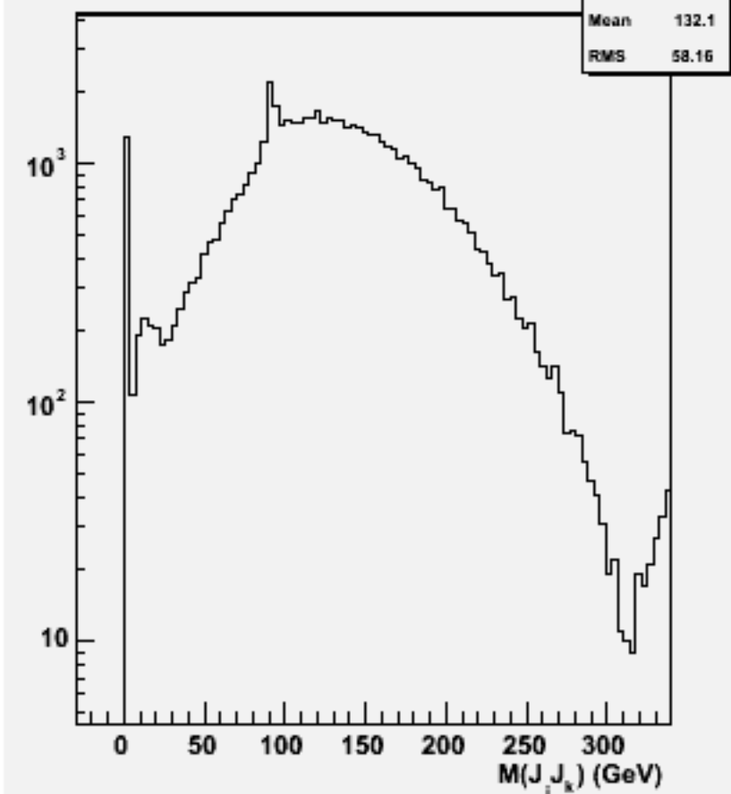
2jets mass(All comb)w102576 e2e2dddd_o
