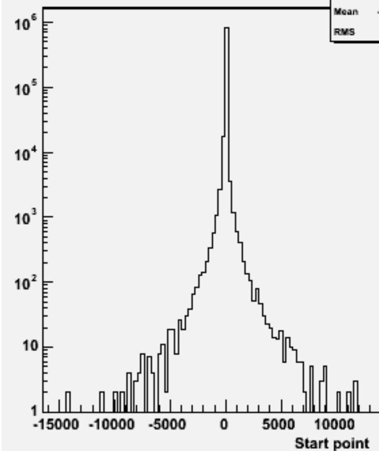
Start point Z : w102576 e2e2dddd_o
