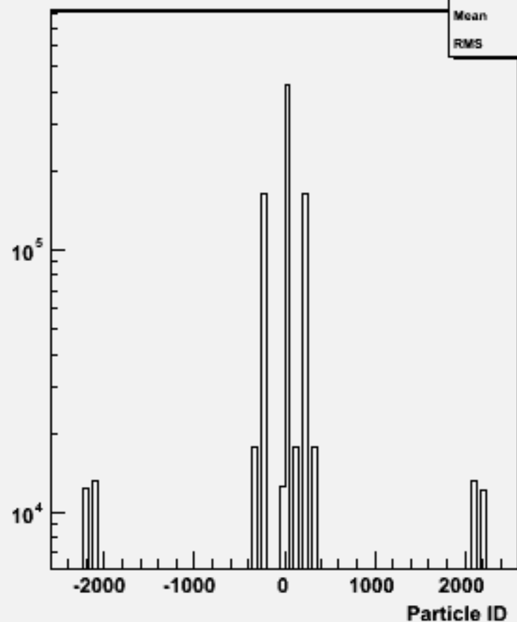
Particle ID : w102576 e2e2dddd_o
