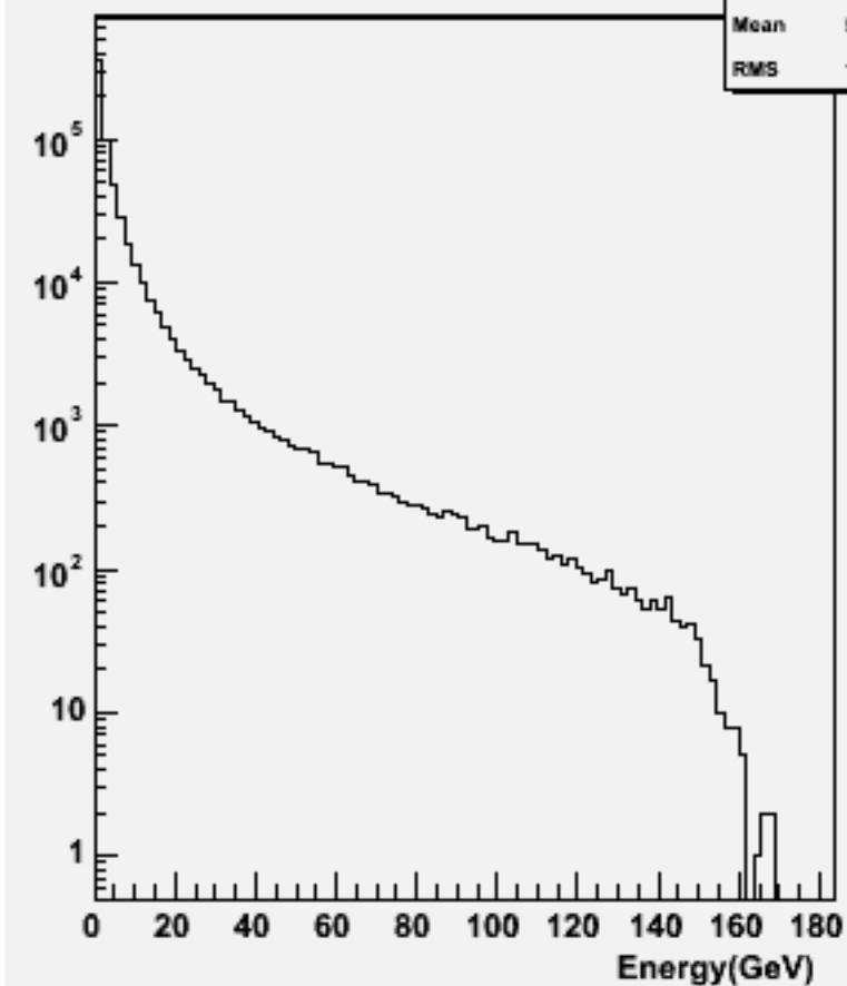
Particle Energy : w102573 e2e2e3e3bb_o
