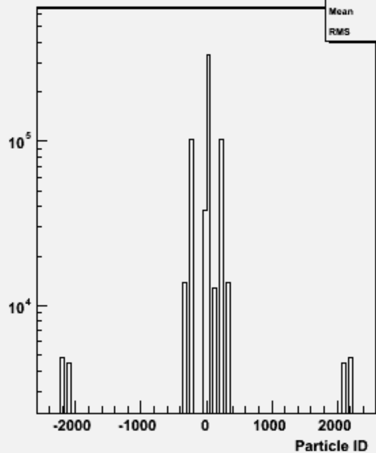
Particle ID : w102573 e2e2e3e3bb_o
