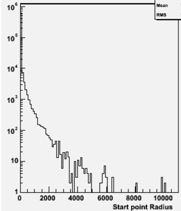
Start point R : w102573 e2e2e3e3bb_o
