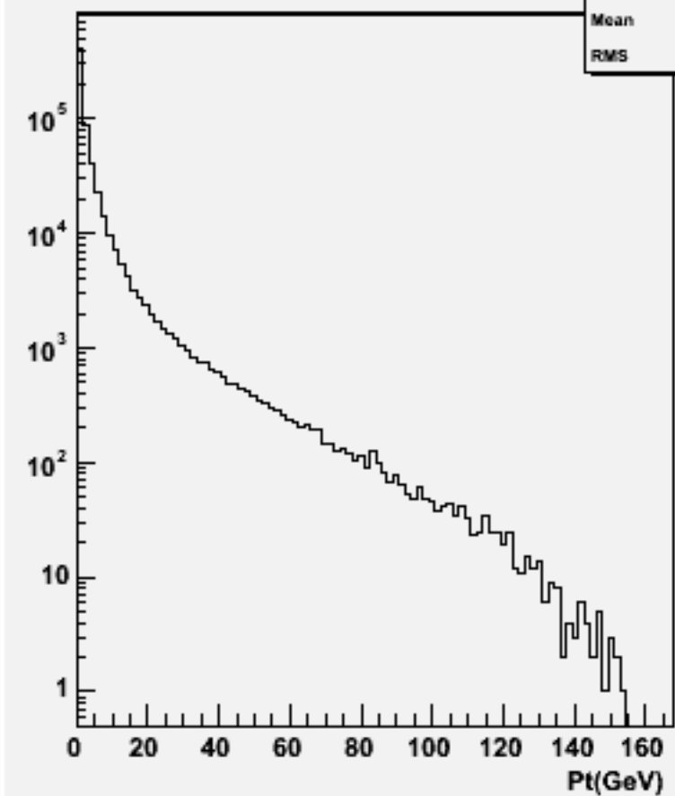
Particle Pt : w102573 e2e2e3e3bb_o
