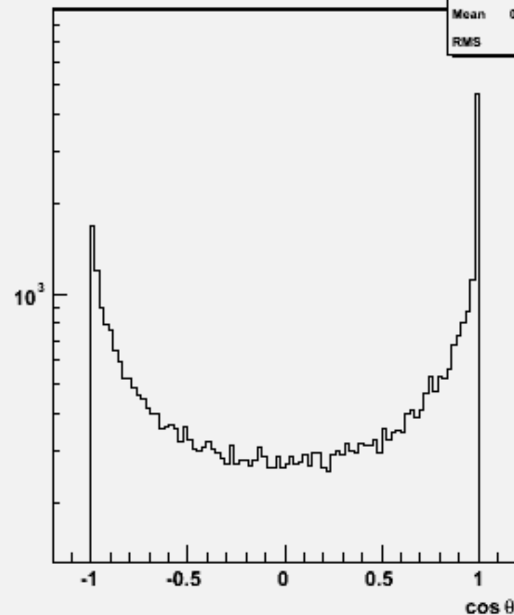
Jet cos \theta (All jets)w102573 e2e2e3e3bb_o
