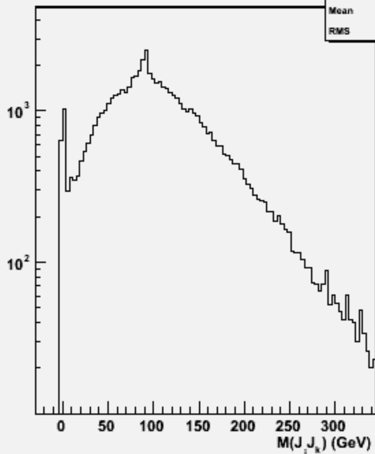
2jets mass(All comb)w102573 e2e2e3e3bb_o
