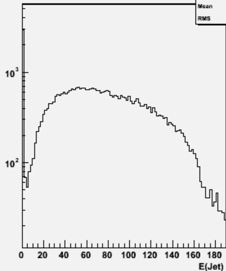
Jet energies(All jets)w102573 e2e2e3e3bb_o
