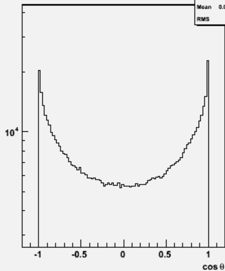
Particle cos \theta : w102573 e2e2e3e3bb_o
