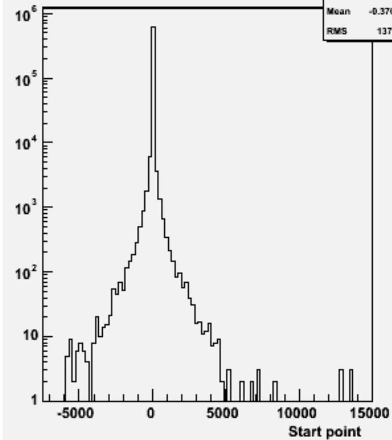
Start point Z : w102573 e2e2e3e3bb_o
