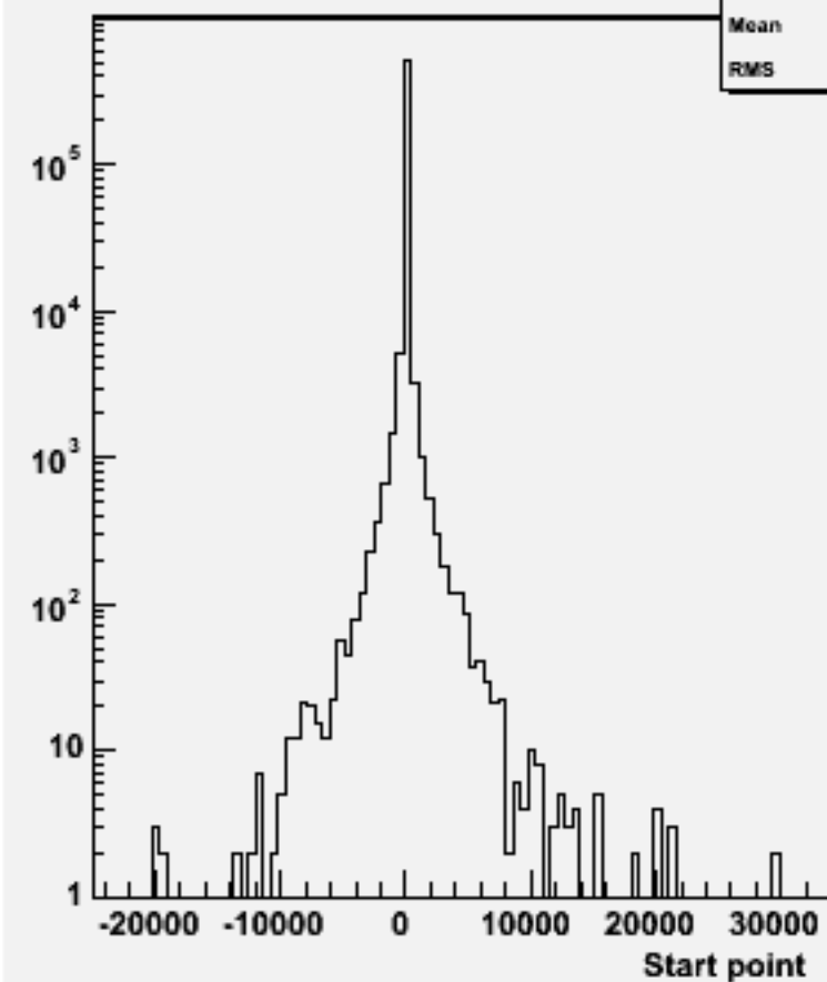
Start point Z : w102569 e2e2e3e3ss_o
