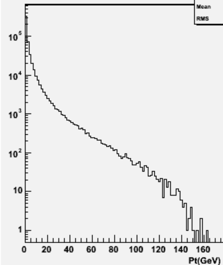
Particle Pt : w102569 e2e2e3e3ss_o
