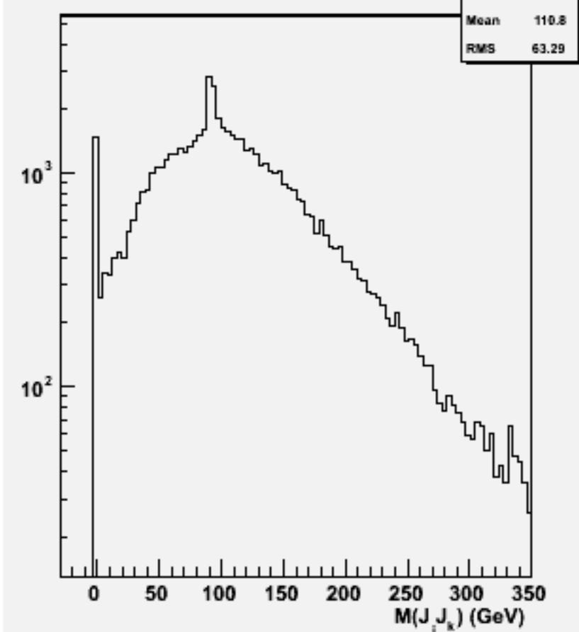
2jets mass(All comb)w102569 e2e2e3e3ss_o
