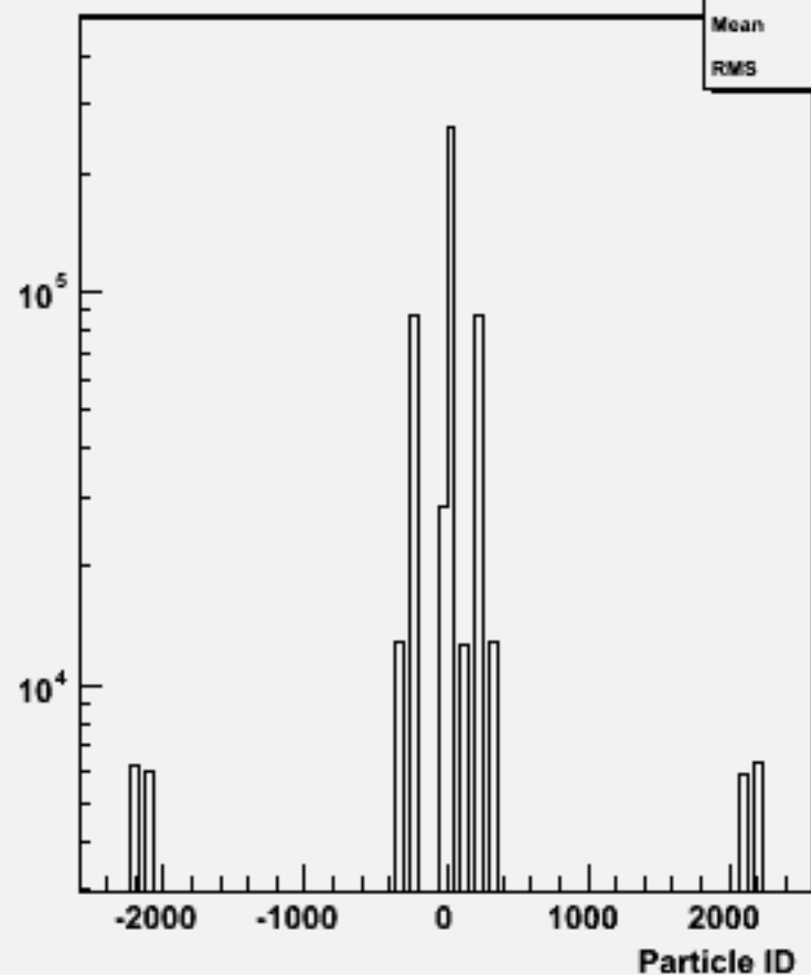
Particle ID : w102569 e2e2e3e3ss_o
