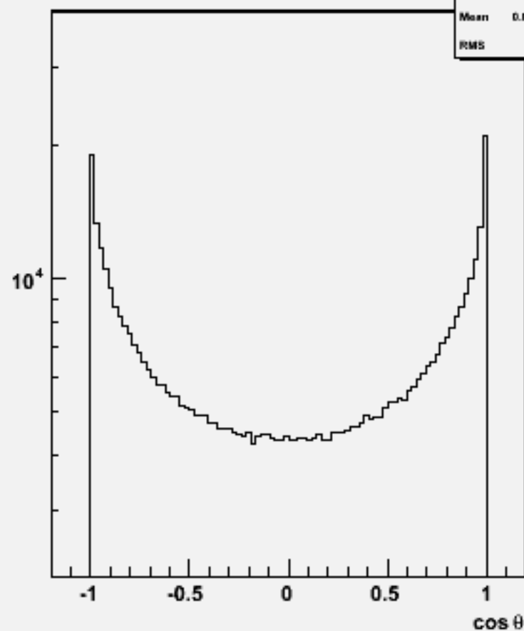
Particle cosθ : w102569 e2e2e3e3ss_o
