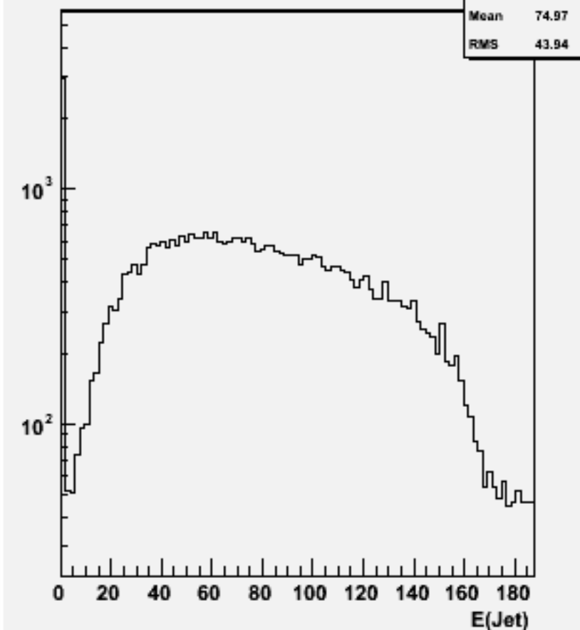
Jet energies(All jets)w102569 e2e2e3e3ss_o
