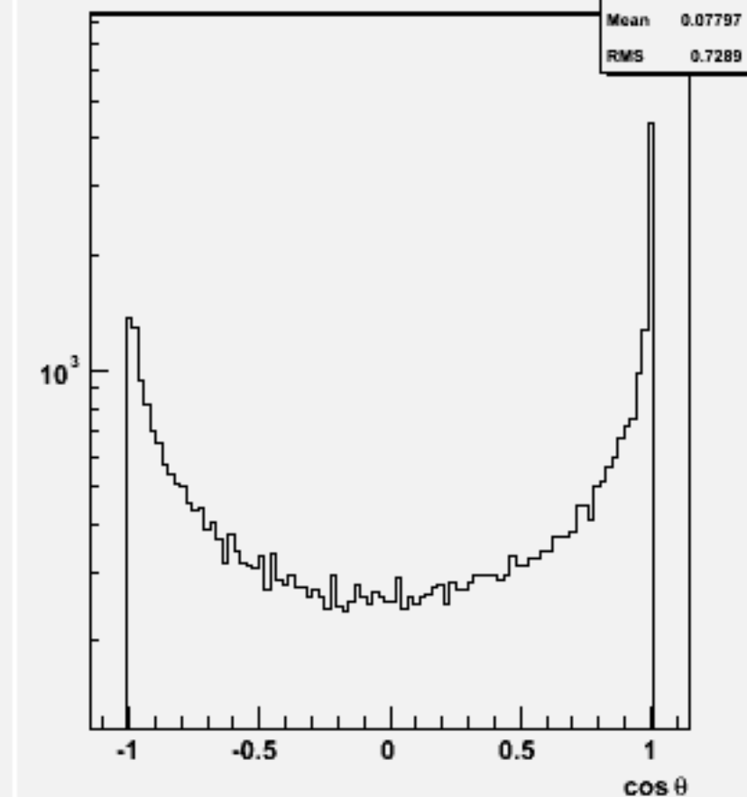
Jet cos \theta (All jets)w102569 e2e2e3e3ss_o
