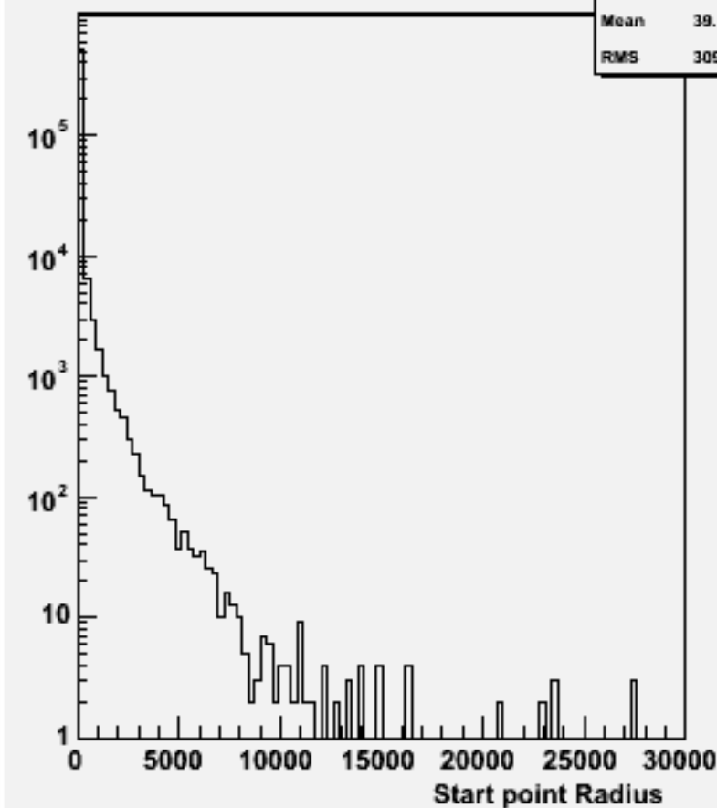
Start point R : w102569 e2e2e3e3ss_o
