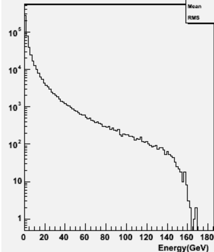
Particle Energy : w102569 e2e2e3e3ss_o
