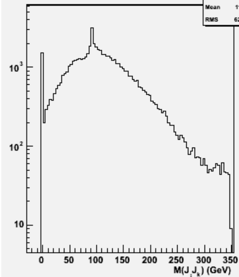
2jets mass(All comb)w102568 e2e2e3e3ss_o
