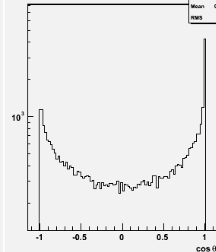
Jet cos \theta (All jets)w102568 e2e2e3e3ss_o
