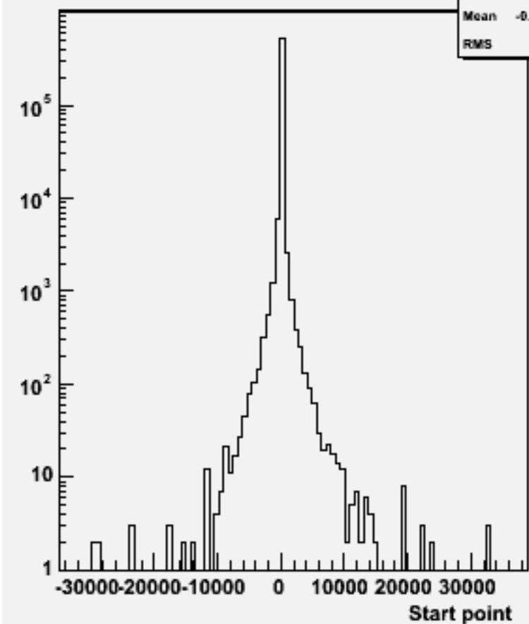
Start point Z : w102568 e2e2e3e3ss_o
