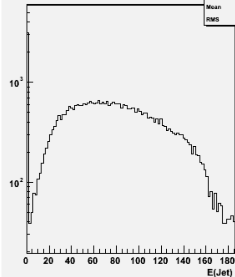
Jet energies(All jets)w102568 e2e2e3e3ss_o
