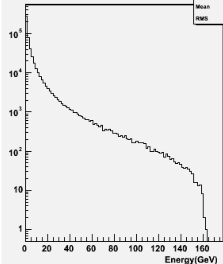
Start point R : w102568 e2e2e3e3ss_o
