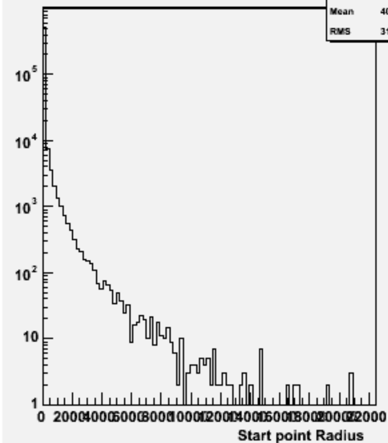
Start point R : w102568 e2e2e3e3ss_o
