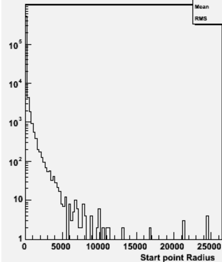
Start point R : w102565 e2e2e3e3dd_o
