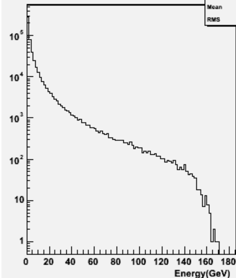
Particle Energy : w102565 e2e2e3e3dd_o
