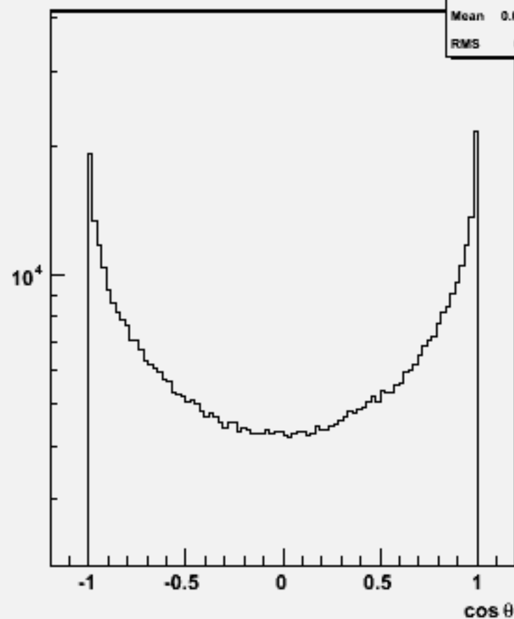
Particle cos \theta : w102565 e2e2e3e3dd_o
