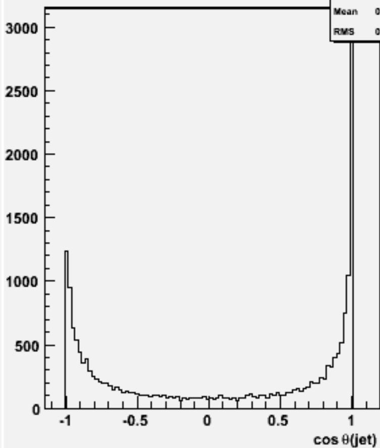
cos \theta for 2-jets :w102565 e2e2e3e3dd_o
