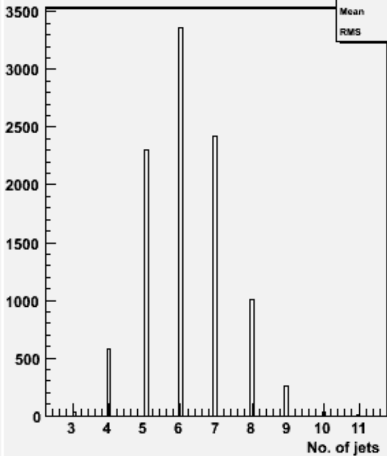
No. jets (ycut=0.001) : w102565 e2e2e3e3dd_o
