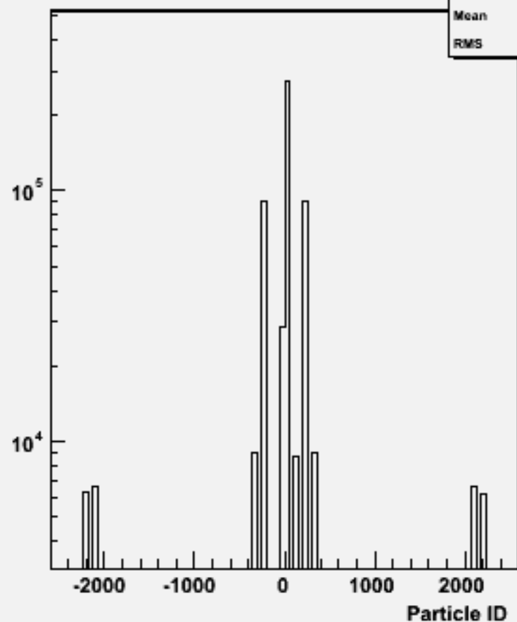
Particle ID : w102565 e2e2e3e3dd_o
