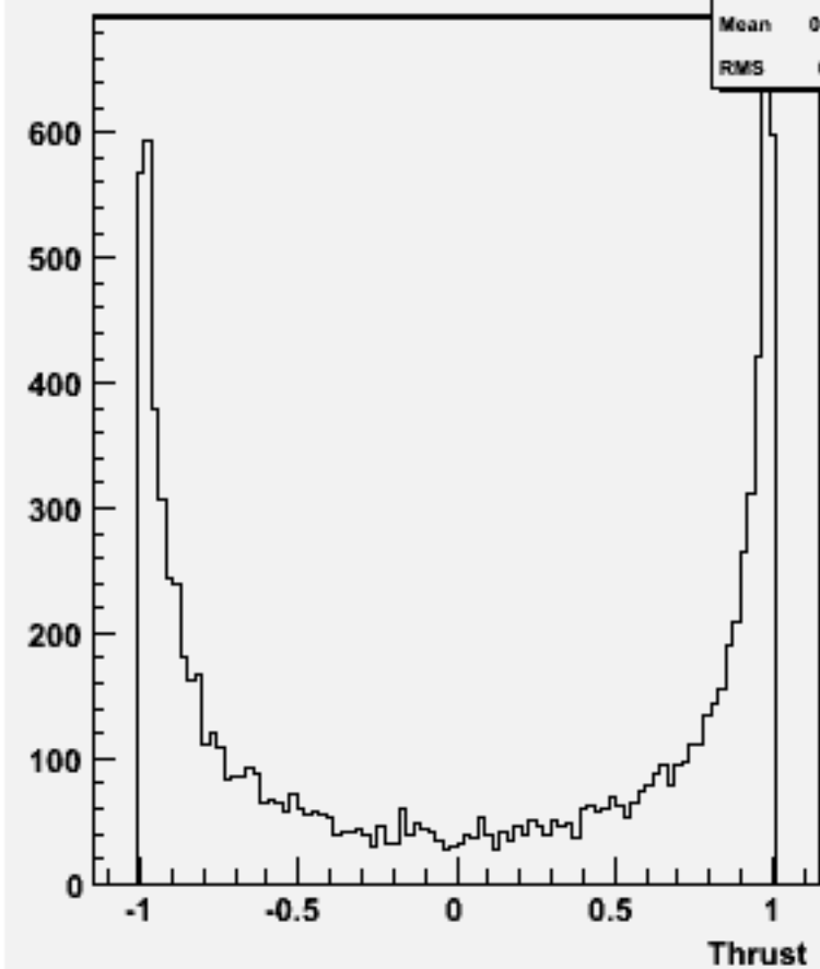
cos \Theta (thrust) w102565 e2e2e3e3dd_o
