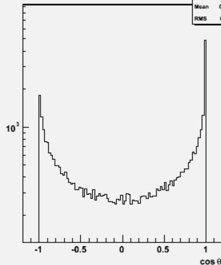
Jet cos \theta (All jets)w102565 e2e2e3e3dd_o
