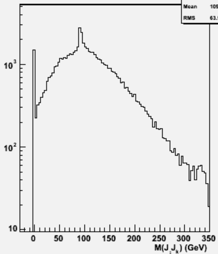
2jets mass(All comb)w102565 e2e2e3e3dd_o
