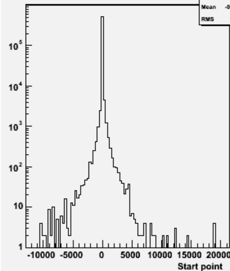
Start point Z : w102565 e2e2e3e3dd_o
