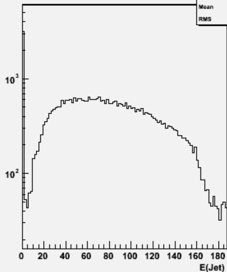
Jet energies(All jets)w102565 e2e2e3e3dd_o
