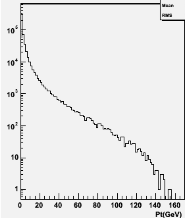
Particle Pt : w102565 e2e2e3e3dd_o
