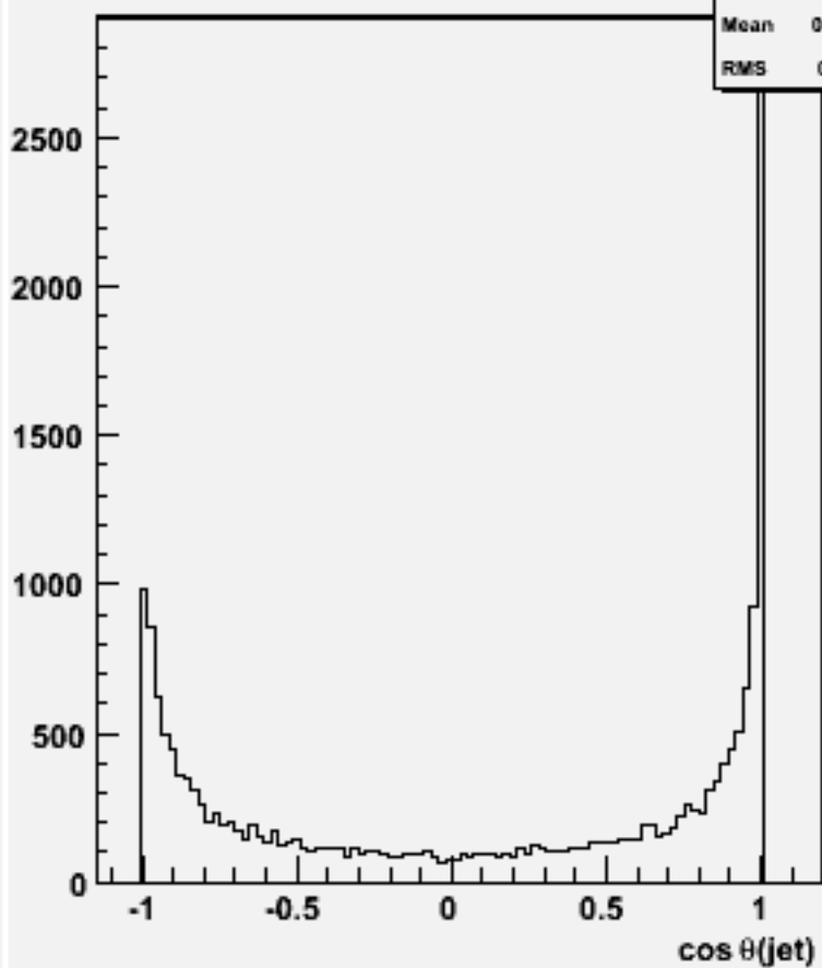
cos \theta for 2-jets :w102564 e2e2e3e3dd_o
