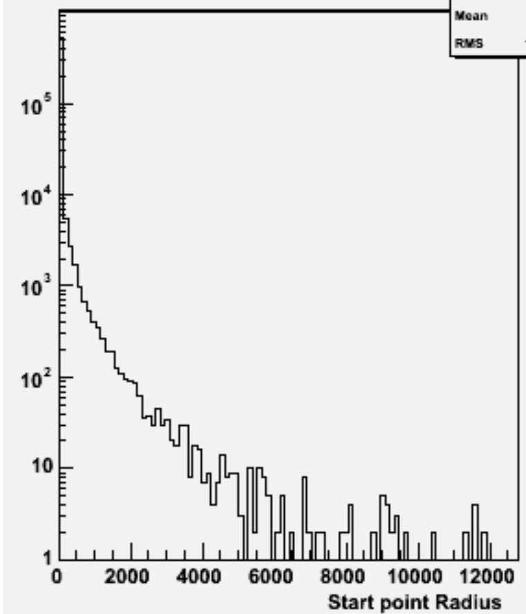
Start point R : w102564 e2e2e3e3dd_o
