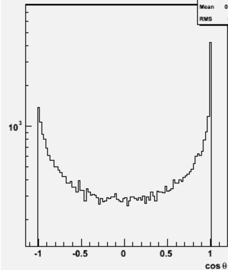
Jet cos \theta (All jets)w102564 e2e2e3e3dd_o
