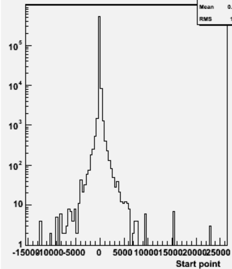
Start point Z : w102564 e2e2e3e3dd_o
