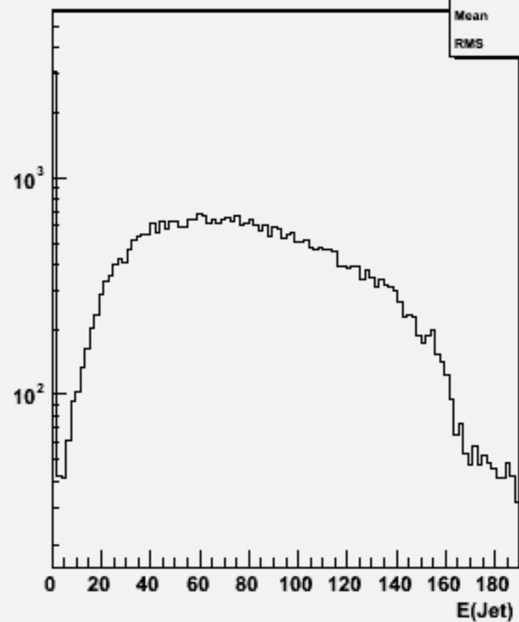
Jet energies(All jets)w102564 e2e2e3e3dd_o
