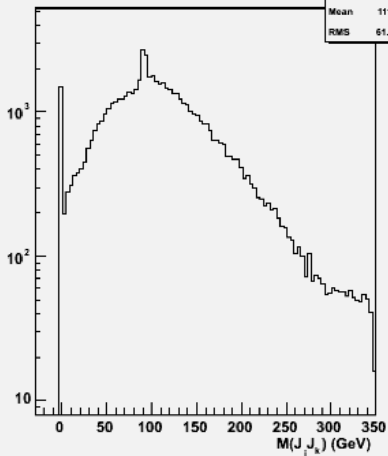
2jets mass(All comb)w102564 e2e2e3e3dd_o
