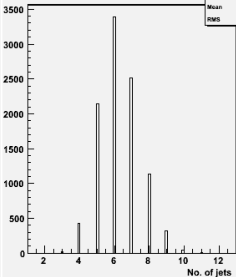
No. jets (ycut=0.001) : w102564 e2e2e3e3dd_o
