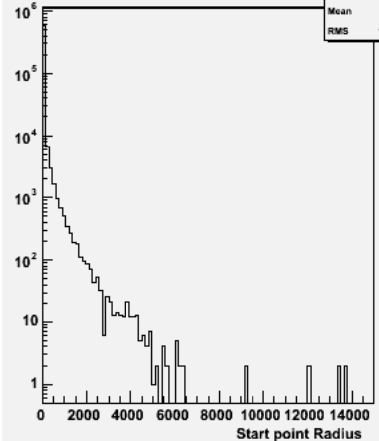
Start point R : w102557 e2e2e2e2bb_o
