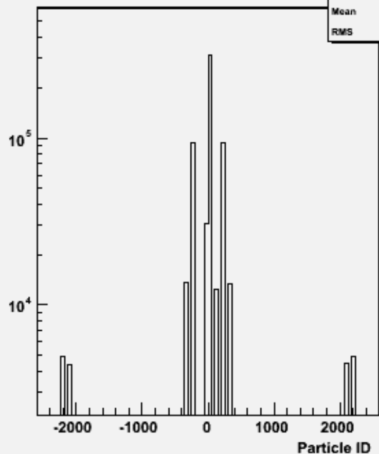
Particle ID : w102557 e2e2e2e2bb_o
