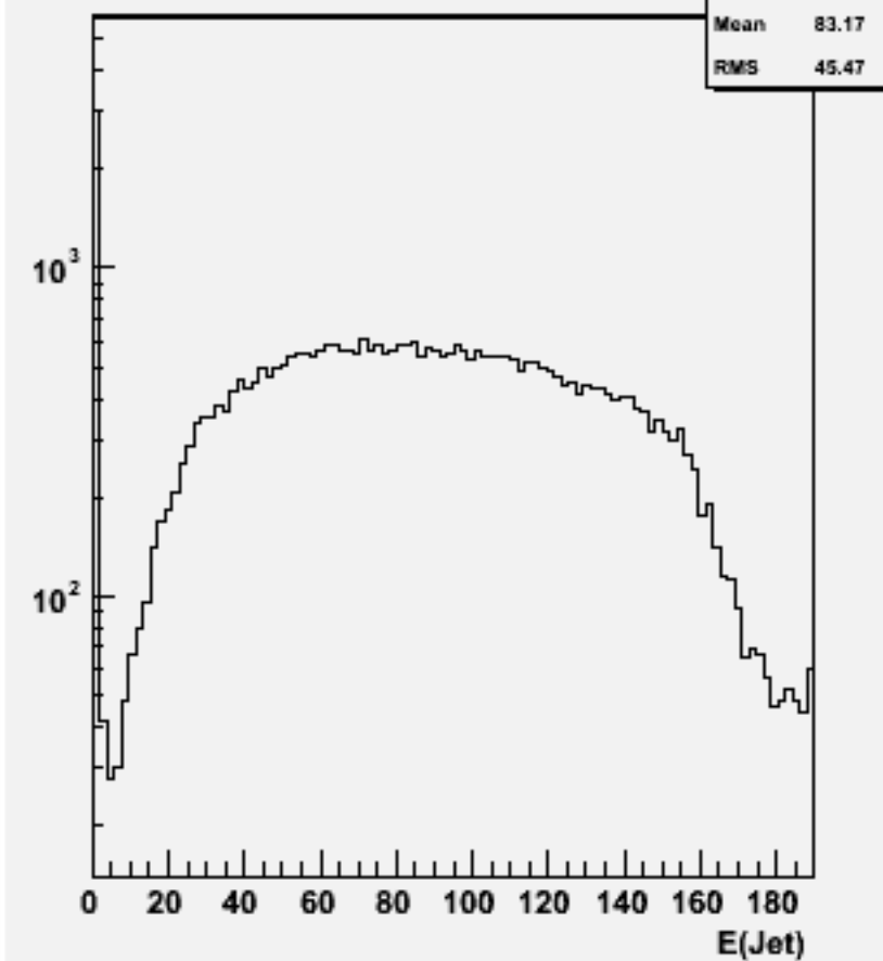
Jet energies(All jets)w102557 e2e2e2e2bb_o
