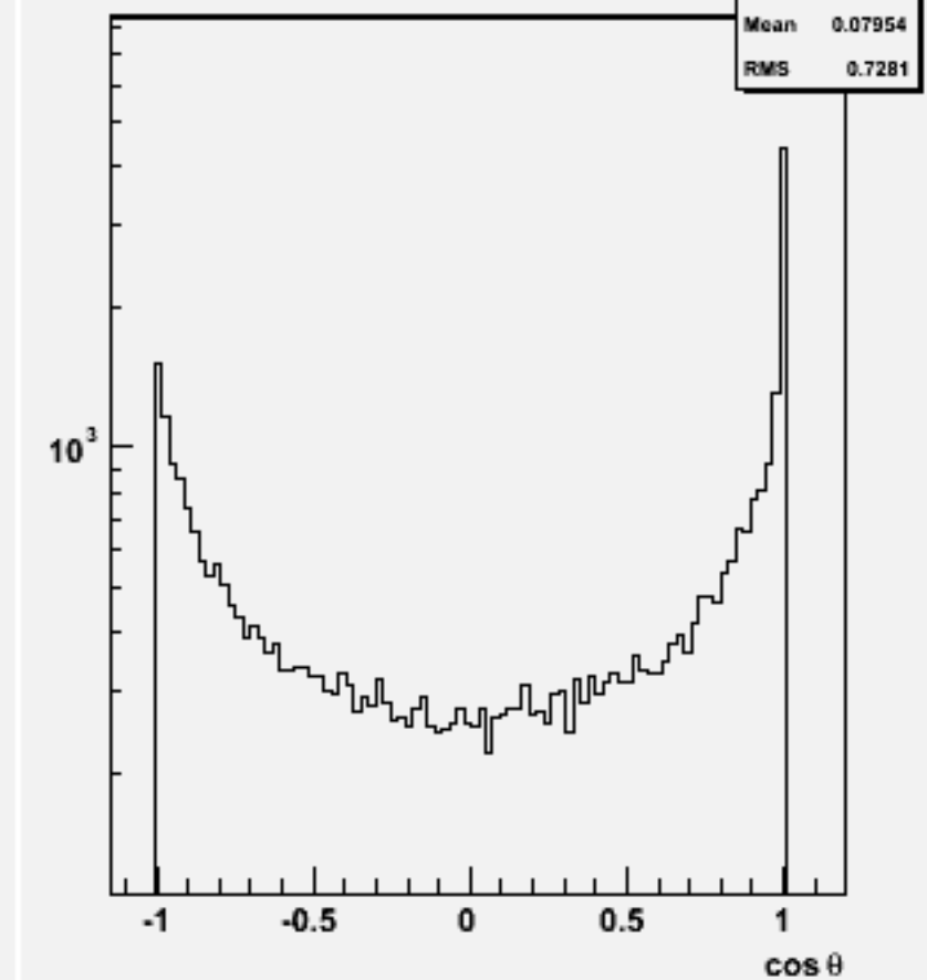
Jet cos \theta (All jets)w102557 e2e2e2e2bb_o
