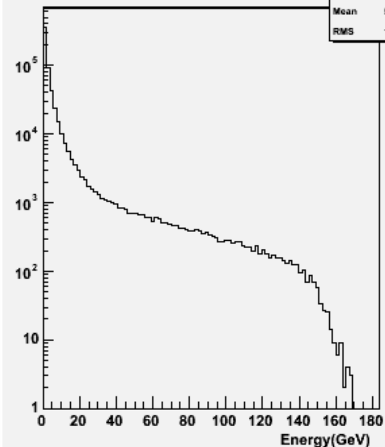
Particle Energy : w102557 e2e2e2e2bb_o
