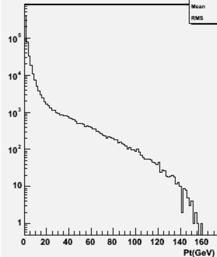
Particle Pt : w102557 e2e2e2e2bb_o
