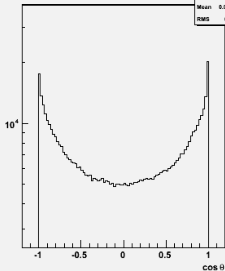
Particle cos \theta : w102557 e2e2e2e2bb_o
