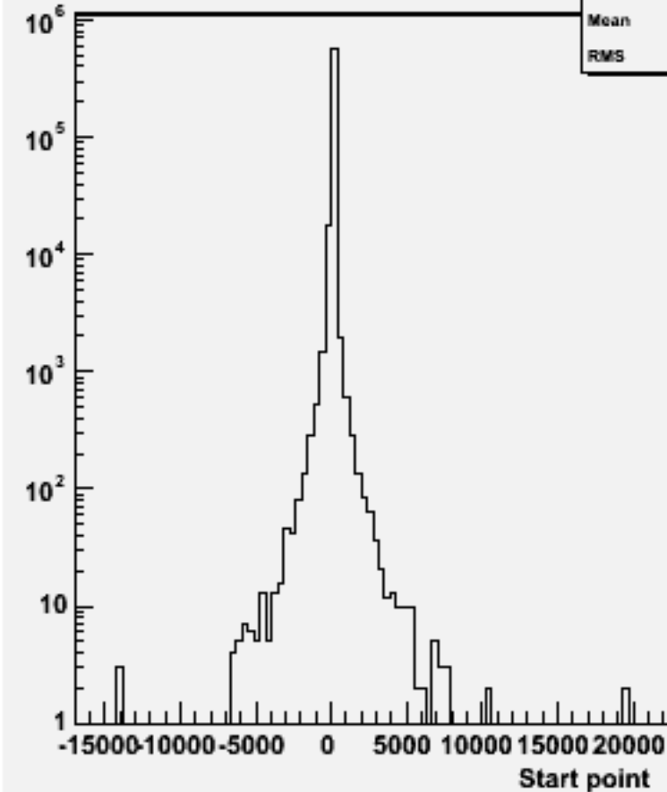
Start point Z : w102557 e2e2e2e2bb_o
