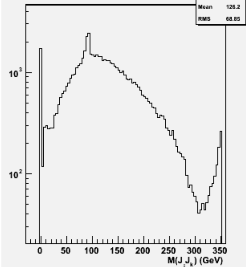
2jets mass(All comb)w102557 e2e2e2e2bb_o
