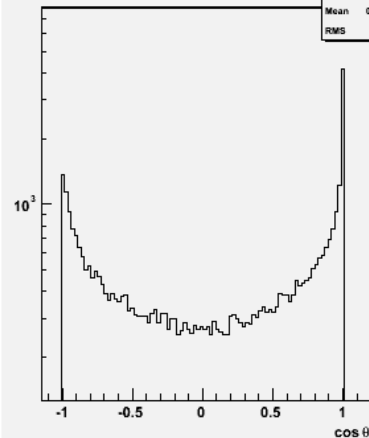
Jet cos \theta (All jets)w102556 e2e2e2e2bb_o
