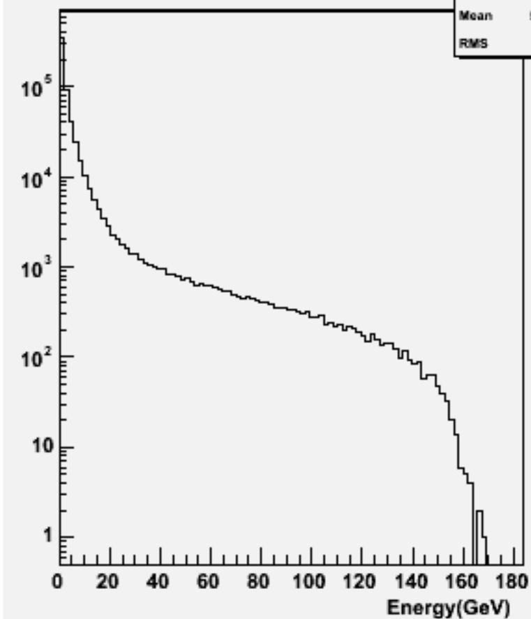
Particle Energy : w102556 e2e2e2e2bb_o
