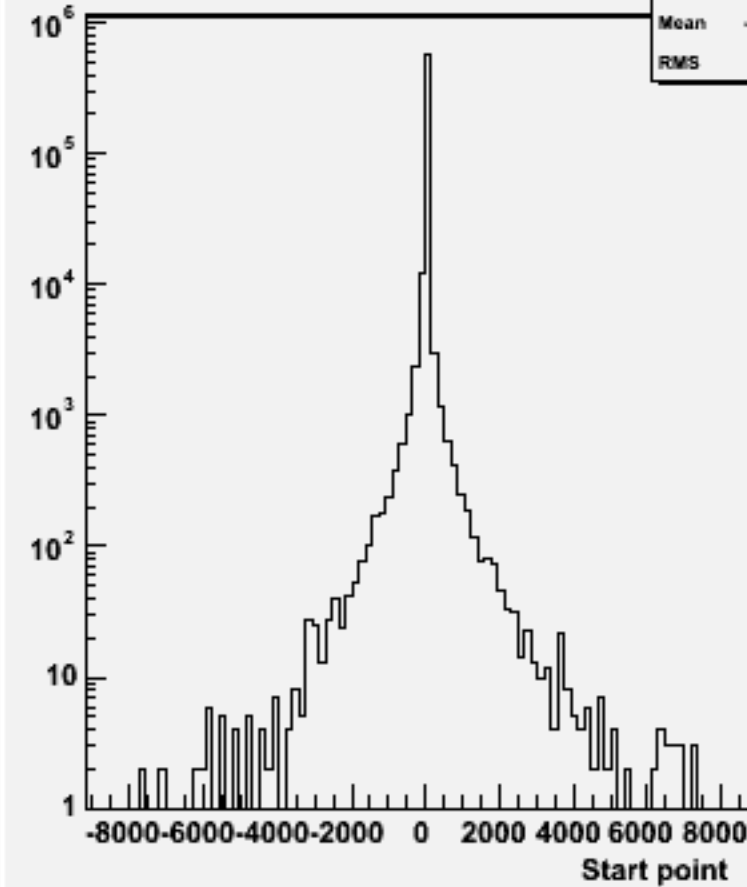
Start point Z : w102556 e2e2e2e2bb_o
