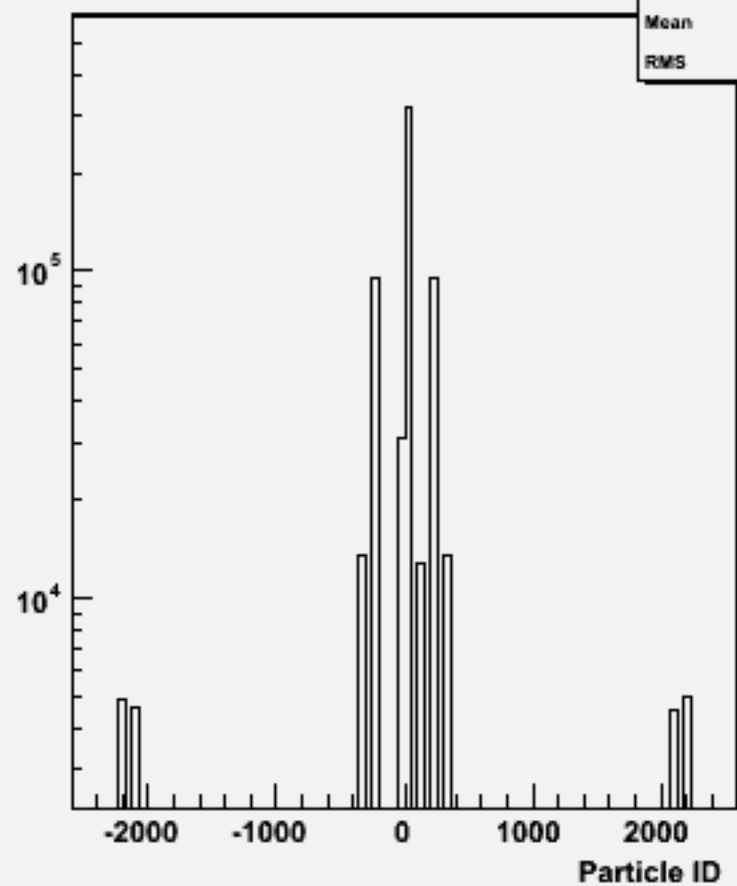
Particle ID : w102556 e2e2e2e2bb_o
