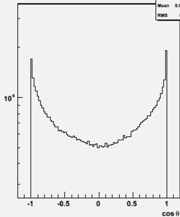
Particle cos \theta : w102556 e2e2e2e2bb_o
