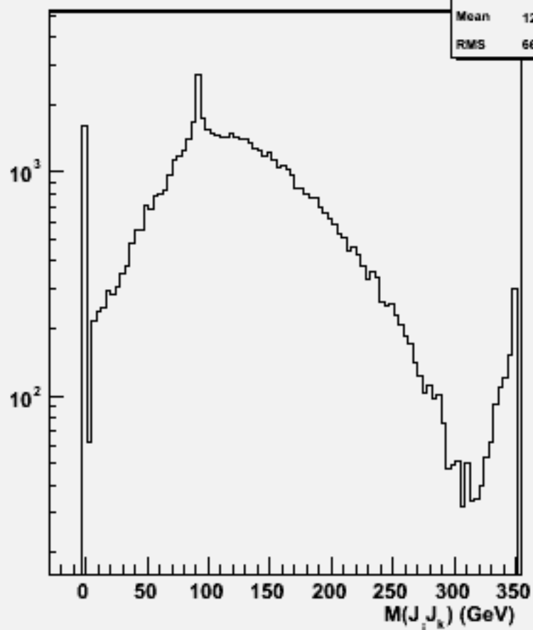
2jets mass(All comb)w102556 e2e2e2e2bb_o
