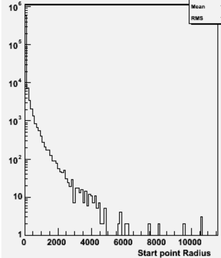
Start point R : w102556 e2e2e2e2bb_o
