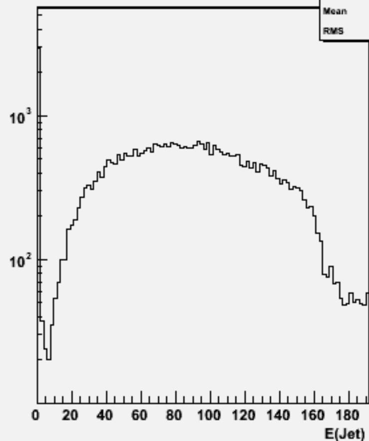
Jet energies(All jets)w102556 e2e2e2e2bb_o
