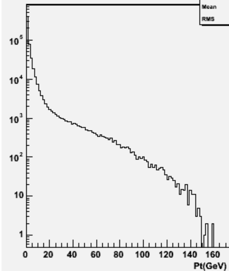
Particle Pt : w102556 e2e2e2e2bb_o
