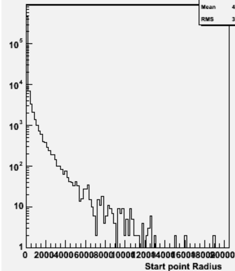
Start point R : w102552 e2e2e2e2ss_o
