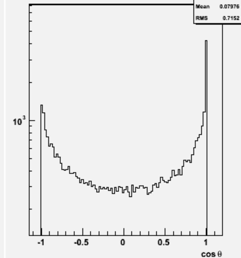
Jet cos \theta (All jets)w102552 e2e2e2e2ss_o
