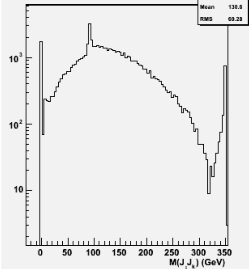
2jets mass(All comb)w102552 e2e2e2e2ss_o
