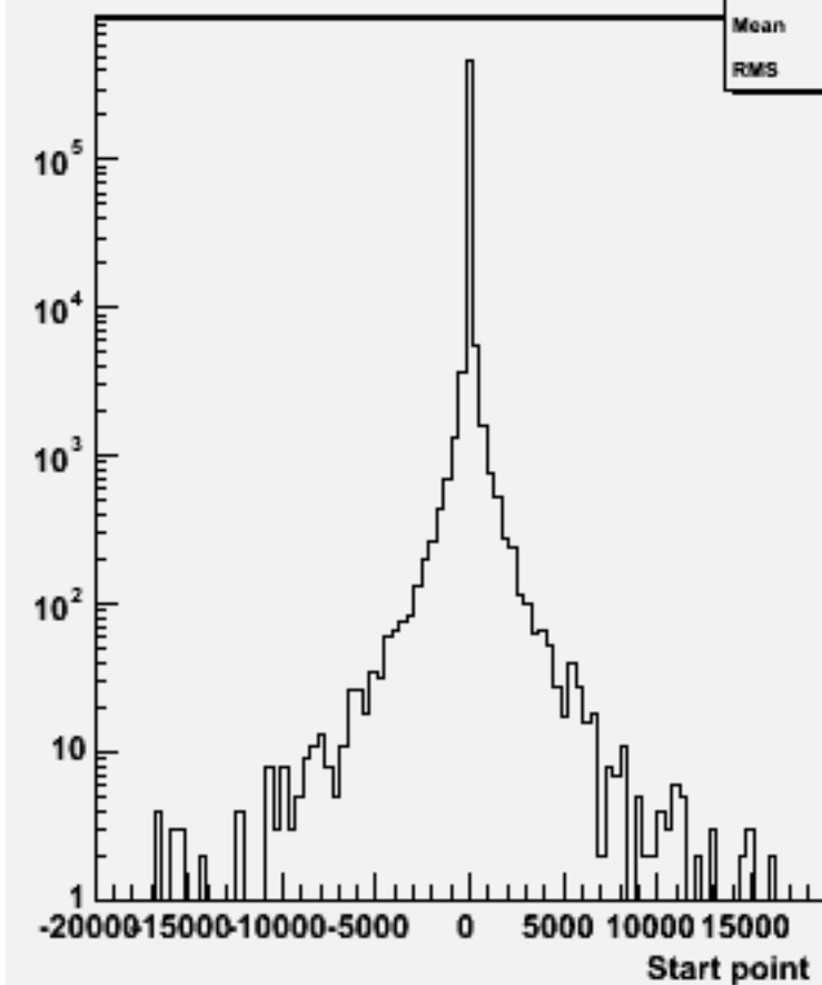
Start point Z : w102552 e2e2e2e2ss_o
