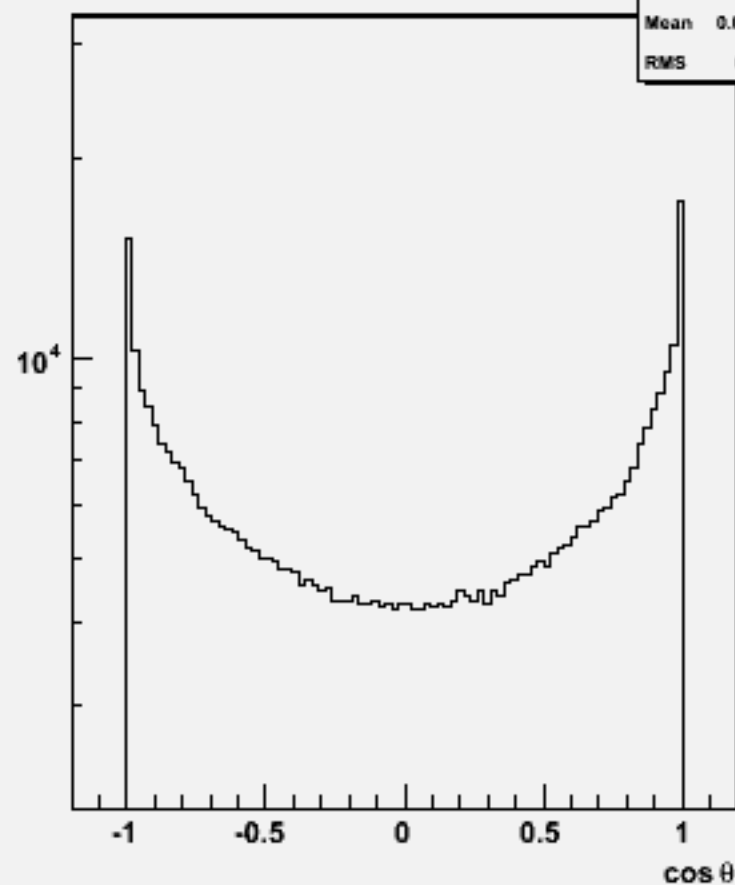
Particle cosθ : w102552 e2e2e2e2ss_o
