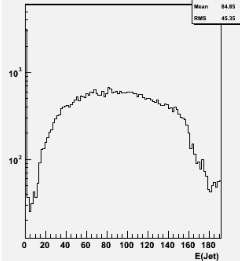
Jet energies(All jets)w102552 e2e2e2e2ss_o
