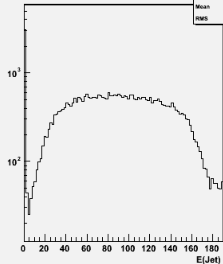
Jet energies(All jets)w102549 e2e2e2e2dd_o
