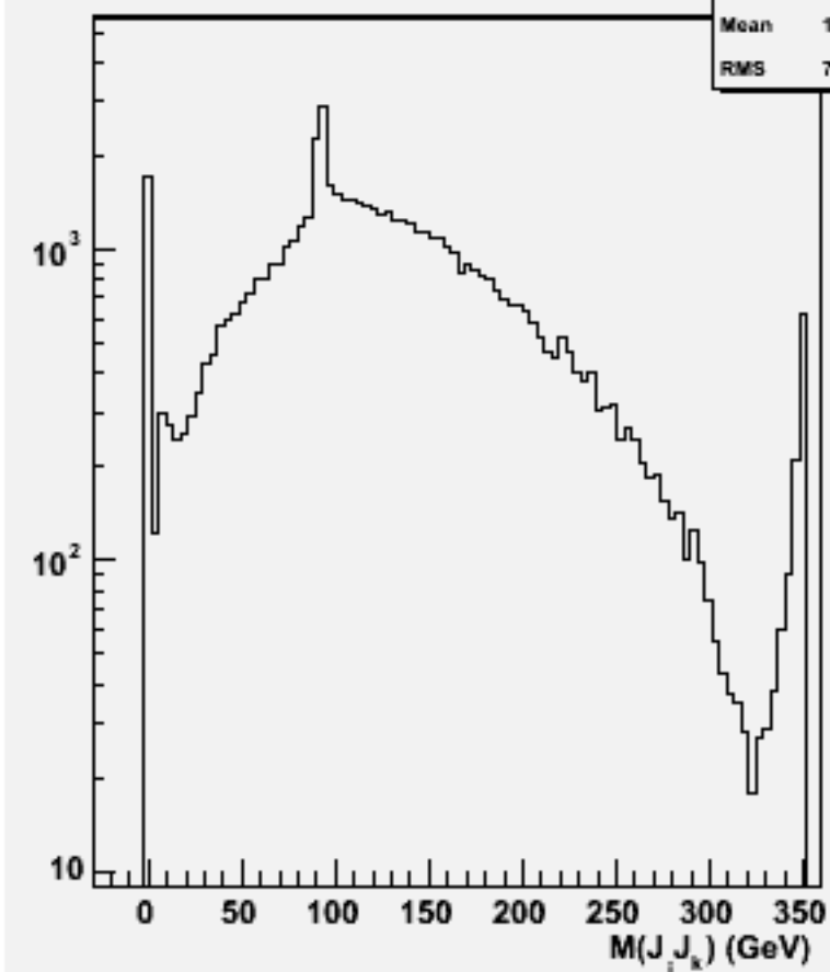
2jets mass(All comb)w102549 e2e2e2e2dd_o
