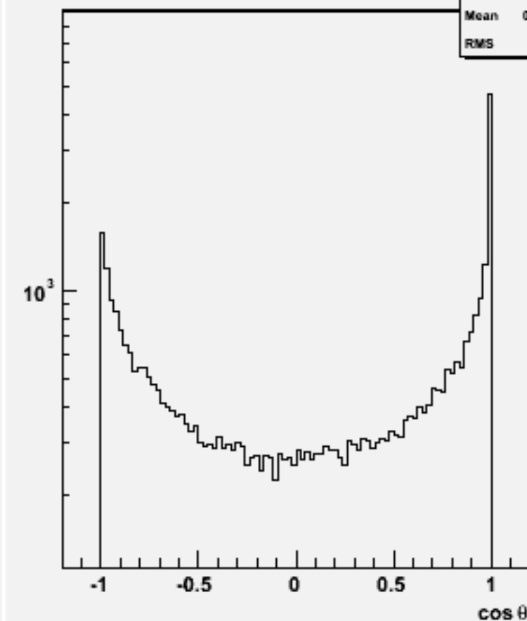
Jet cos \theta (All jets)w102549 e2e2e2e2dd_o
