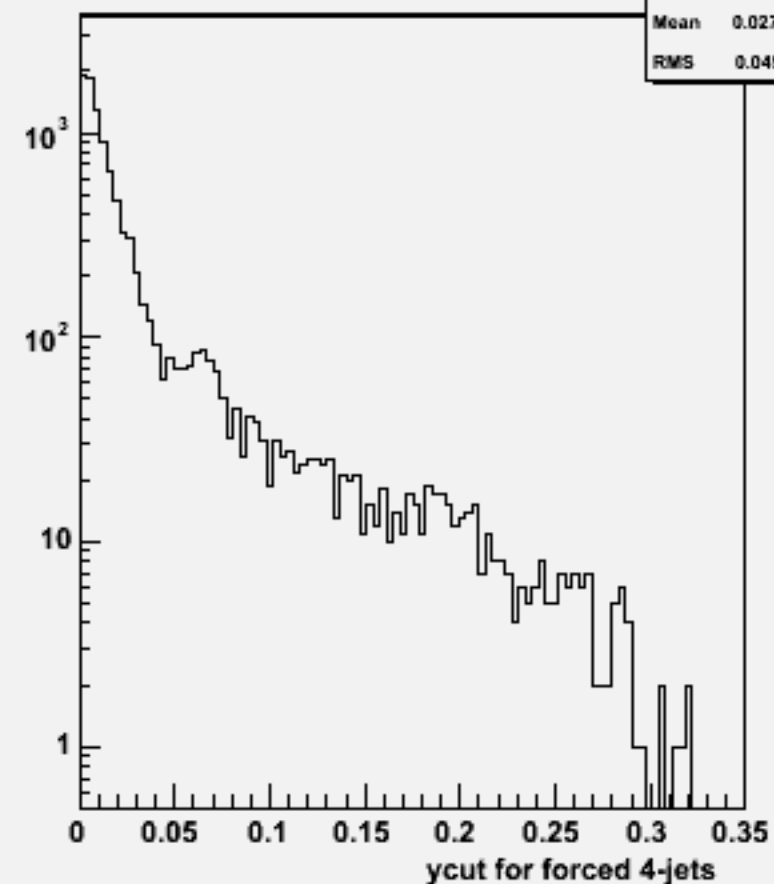
Ycut for 4-jets :w102549 e2e2e2e2dd_o
