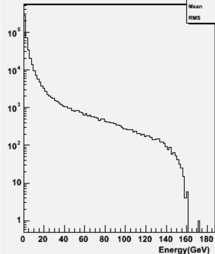
Particle Energy : w102548 e2e2e2e2dd_o
