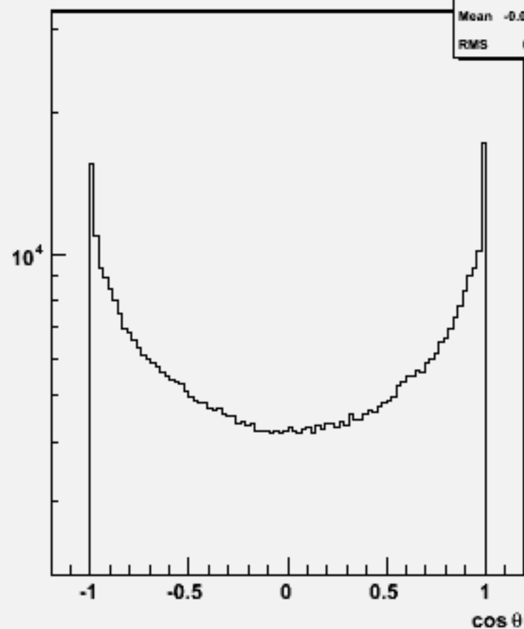
Particle cos \theta : w102548 e2e2e2e2dd_o
