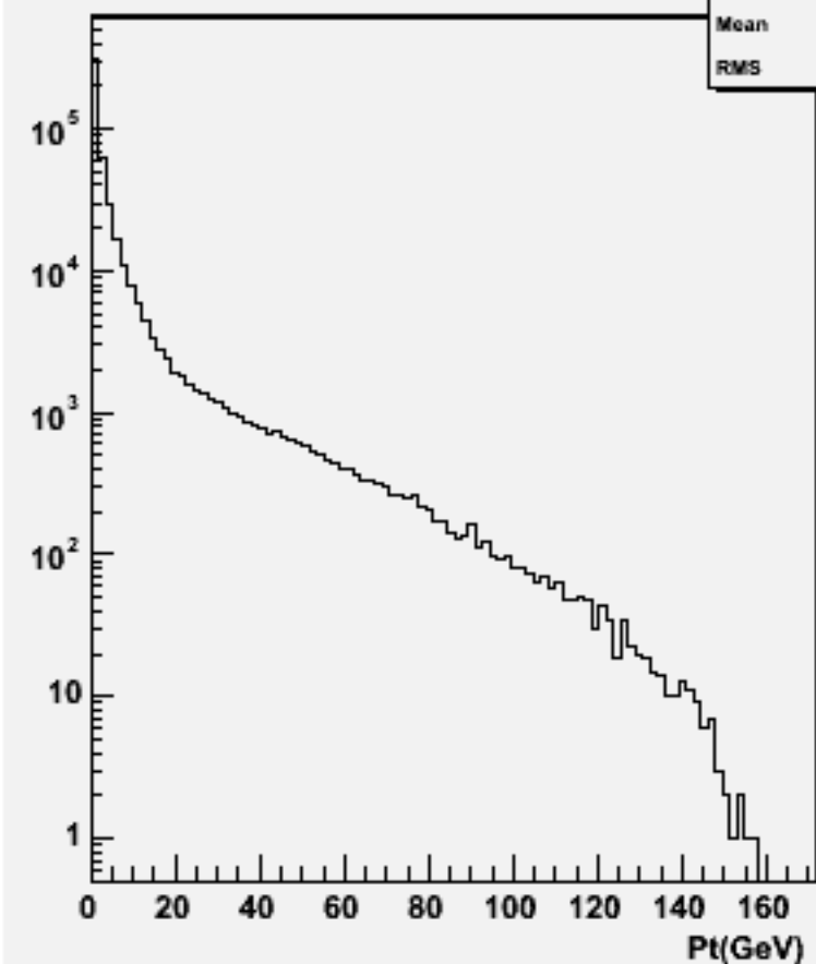
Particle Pt : w102548 e2e2e2e2dd_o
