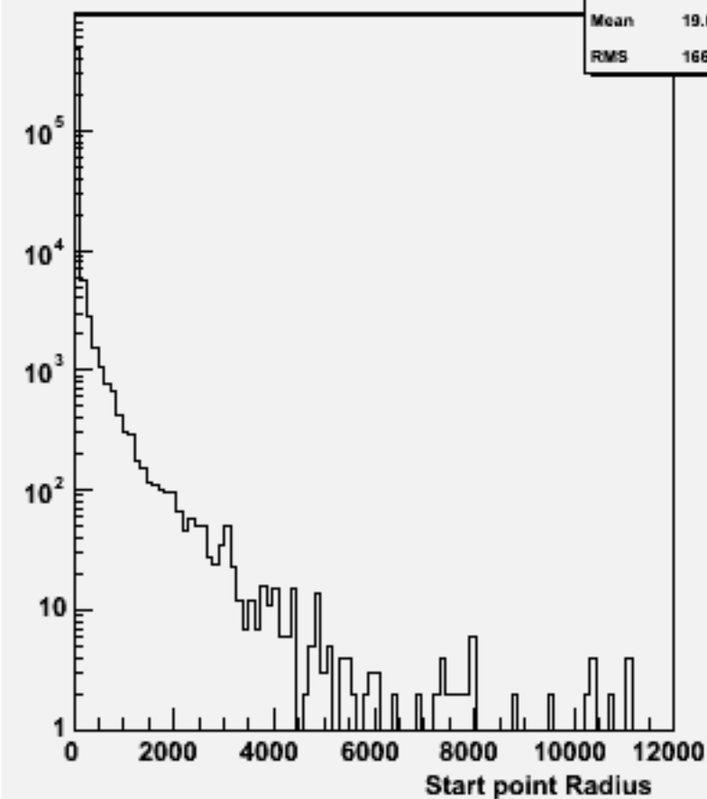
Start point R : w102548 e2e2e2e2dd_o
