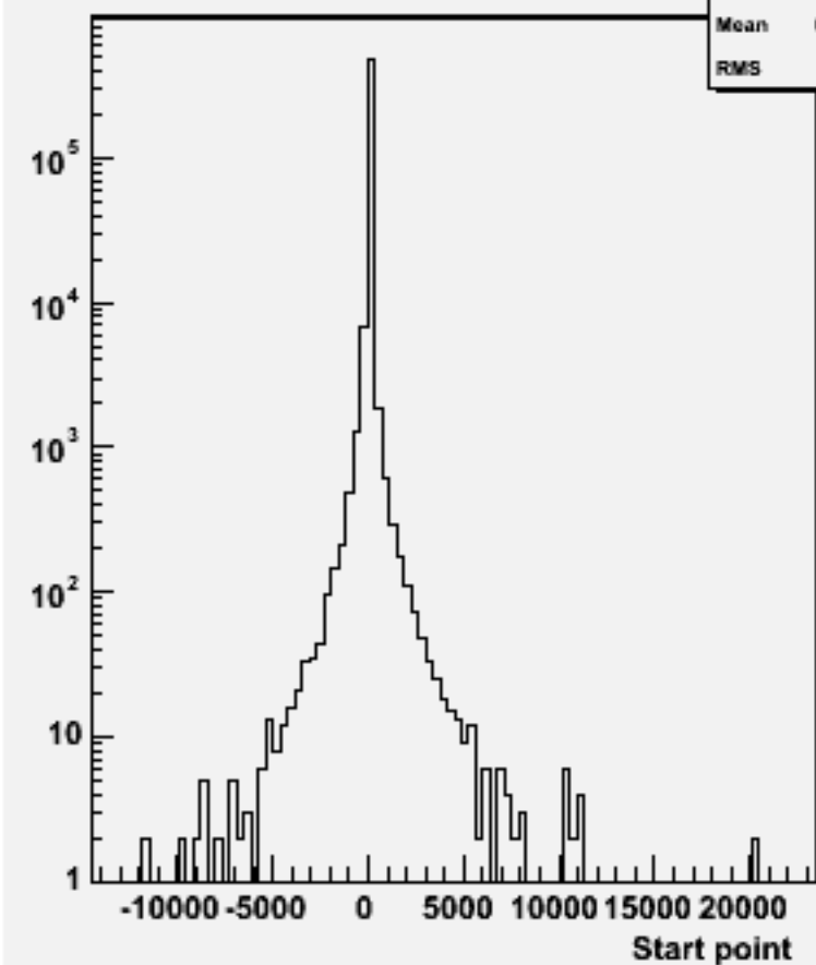
Start point Z : w102548 e2e2e2e2dd_o
