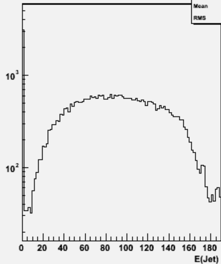
Jet energies(All jets)w102548 e2e2e2e2dd_o
