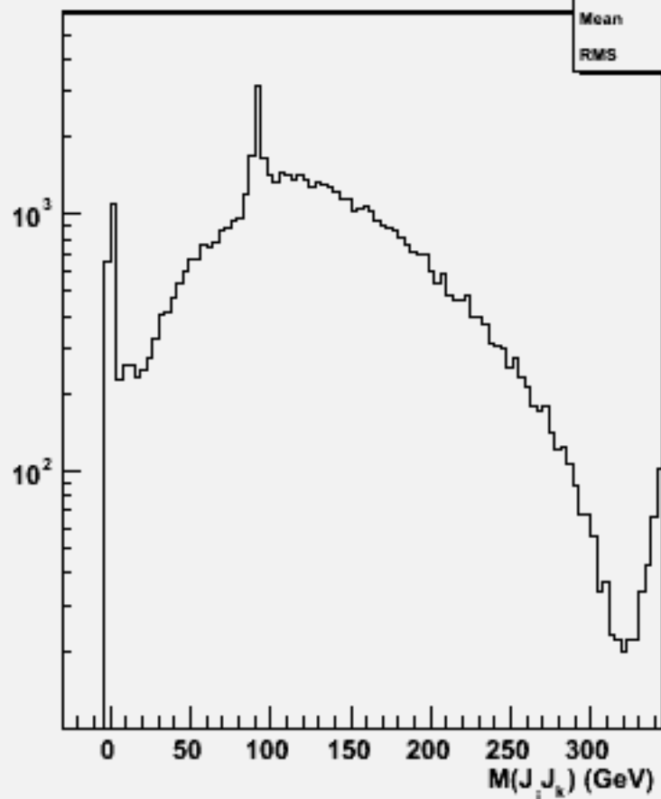
2jets mass(All comb)w102548 e2e2e2e2dd_o
