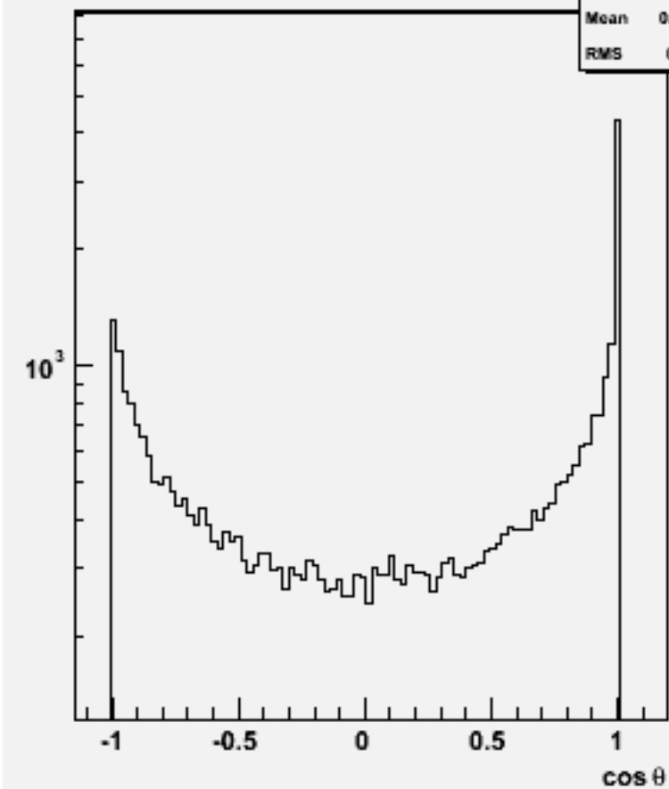
Jet cos \theta (All jets)w102548 e2e2e2e2dd_o
