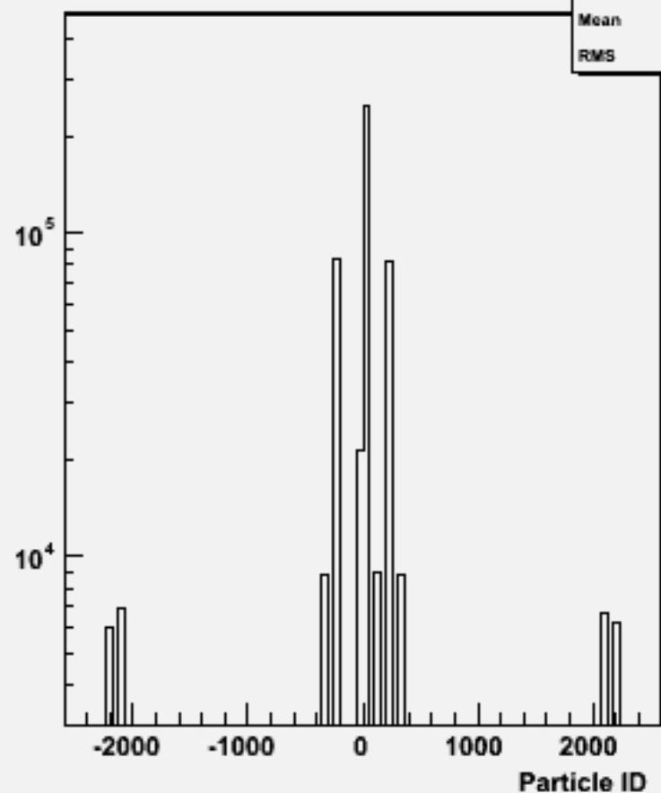
Particle ID : w102548 e2e2e2e2dd_o
