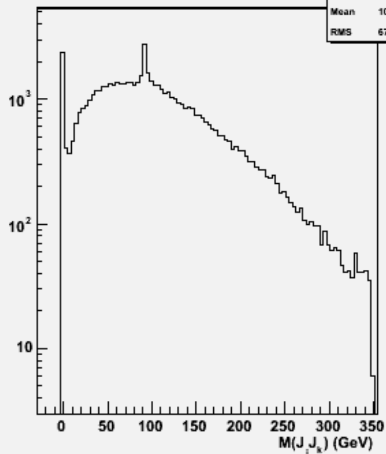
2jets mass(All comb)w102545 e2e2e2e2e3e3_o
