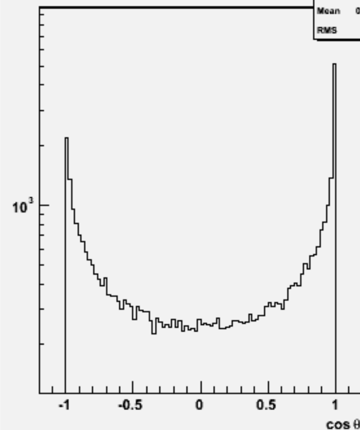
Jet cos \theta (All jets)w102545 e2e2e2e2e3e3_o
