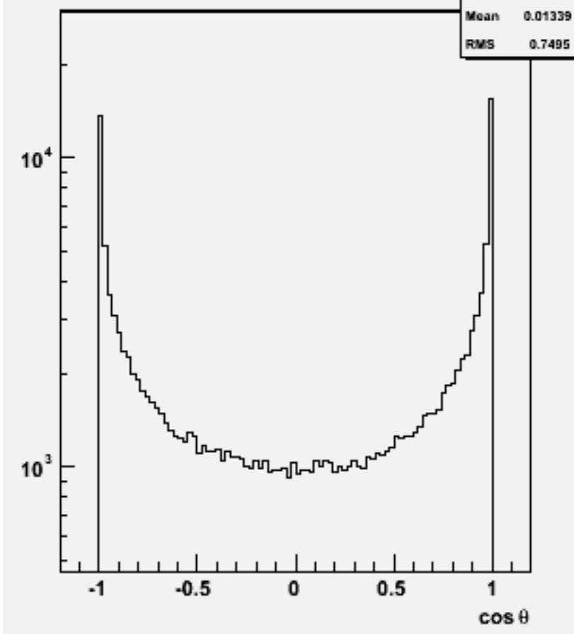
Particle cos \theta : w102545 e2e2e2e2e3e3_o
