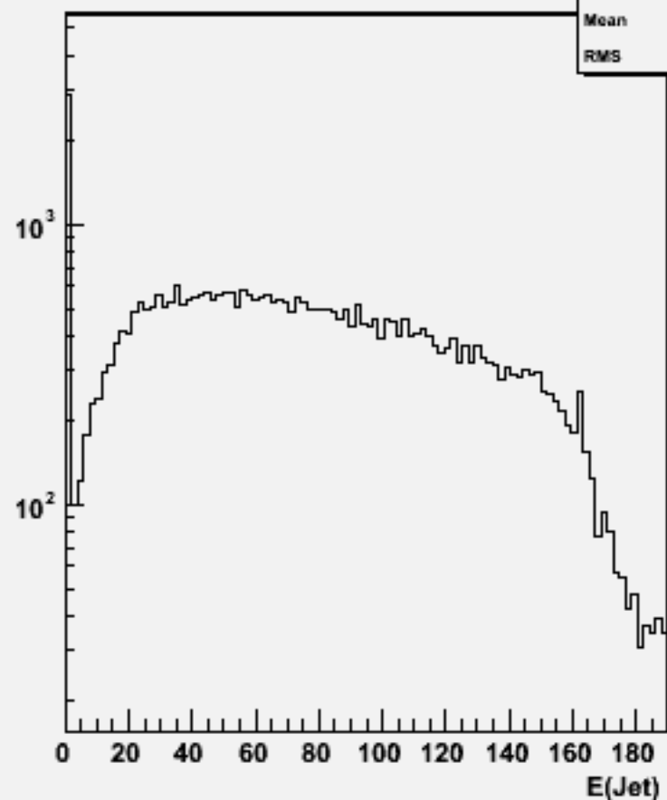
Jet energies(All jets)w102545 e2e2e2e2e3e3_o
