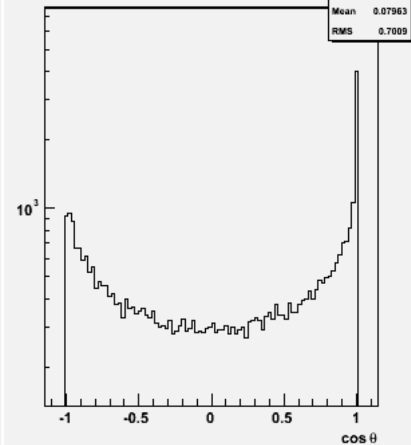
Jet cos \theta (All jets)w102537 e1e1bbbb_o
