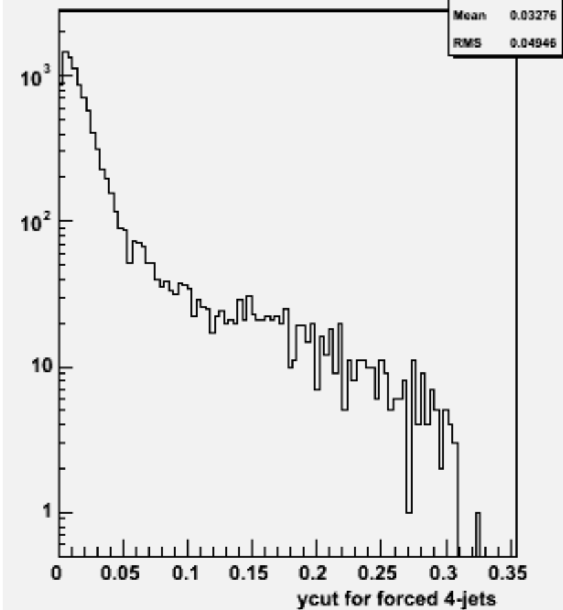
Ycut for 4-jets :w102537 e1e1bbbb_o
