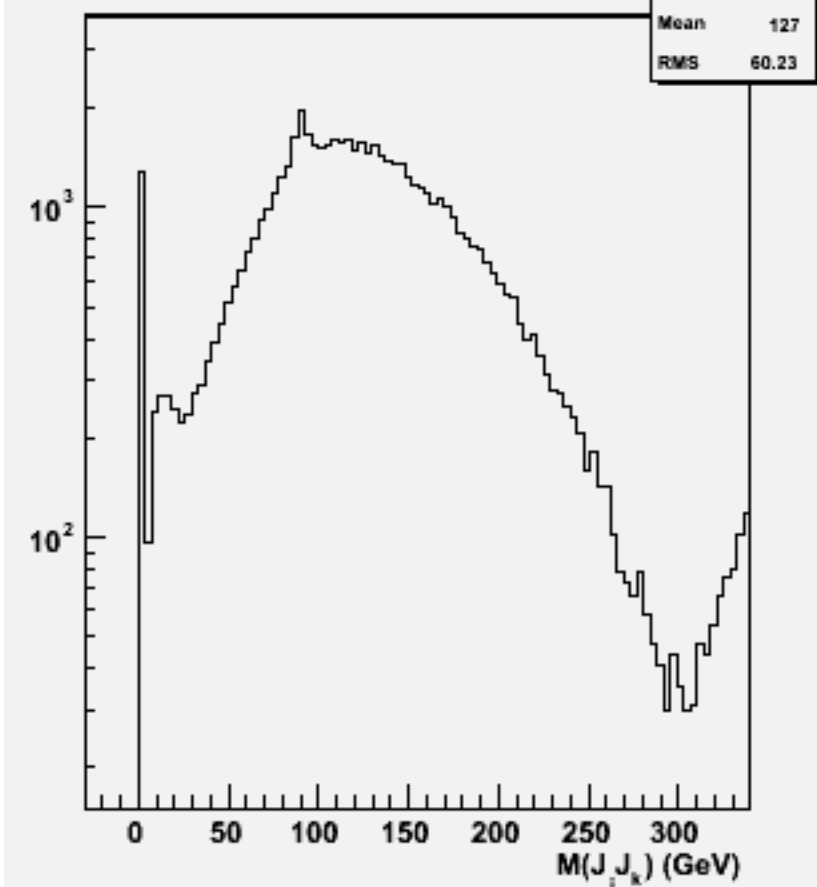
2jets mass(All comb)w102537 e1e1bbbb_o
