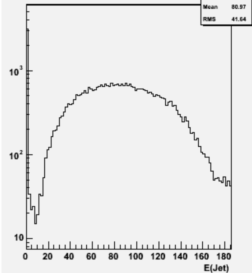
Jet energies(All jets)w102537 e1e1bbbb_o
