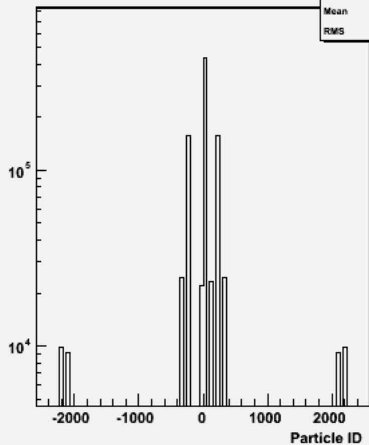
Particle ID : w102534 e1e1ssbb_o
