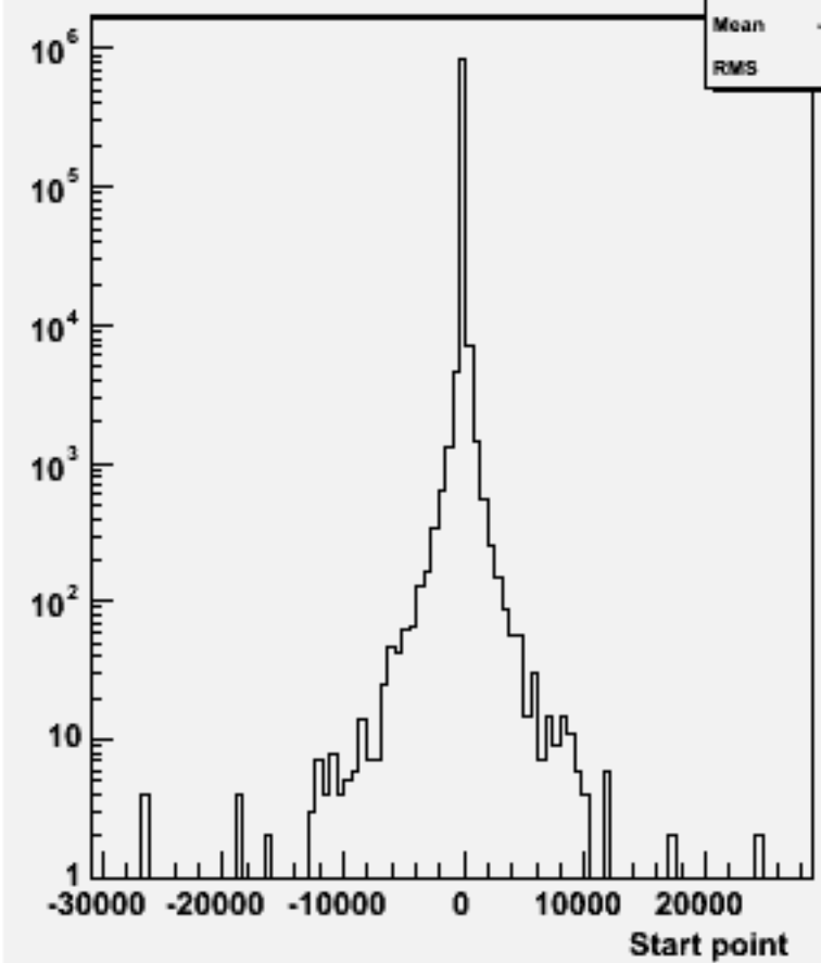
Start point Z : w102534 e1e1ssbb_o
