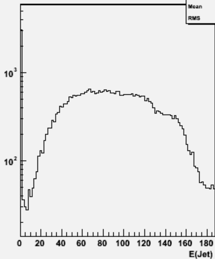
Jet energies(All jets)w102534 e1e1ssbb_o
