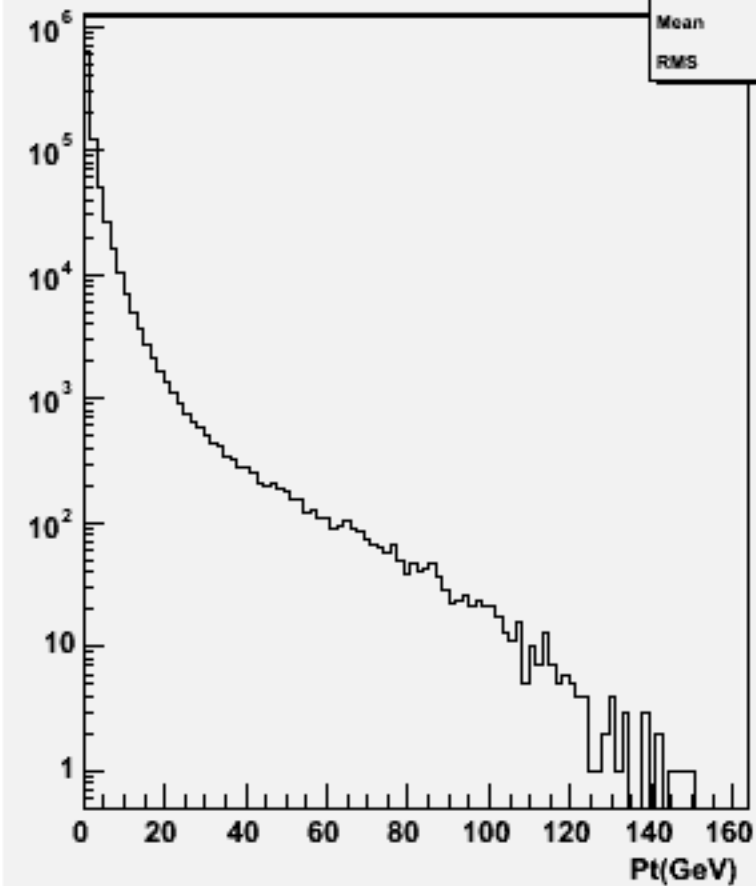
Particle Pt : w102534 e1e1ssbb_o
