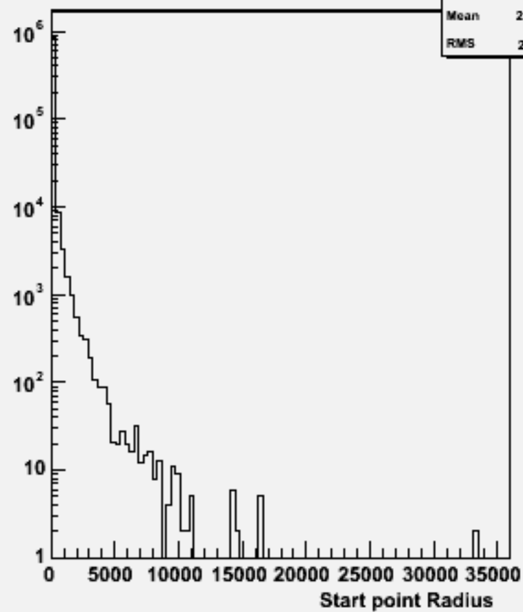
Start point R : w102534 e1e1ssbb_o
