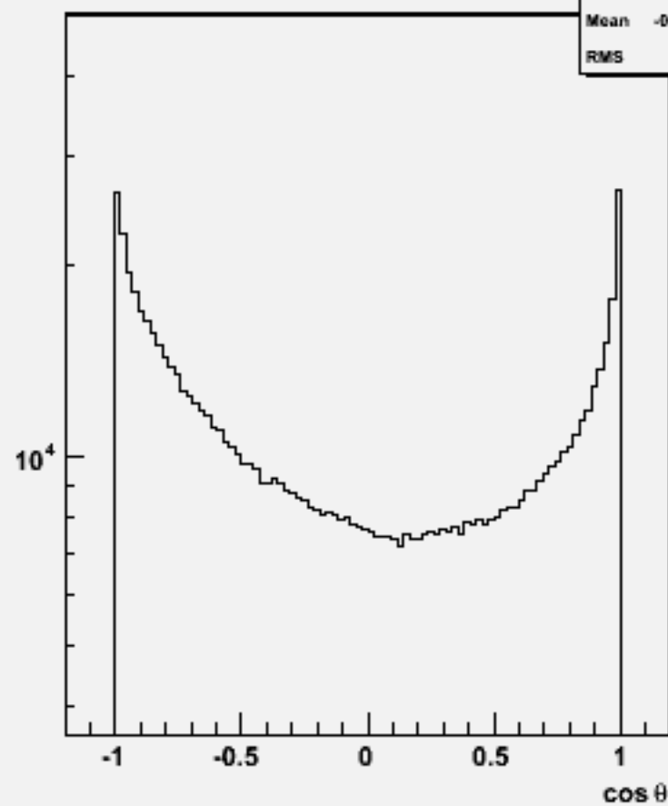
Particle cos \theta : w102534 e1e1ssbb_o
