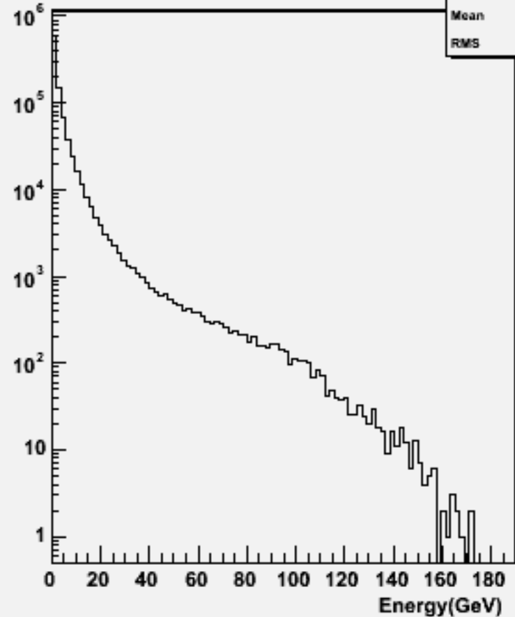
Particle Energy : w102533 e1e1ssbb_o
