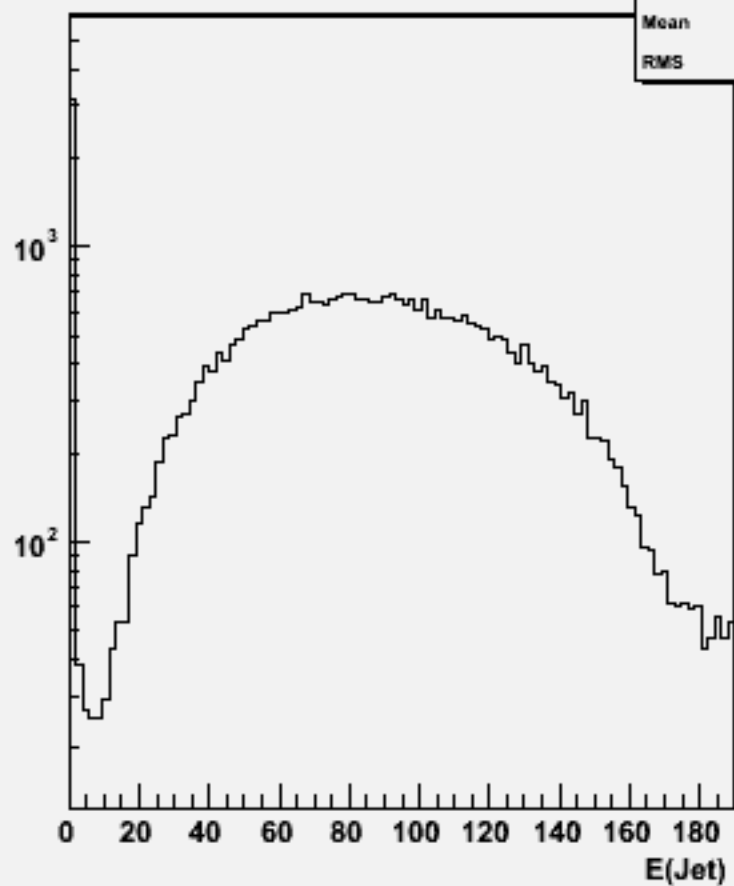
Jet energies(All jets)w102533 e1e1ssbb_o
