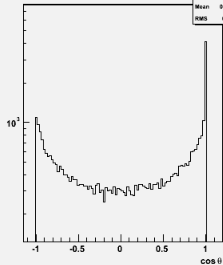
Jet cosθ (All jets)w102533 e1e1ssbb_o
