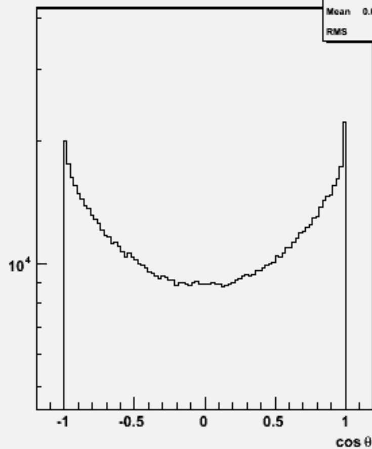
Particle cos \theta : w102533 e1e1ssbb_o
