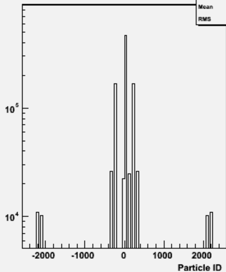
Particle ID : w102533 e1e1ssbb_o
