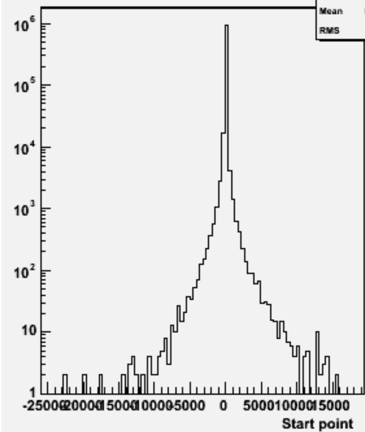
Start point Z : w102533 e1e1ssbb_o
