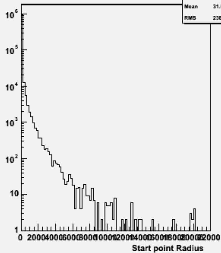
Start point R : w102533 e1e1ssbb_o
