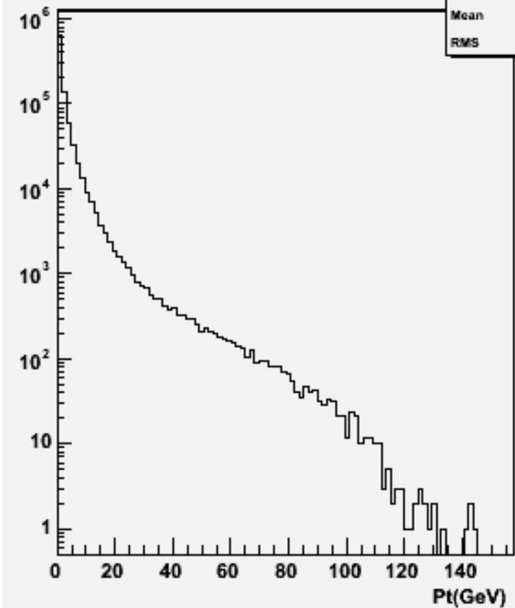
Particle Pt : w102533 e1e1ssbb_o
